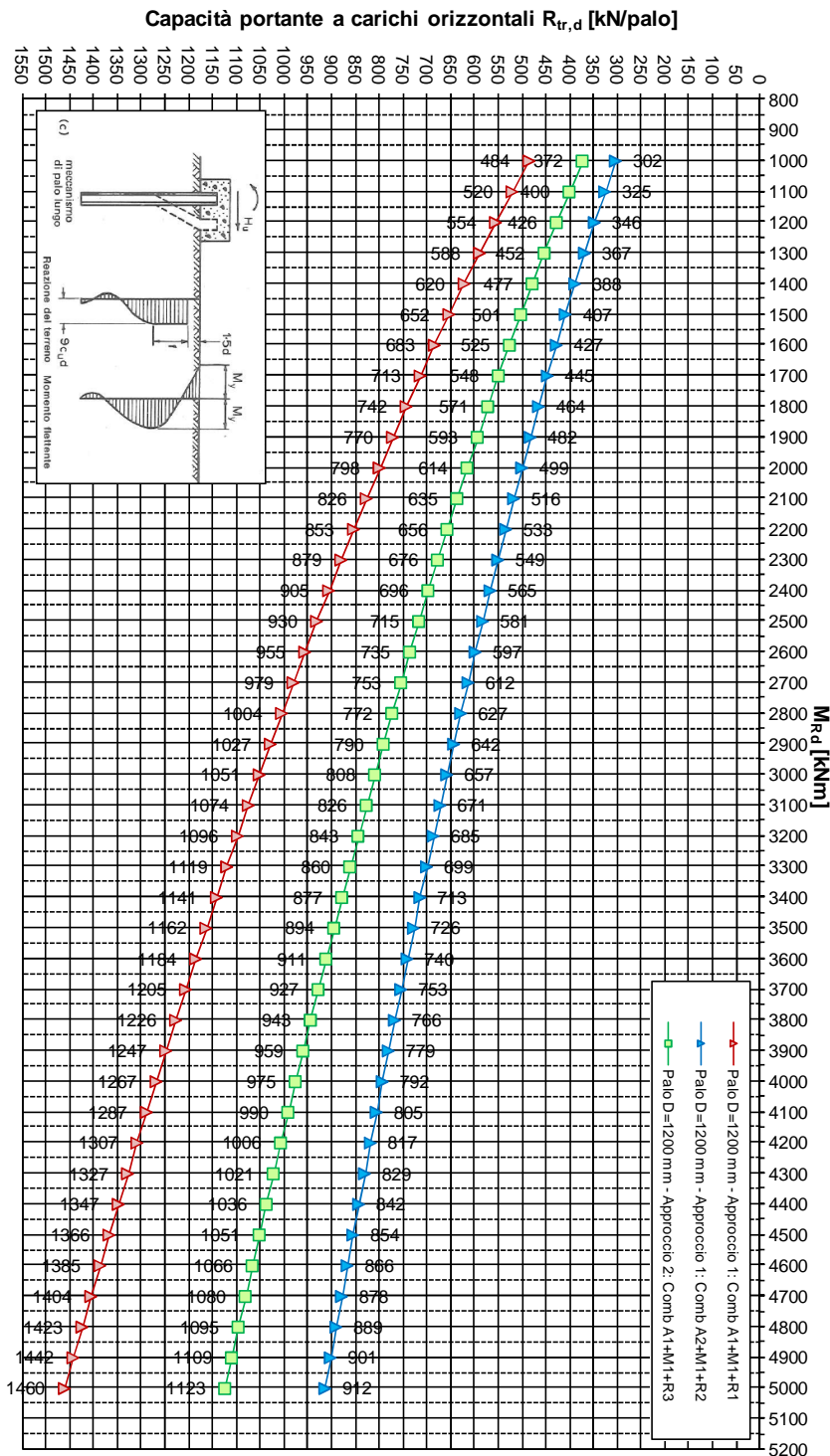
Capacità portante di progetto del singolo palo soggetto a carichi trasversali - R_{tr,d} D = 1200 mm - condizione di incastro in testa Pali di fondazione - Opera ICV04 - ZO F
