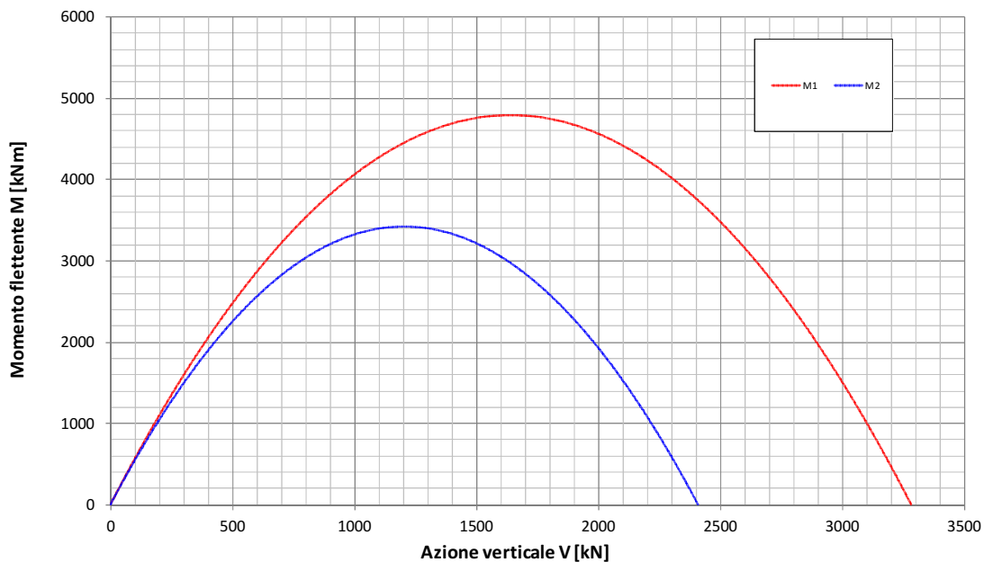
Fondazione B=12.9m - Approfondimento D=0.9m Condizione Sismica Non Drenata Dominio di interazione nel piano V-M ( Gourvenec, 2007 )
