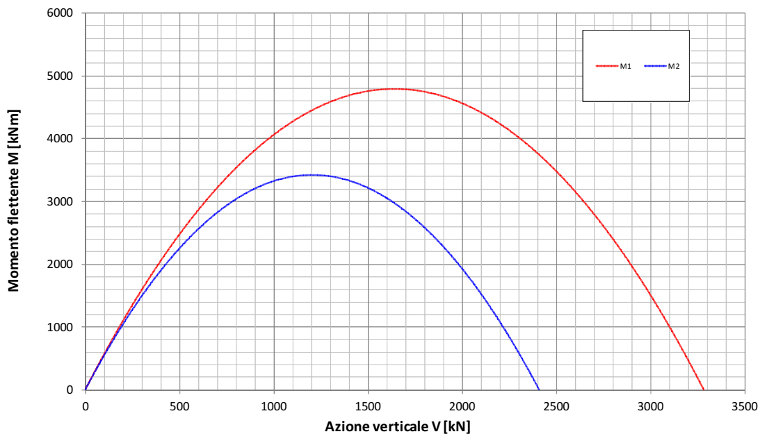
Fondazione B=12.9m - Approfondimento D=0.9m Condizione Statica Non Drenata Dominio di interazione nel piano V-M (Gourvenec, 2007)
