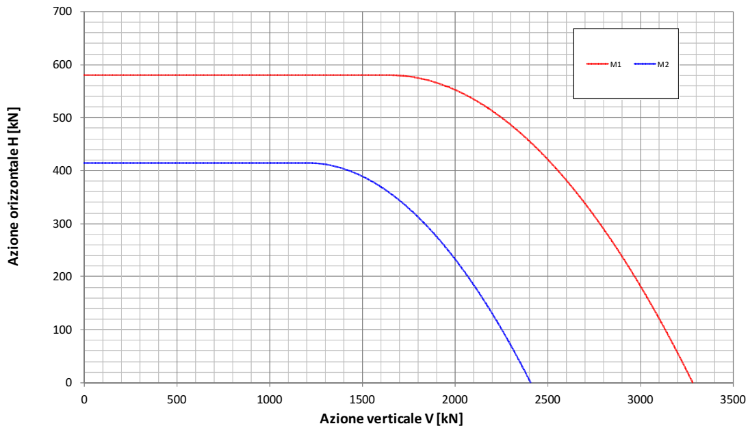
Fondazione B=12.9m - Approfondimento D=0.9m Condizione Sismica Non Drenata Dominio di interazione nel piano V-H ( Gourvenec, 2007 )
