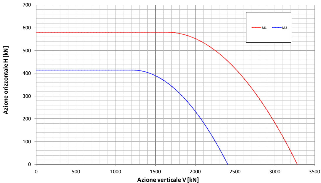
Fondazione B=12.9m - Approfondimento D=0.9m Condizione Statica Non Drenata Dominio di interazione nel piano V-H (Gourvenec, 2007)
