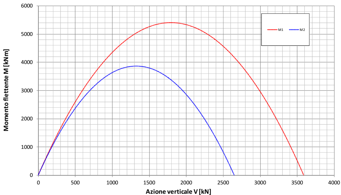
Fondazione B=13.7m - Approfondimento D=1.2m Condizione Sismica Non Drenata Dominio di interazione nel piano V-M ( Gourvenec, 2007 )
