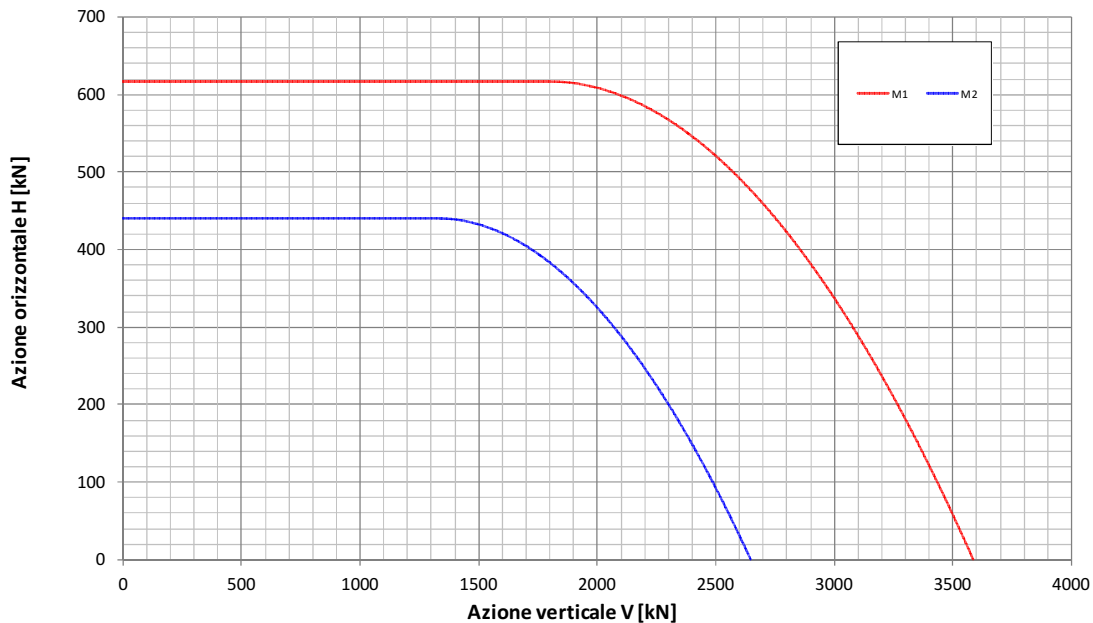
Fondazione B=13.7m - Approfondimento D=1.2m Condizione Sismica Non Drenata Dominio di interazione nel piano V-H ( Gourvenec, 2007 )
