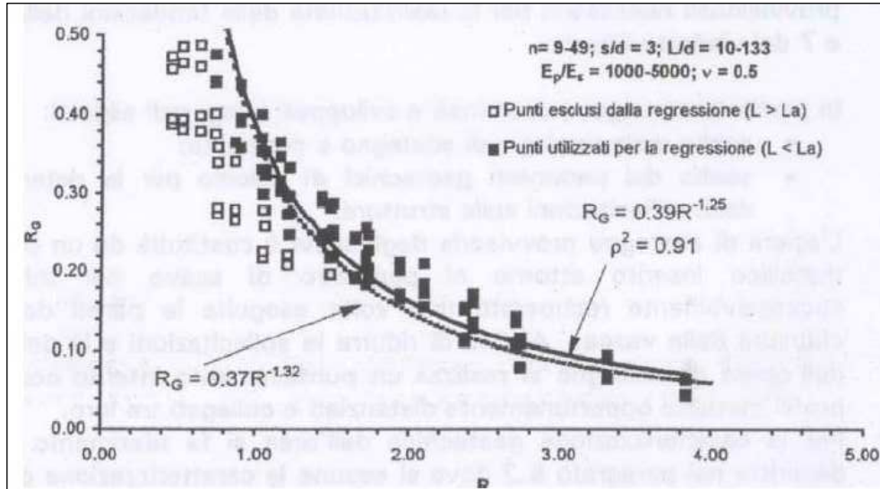
FIGURA 8-1: AMPLIFICAZIONE DEL CEDIMENTO PER EFFETTO GRUPPO
