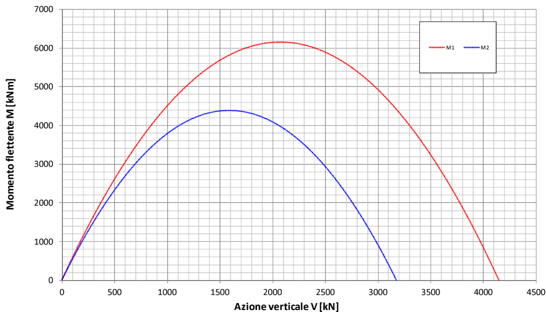
Fondazione B=15.5m - Approfondimento D=2.6m Condizione Statica Non Drenata Dominio di interazione nel piano V-M (Gourvenec, 2007)
