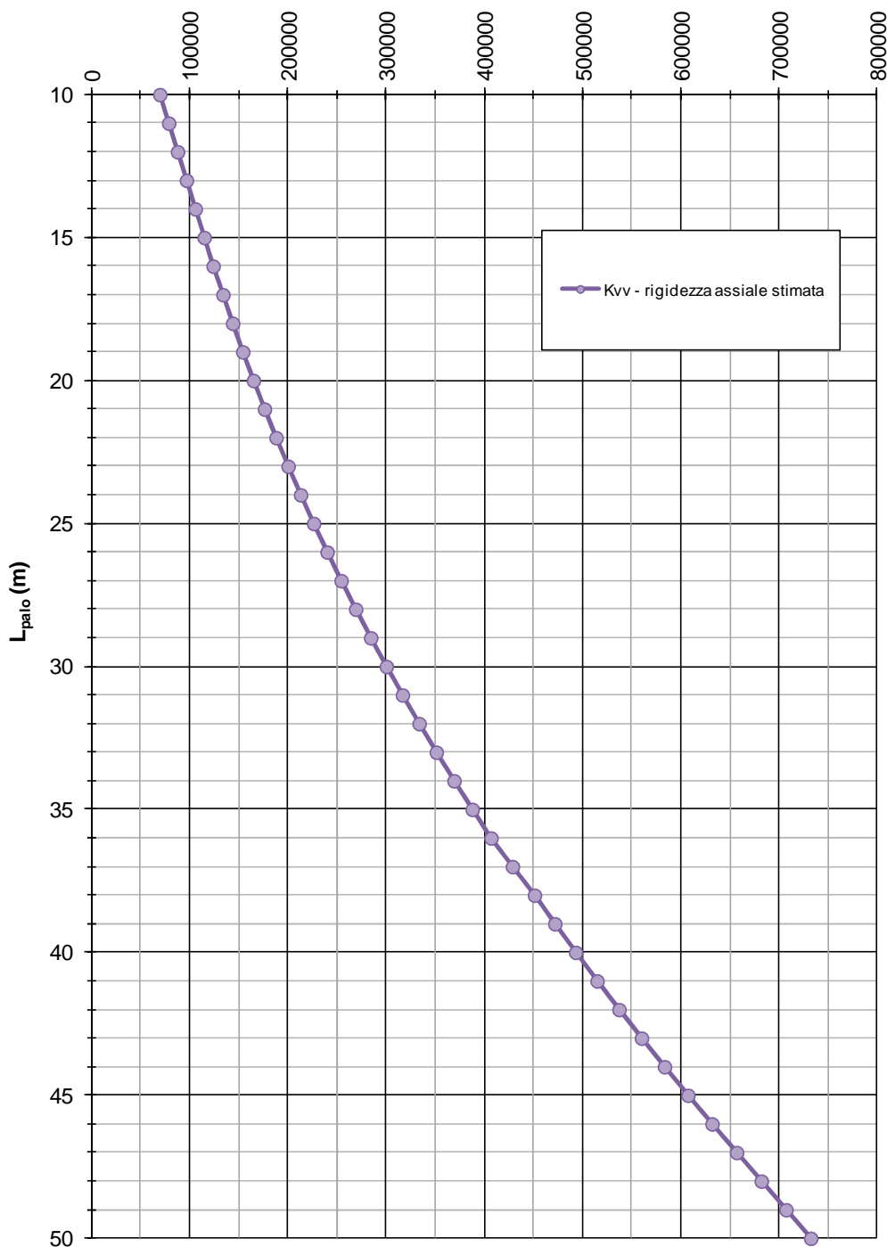
FIGURA 8-3: RIGIDEZZA VERTICALE – PALI TRIVELLATI \phi 800
