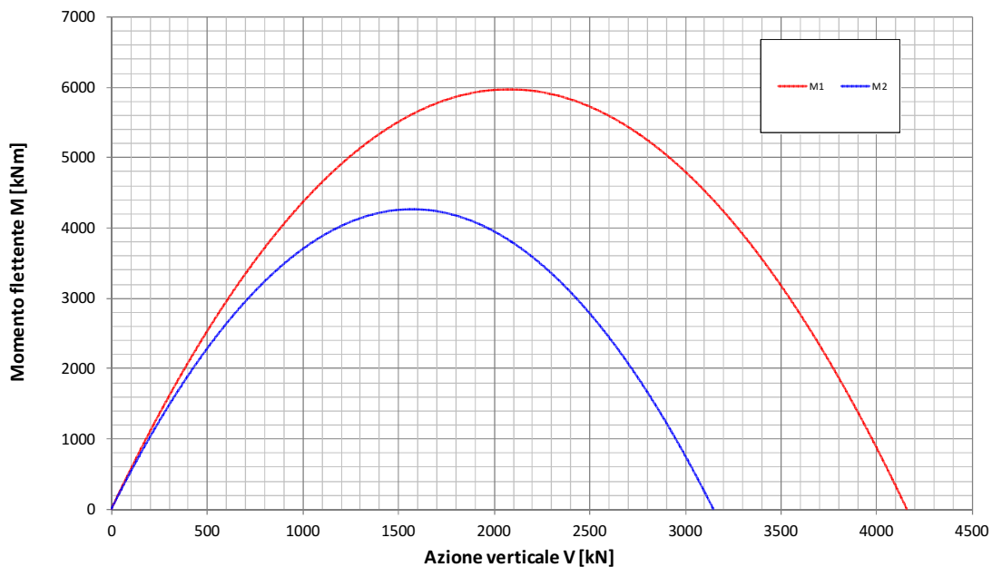
Fondazione B=14.4m - Approfondimento D=2.3m Condizione Statica Non Drenata Dominio di interazione nel piano V-M ( Gourvenec, 2007 )
