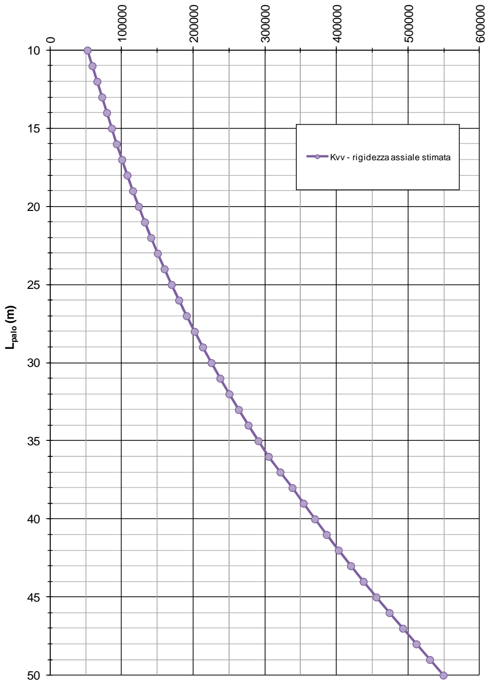
FIGURA 8-2: RIGIDEZZA VERTICALE – PALI TRIVELLATI \phi 600
