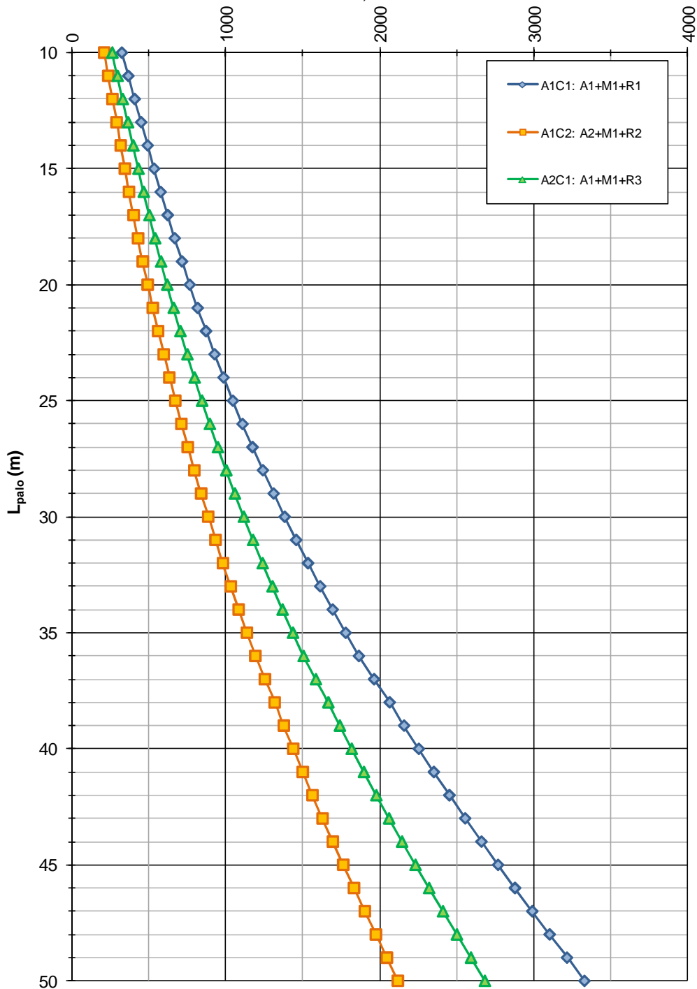
FIGURA 6-2: CAPACITÀ PORTANTE A TRAZIONE – PALI TRIVELLATI \phi 600
