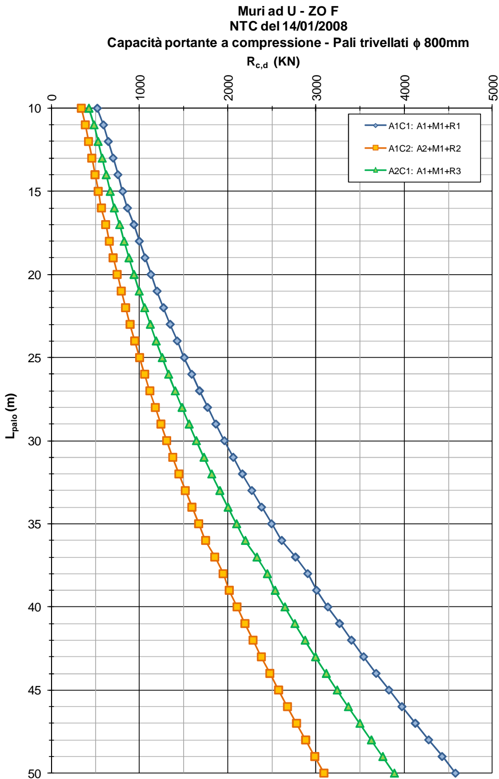
FIGURA 6-3: CAPACITÀ PORTANTE A COMPRESSIONE – PALI TRIVELLATI \phi 800
