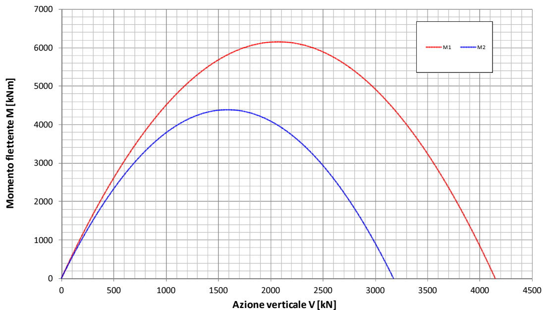
Fondazione B=15.5m - Approfondimento D=2.6m Condizione Sismica Non Drenata Dominio di interazione nel piano V-M (Gourvenec, 2007)
