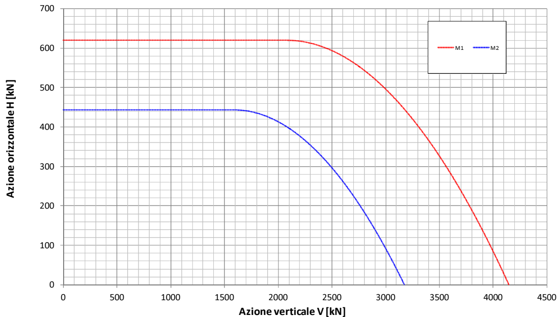
Fondazione B=15.5m - Approfondimento D=2.6m Condizione Sismica Non Drenata Dominio di interazione nel piano V-H (Gourvenec, 2007)
