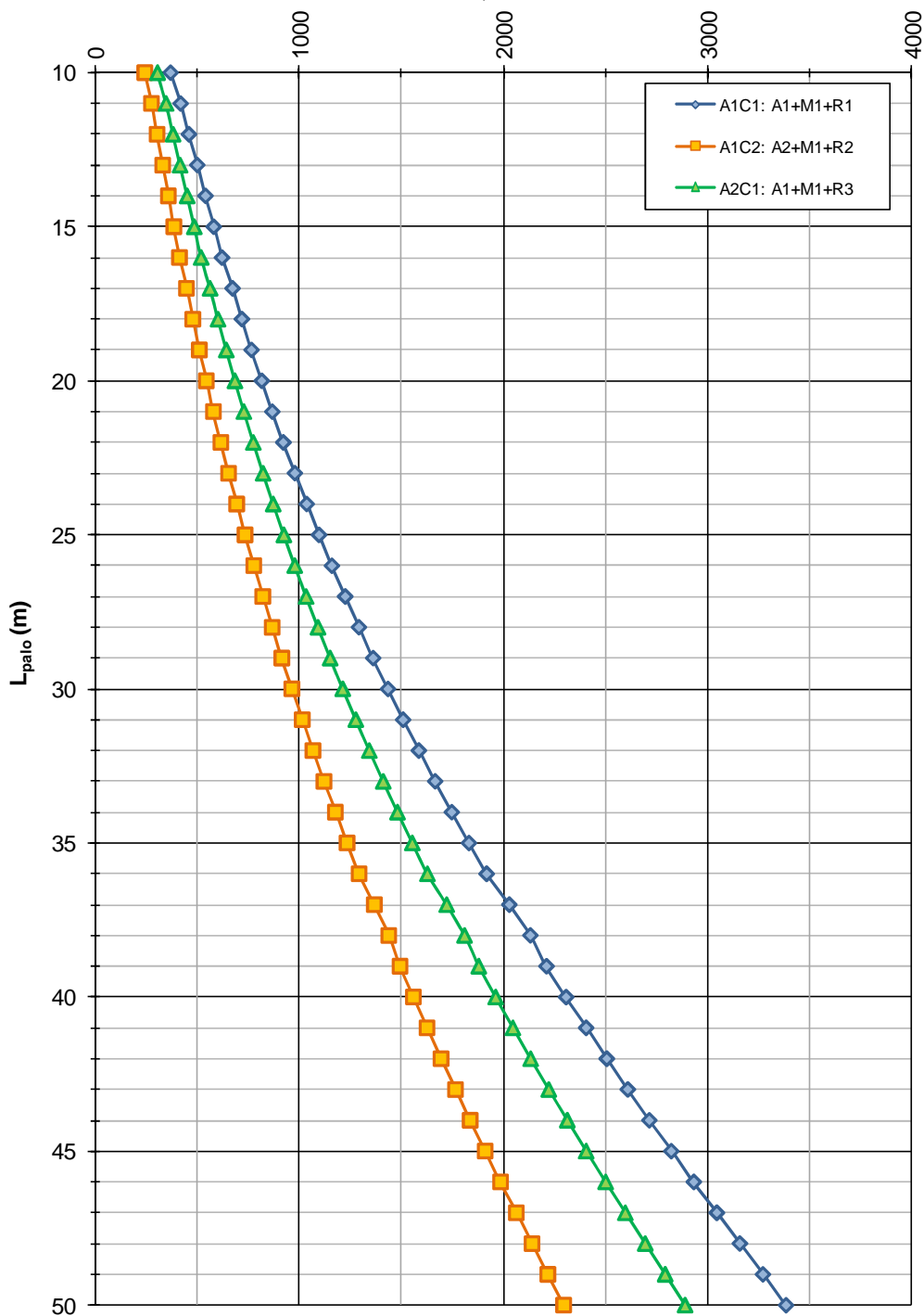
FIGURA 6-1: CAPACITÀ PORTANTE A COMPRESSIONE – PALI TRIVELLATI \phi 600
