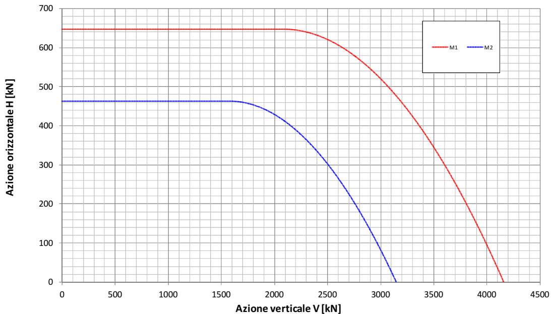
Fondazione B=14.4m - Approfondimento D=2.3m Condizione Statica Non Drenata Dominio di interazione nel piano V-H ( Gourvenec, 2007 )
