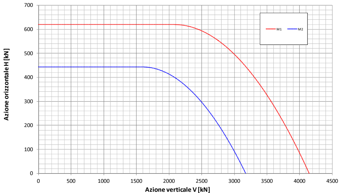
Fondazione B=15.5m - Approfondimento D=2.6m Condizione Statica Non Drenata Dominio di interazione nel piano V-H (Gourvenec, 2007)
