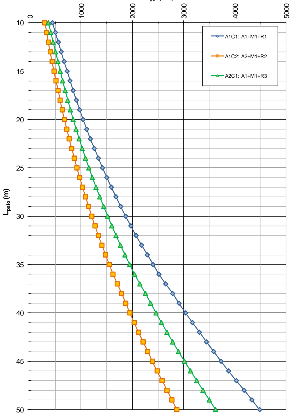
FIGURA 6-4: CAPACITÀ PORTANTE A TRAZIONE – PALI TRIVELLATI \phi 800
