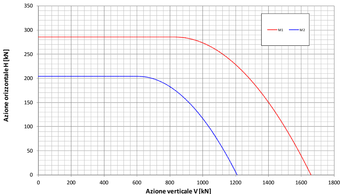
Fondazione B=5.2m - Approfondimento D=0.9m Condizione Statica Non Drenata Dominio di interazione nel piano V-H (Gourvenec, 2007)
