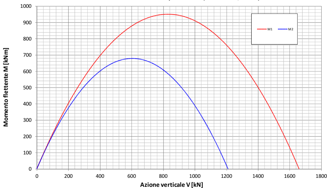
Fondazione B=5.2m - Approfondimento D=0.9m Condizione Statica Non Drenata Dominio di interazione nel piano V-M (Gourvenec, 2007)
