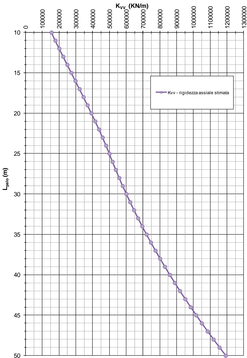
FIGURA 10-2: RIGIDEZZA VERTICALE – PALI TRIVELLATI \phi 1000 (ZONA OMOGENEA 3)
