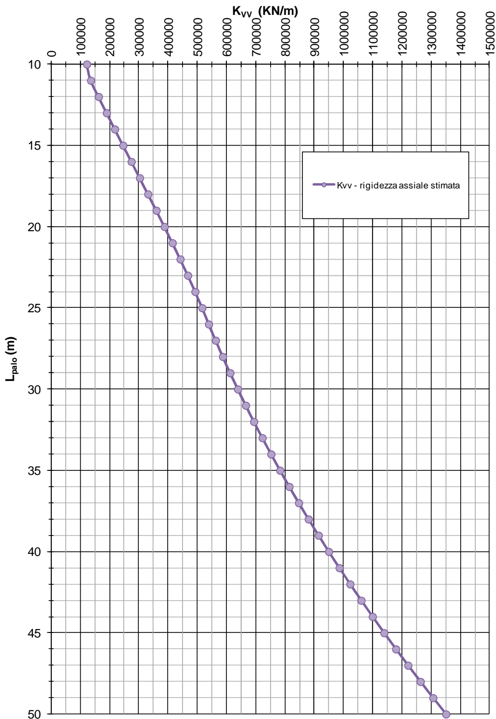
FIGURA 10-5: RIGIDEZZA VERTICALE – PALI TRIVELLATI \phi 1200 (ZONA OMOGENEA 4)
