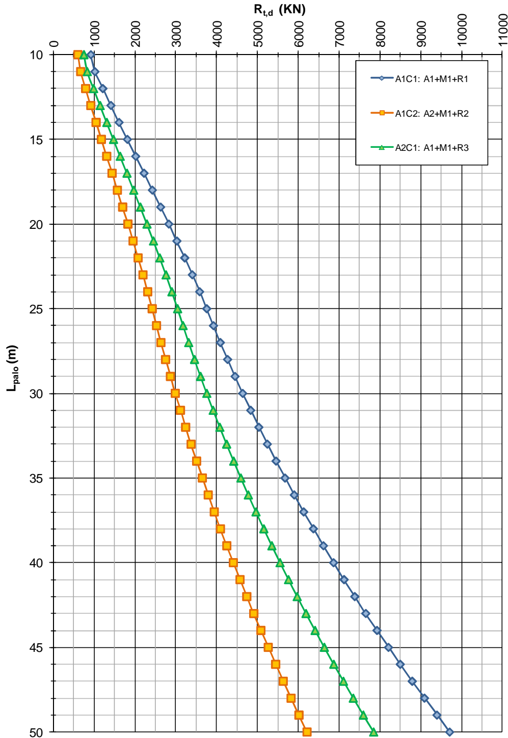
FIGURA 4-8: CAPACITÀ PORTANTE A TRAZIONE – PALI TRIVELLATI \phi 1200 (ZONA OMOGENEA 4)
