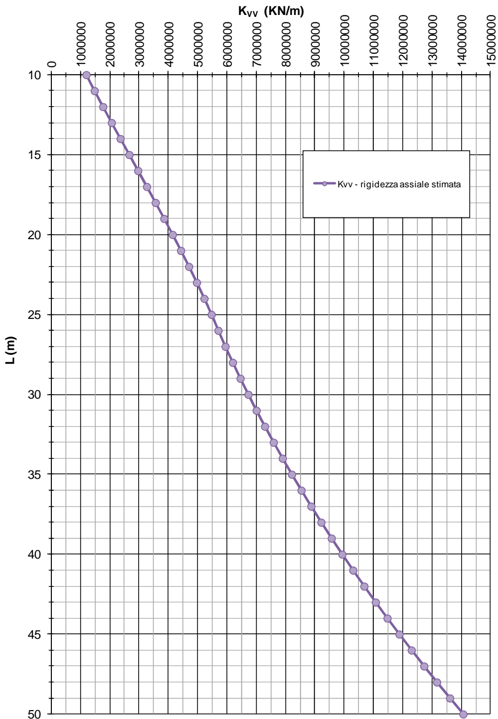
FIGURA 10-8: RIGIDEZZA VERTICALE – POZZO DI DIAFRAMMI 12.5M X 7M (ZONA OMOGENEA 3)
