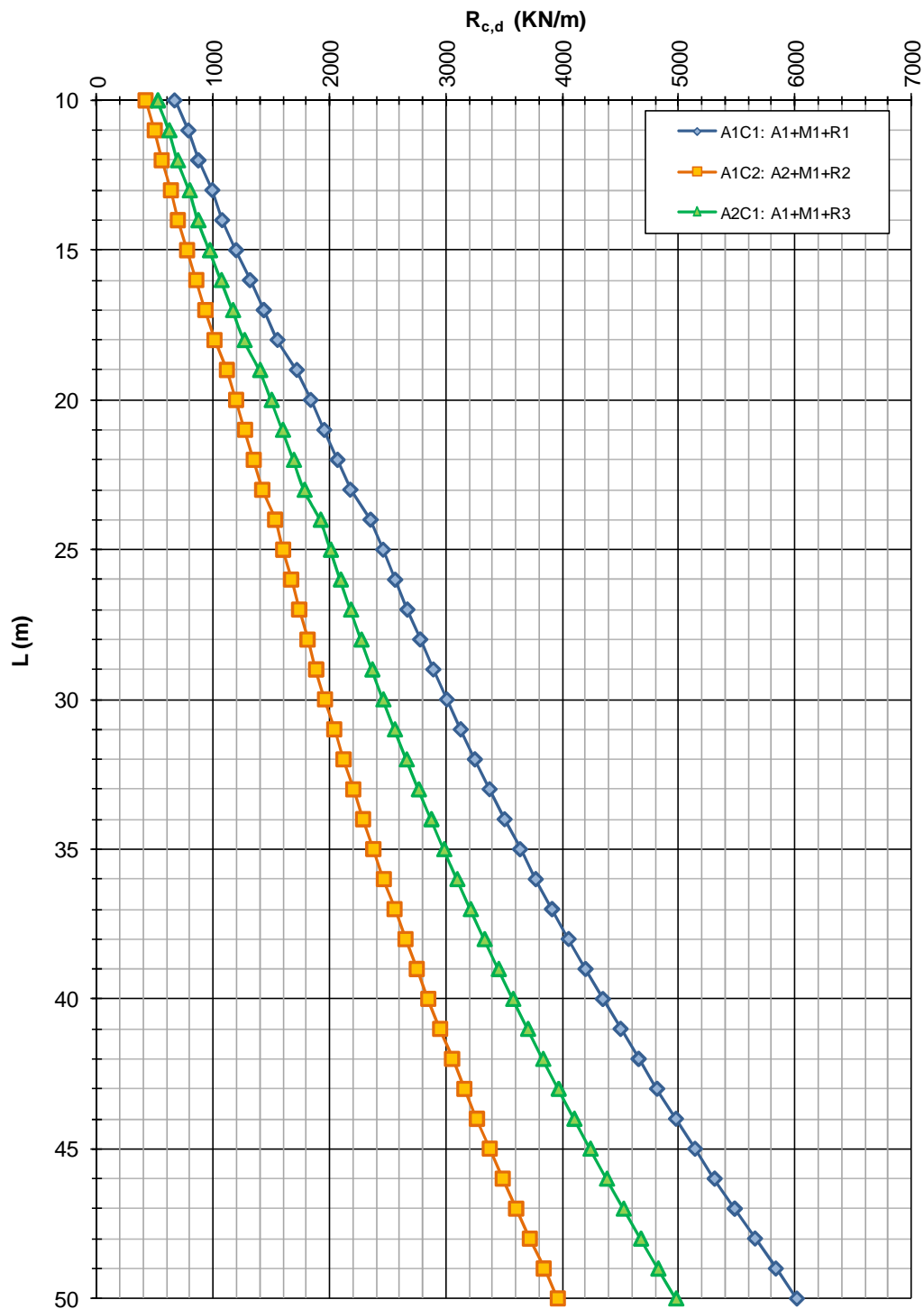
FIGURA 4-9: CAPACITÀ PORTANTE A COMPRESSIONE – DIAFRAMMI S 1000 (ZONA OMOGENEA 3)
