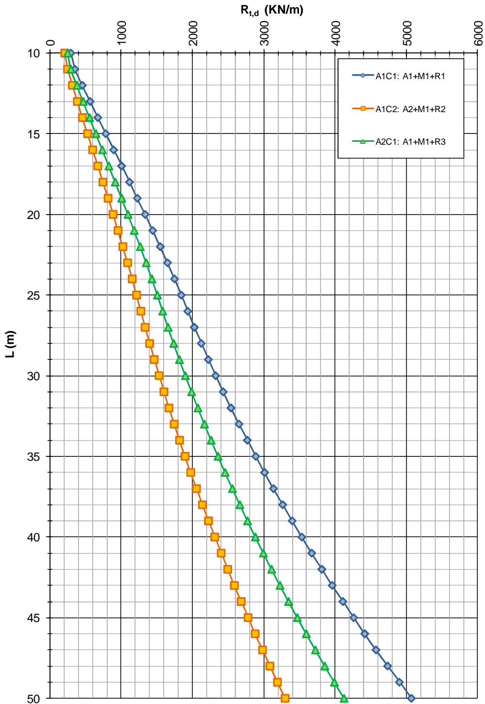
FIGURA 4-12: CAPACITÀ PORTANTE A TRAZIONE – DIAFRAMMI S 1000 (ZONA OMOGENEA 4)
