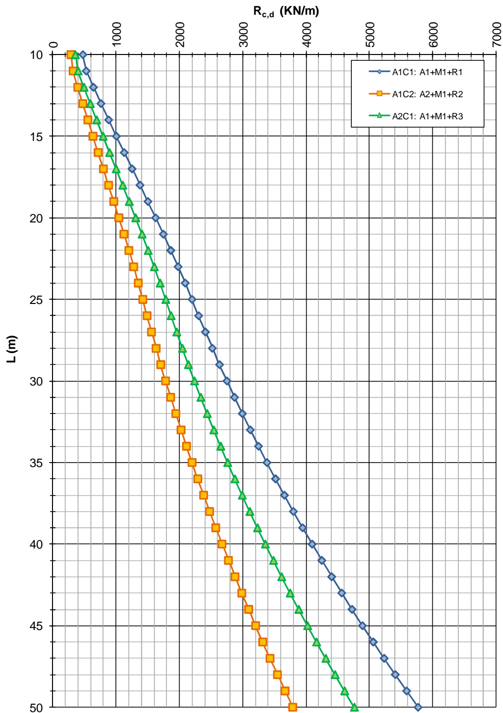
FIGURA 4-11: CAPACITÀ PORTANTE A COMPRESSIONE – DIAFRAMMI S 1000 (ZONA OMOGENEA 4)
