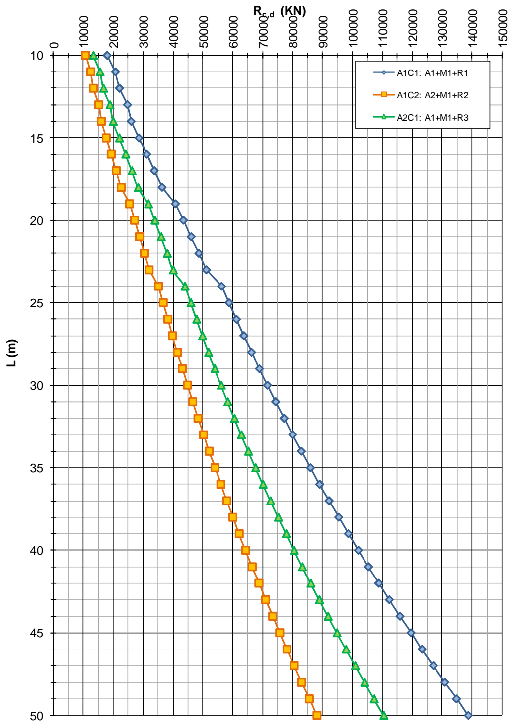
FIGURA 4-13: CAPACITÀ PORTANTE A COMPRESSIONE – POZZO DI DIAFRAMMI 12.5M X 7M (ZONA OMOGENEA 3)
