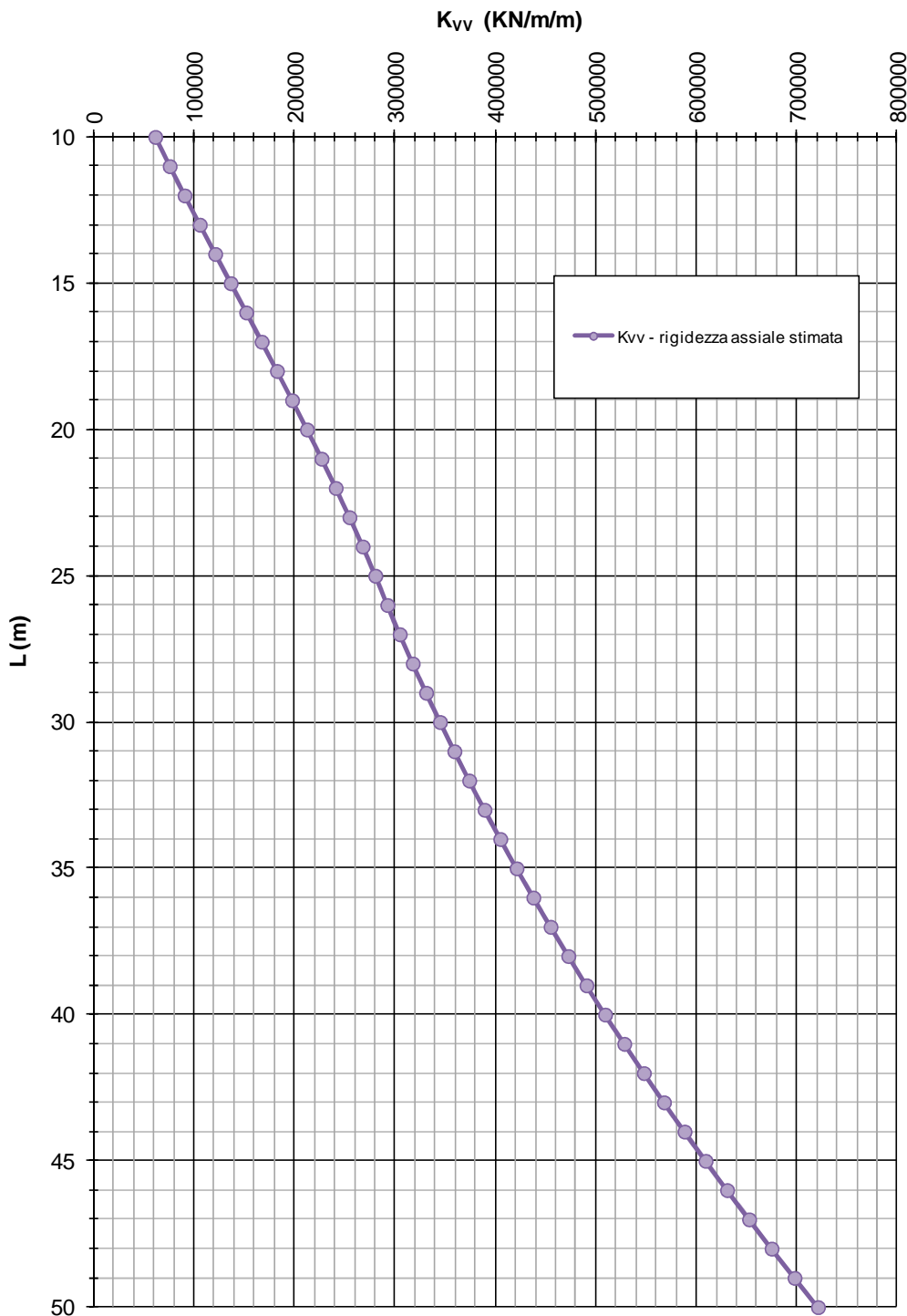
FIGURA 10-6: RIGIDEZZA VERTICALE – DIAFRAMMI S 1000 (ZONA OMOGENEA 3)
