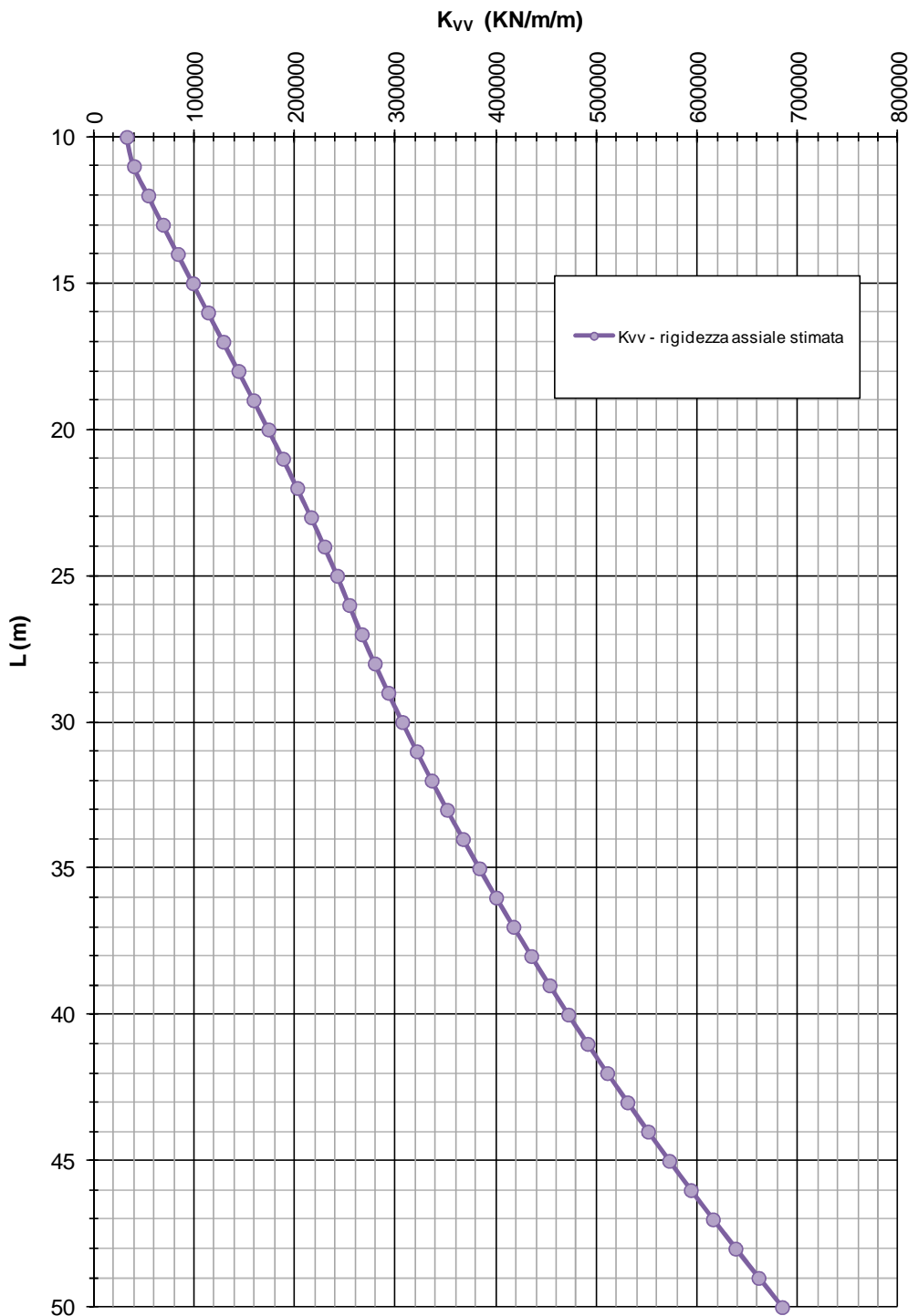
FIGURA 10-7: RIGIDEZZA VERTICALE – DIAFRAMMI S 1000 (ZONA OMOGENEA 4)
