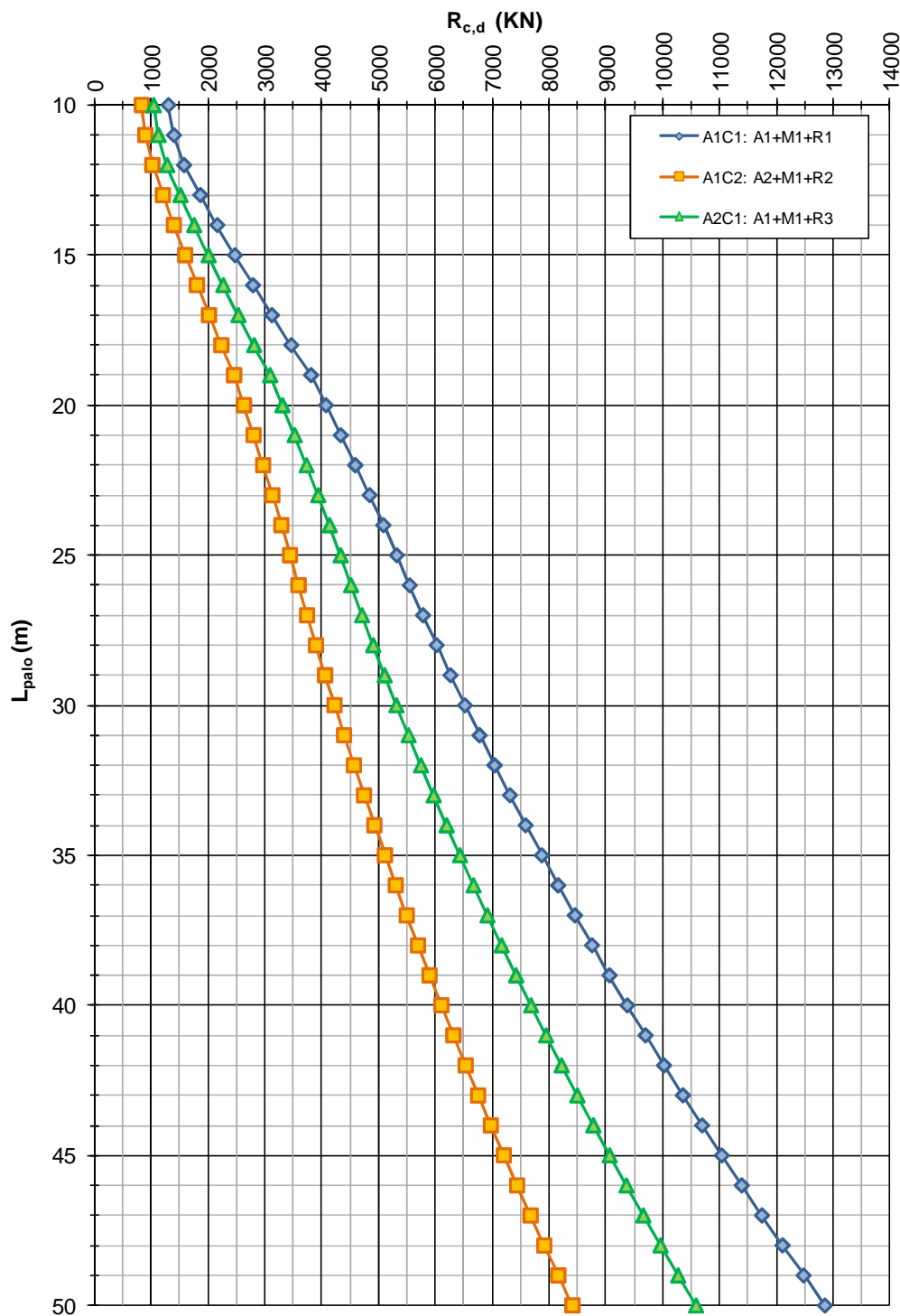
FIGURA 4-7: CAPACITÀ PORTANTE A COMPRESSIONE – PALI TRIVELLATI \phi 1200 (ZONA OMOGENEA 4)
