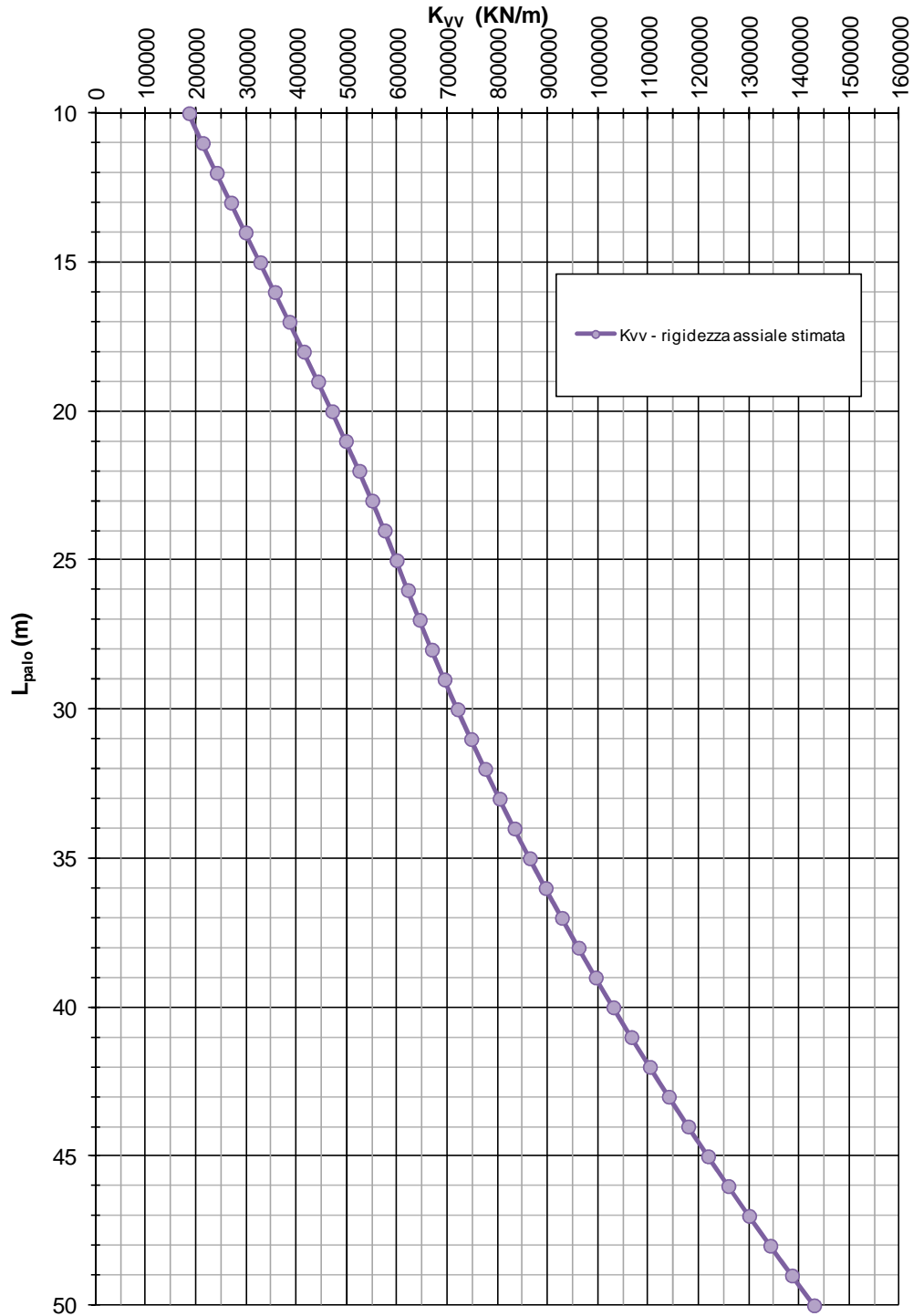
FIGURA 10-3: RIGIDEZZA VERTICALE – PALI TRIVELLATI \phi 1200 (ZONA OMOGENEA 3)
