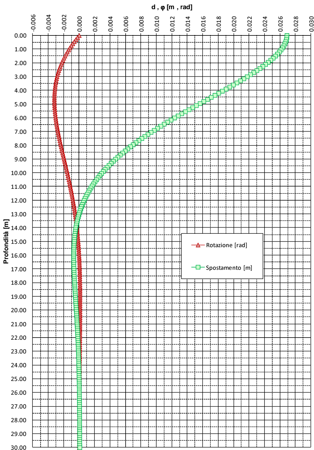
FIGURA 6-8: SPOSTAMENTI E ROTAZIONI – PALI TRIVELLATI \phi 1200 (ZONA OMOGENEA 4)
