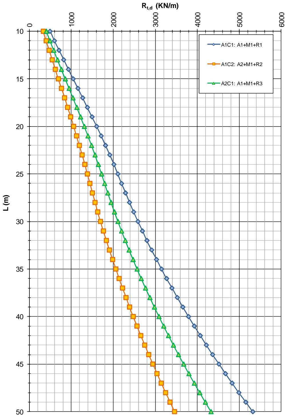
FIGURA 4-10: CAPACITÀ PORTANTE A TRAZIONE – DIAFRAMMI 1000 (ZONA OMOGENEA 3)
