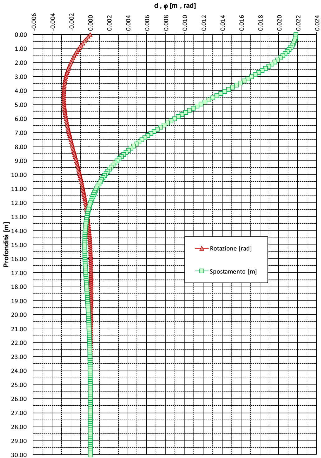
FIGURA 6-4: SPOSTAMENTI E ROTAZIONI – PALI TRIVELLATI φ 1200 (ZONA OMOGENEA 3)
