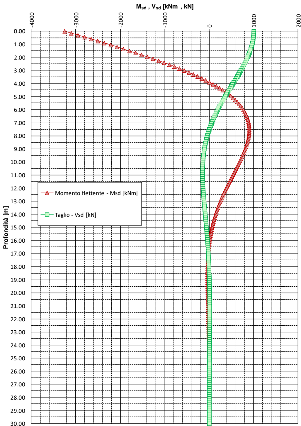
FIGURA 6-5: ANDAMENTO DELLE SOLLECITAZIONI FLETTENTE E TAGLIANTE – PALI TRIVELLATI \phi 1000 (ZONA OMOGENEA 4)
