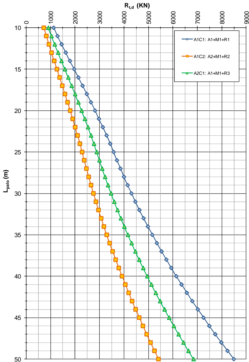
FIGURA 4-2: CAPACITÀ PORTANTE A TRAZIONE – PALI TRIVELLATI \phi 1000 (ZONA OMOGENEA 3)
