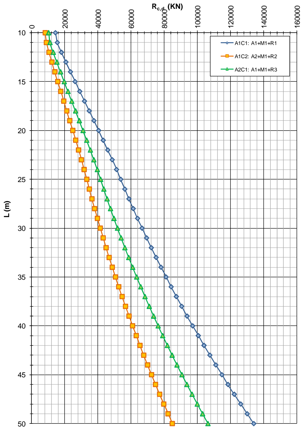
FIGURA 4-15: CAPACITÀ PORTANTE A COMPRESSIONE – POZZO DI DIAFRAMMI 12.5M X 7M (ZONA OMOGENEA 4)
