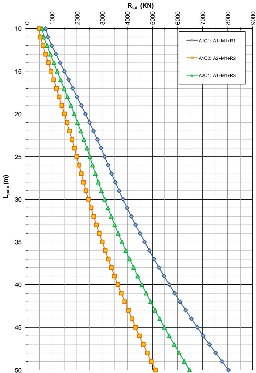
FIGURA 4-6: CAPACITÀ PORTANTE A TRAZIONE – PALI TRIVELLATI \phi 1000 (ZONA OMOGENEA 4)
