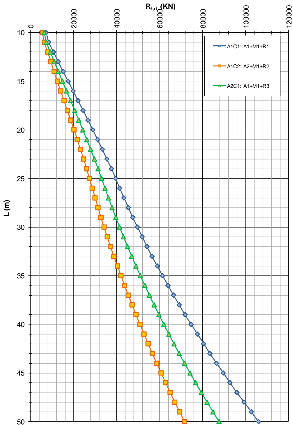
FIGURA 4-16: CAPACITÀ PORTANTE A TRAZIONE – POZZO DI DIAFRAMMI 12.5M X 7M (ZONA OMOGENEA 4)
