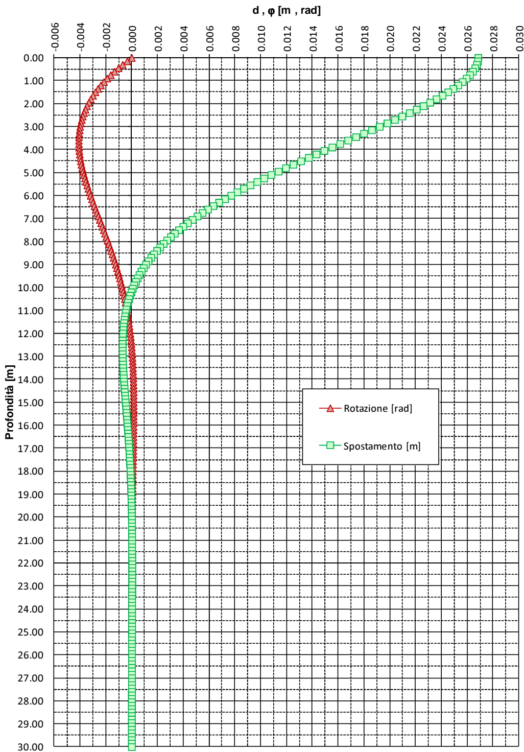
FIGURA 6-2: SPOSTAMENTI E ROTAZIONI – PALI TRIVELLATI \phi 1000 (ZONA OMOGENEA 3)
