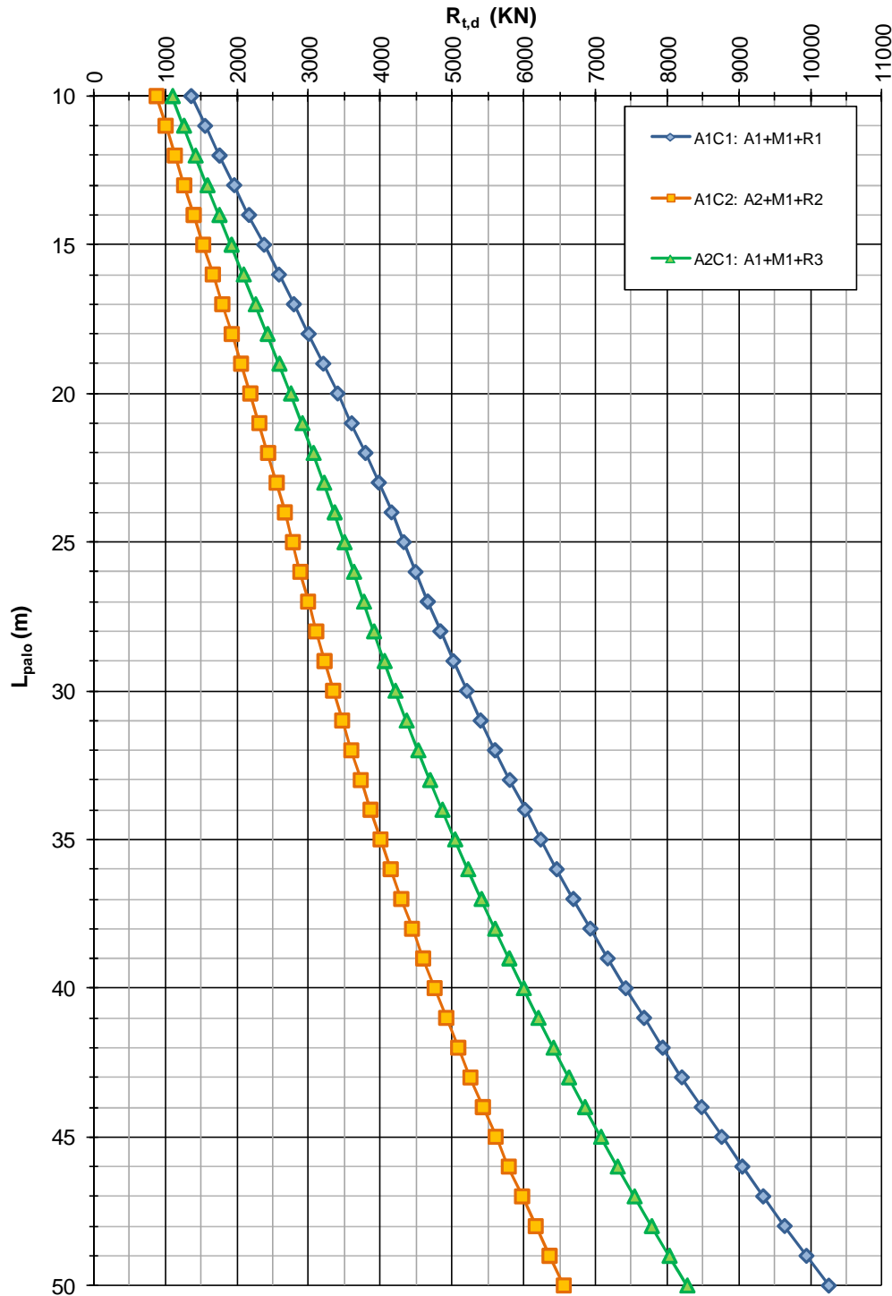
FIGURA 4-4: CAPACITÀ PORTANTE A TRAZIONE – PALI TRIVELLATI \phi 1200 (ZONA OMOGENEA 3)
