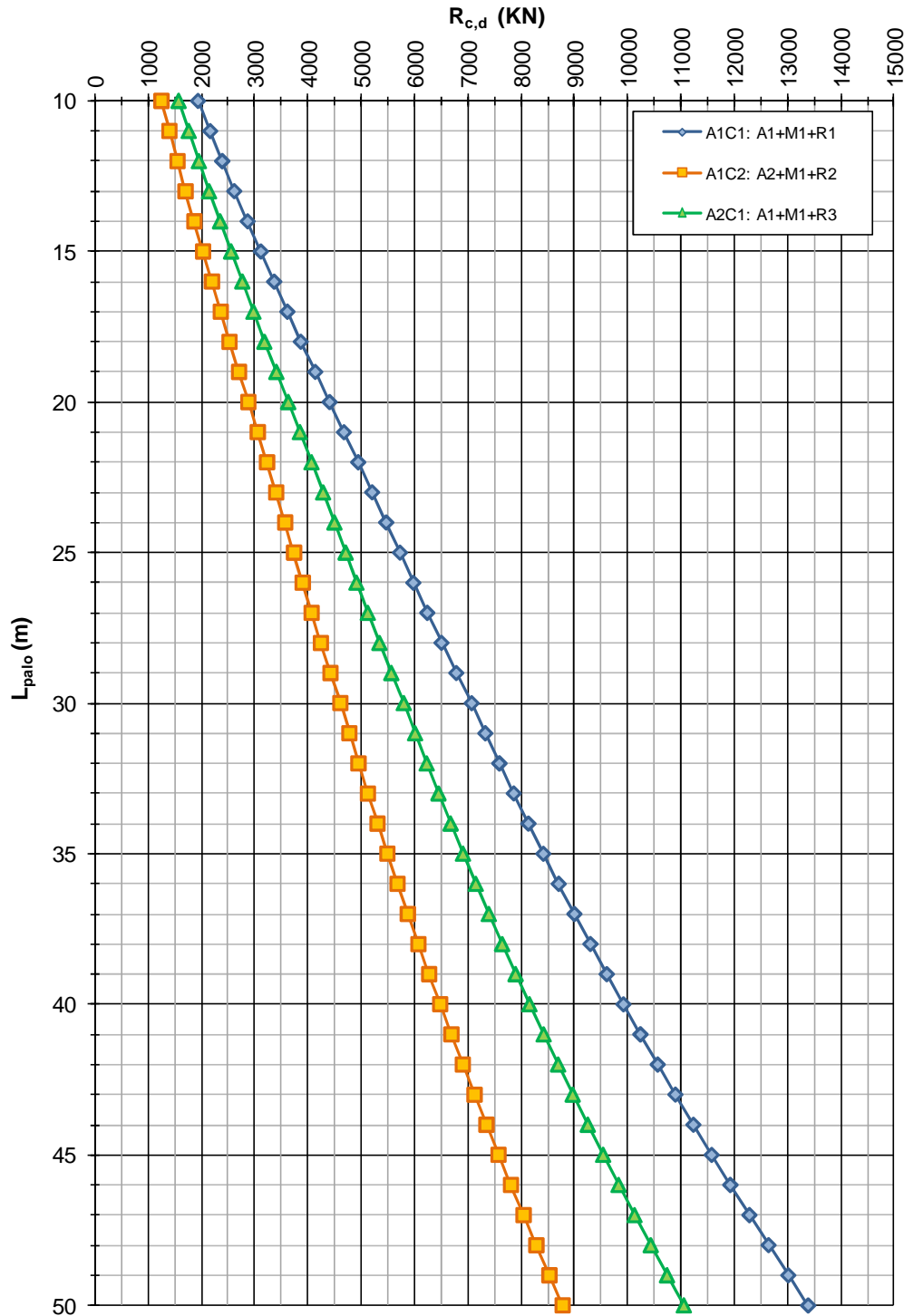
FIGURA 4-3: CAPACITÀ PORTANTE A COMPRESSIONE – PALI TRIVELLATI \phi 1200 (ZONA OMOGENEA 3)
