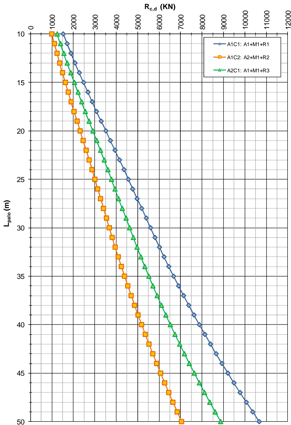
FIGURA 4-1: CAPACITÀ PORTANTE A COMPRESSIONE – PALI TRIVELLATI \phi 1000 (ZONA OMOGENEA 3)
