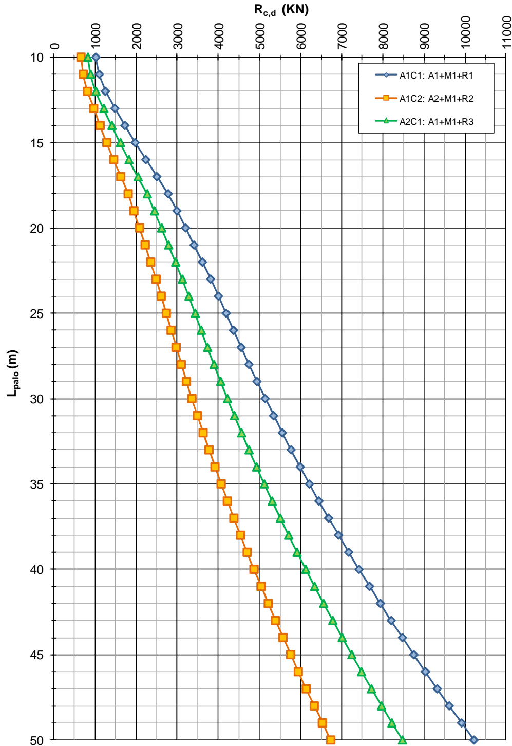
FIGURA 4-5: CAPACITÀ PORTANTE A COMPRESSIONE – PALI TRIVELLATI \phi 1000 (ZONA OMOGENEA 4)
