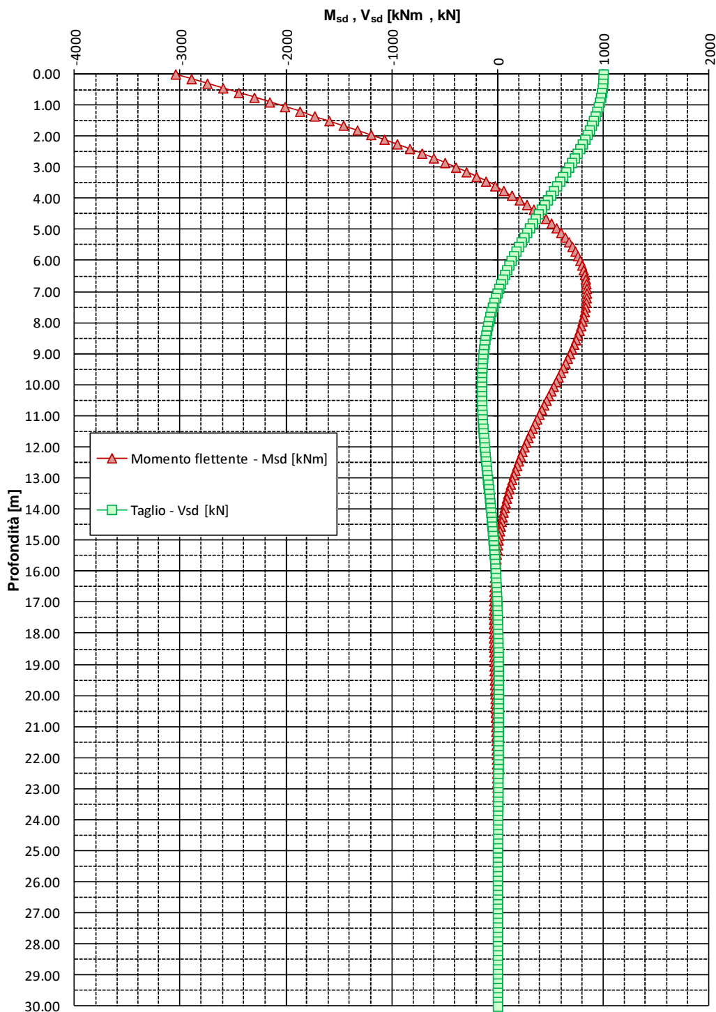
FIGURA 6-1: ANDAMENTO DELLE SOLLECITAZIONI FLETTENTE E TAGLIANTE – PALI TRIVELLATI \phi 1000 (ZONA OMOGENEA 3)
