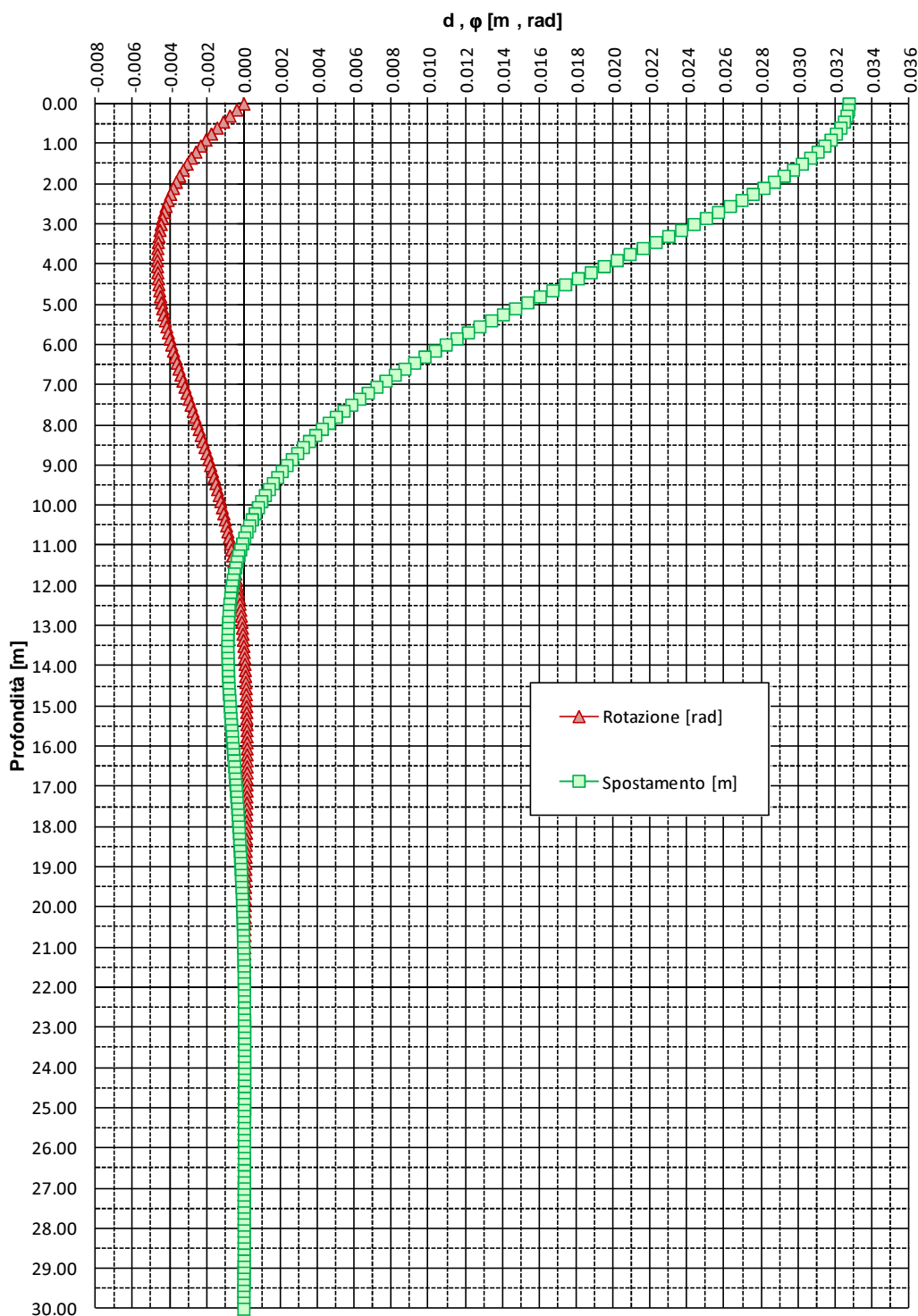
FIGURA 6-6: SPOSTAMENTI E ROTAZIONI – PALI TRIVELLATI \phi 1000 (ZONA OMOGENEA 4)
