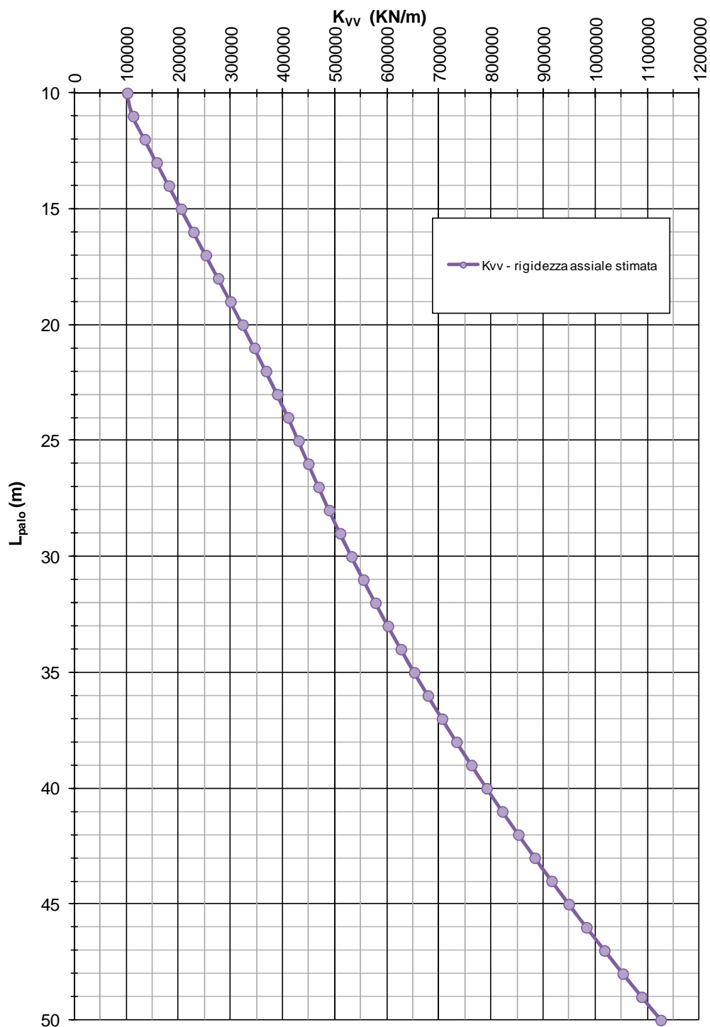
FIGURA 10-4: RIGIDEZZA VERTICALE – PALI TRIVELLATI \phi 1000 (ZONA OMOGENEA 4)
