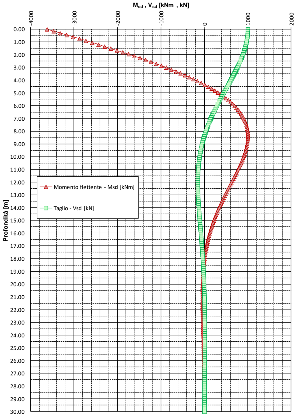
FIGURA 6-3: ANDAMENTO DELLE SOLLECITAZIONI FLETTENTE E TAGLIANTE – PALI TRIVELLATI \phi 1200 (ZONA OMOGENEA 3)
