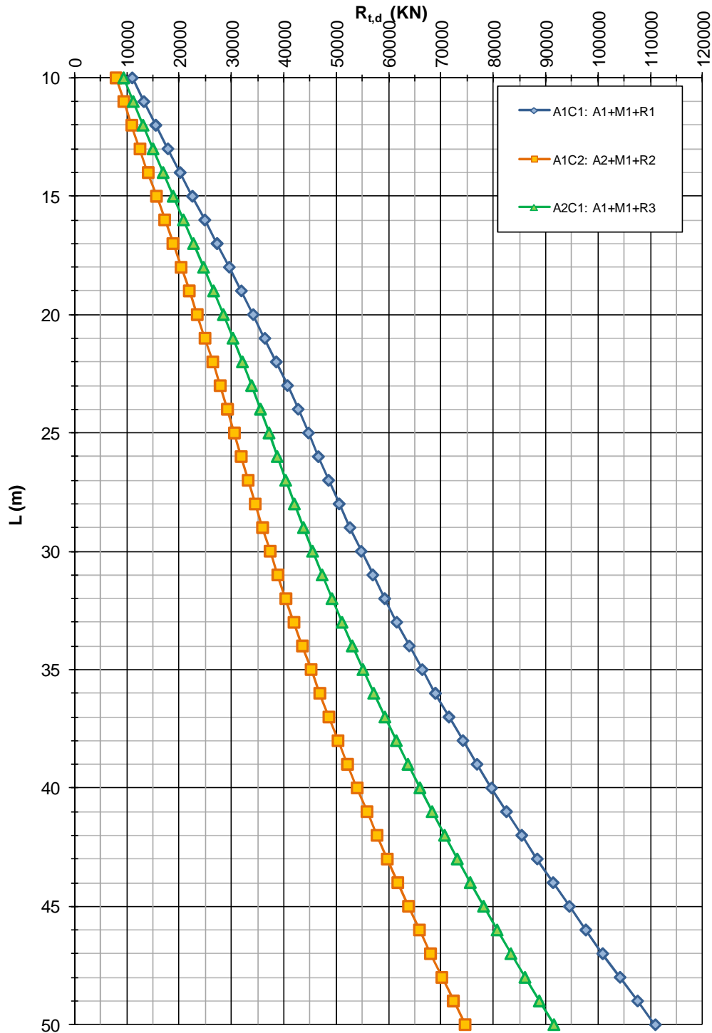
FIGURA 4-14: CAPACITÀ PORTANTE A TRAZIONE – POZZO DI DIAFRAMMI 12.5M X 7M (ZONA OMOGENEA 3)
