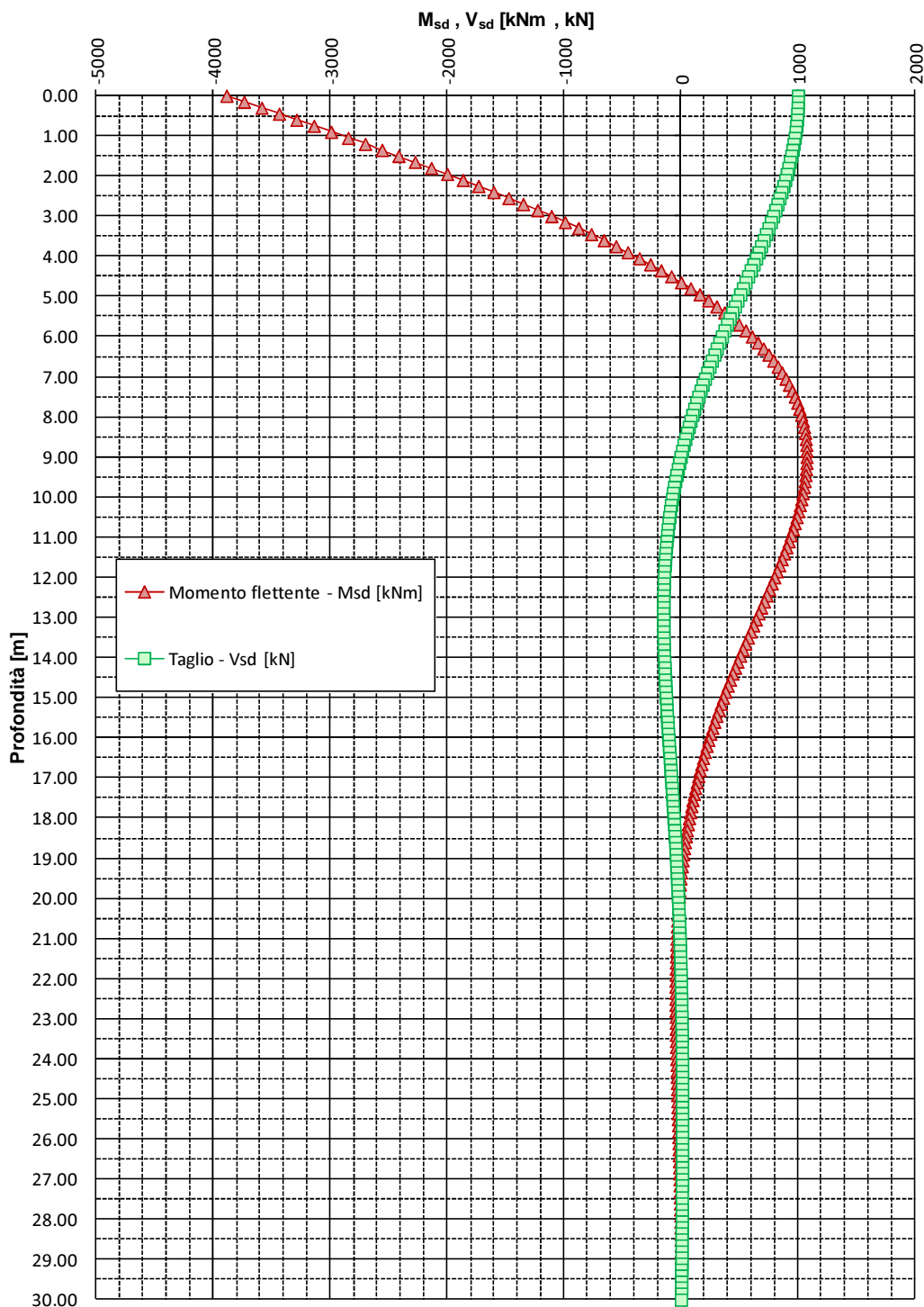
FIGURA 6-7: ANDAMENTO DELLE SOLLECITAZIONI FLETTENTE E TAGLIANTE – PALI TRIVELLATI \phi 1200 (ZONA OMOGENEA 4)
