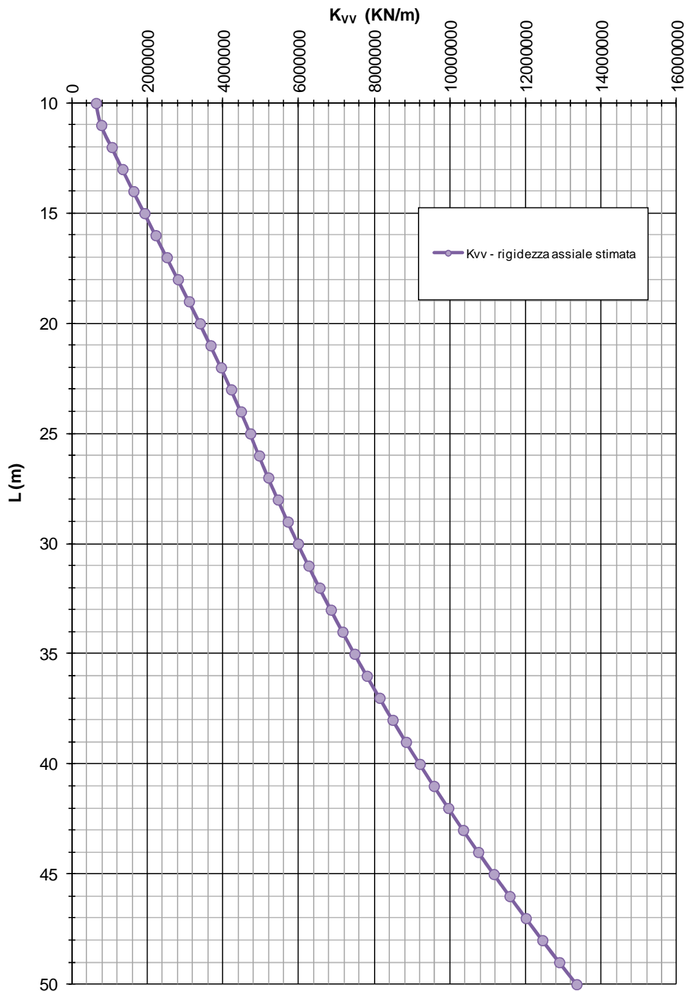
FIGURA 10-9: RIGIDEZZA VERTICALE – POZZO DI DIAFRAMMI 12.5M X 7M (ZONA OMOGENEA 4)
