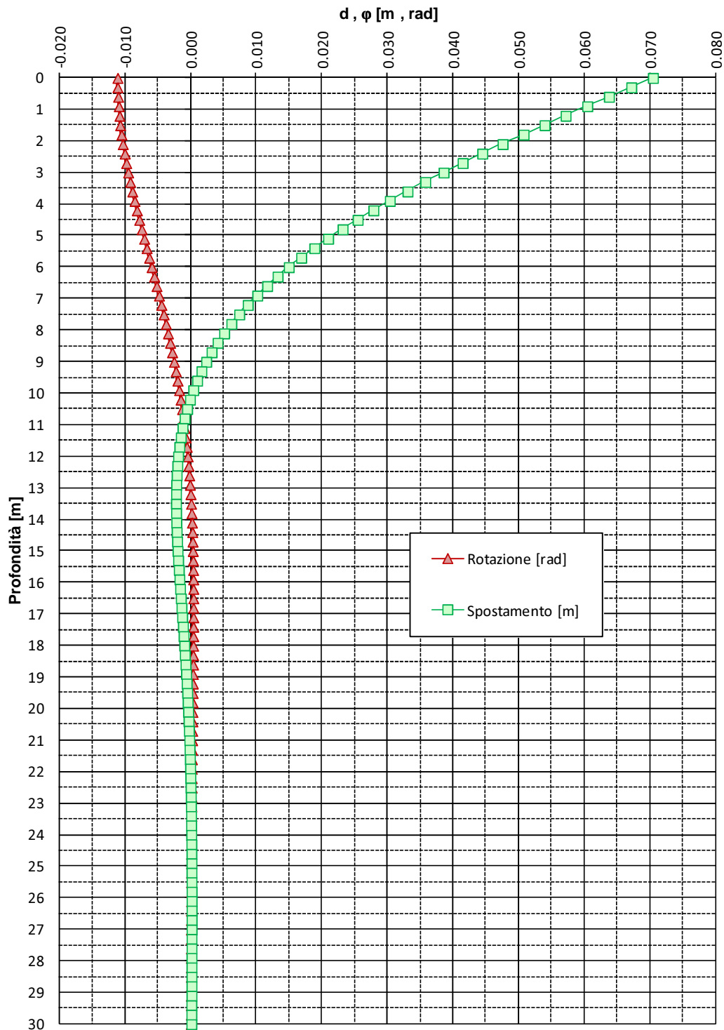
FIGURA 6-6: SPOSTAMENTI E ROTAZIONI (TAGLIO IN TESTA) – PALI TRIVELLATI \phi 1200
