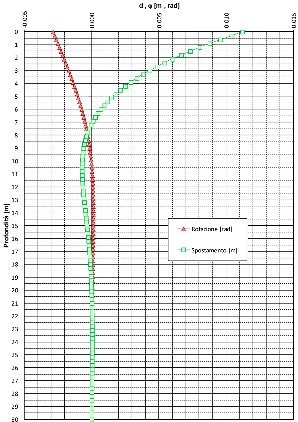
FIGURA 6-8: SPOSTAMENTI E ROTAZIONI (MOMENTO IN TESTA) – PALI TRIVELLATI φ 1200
