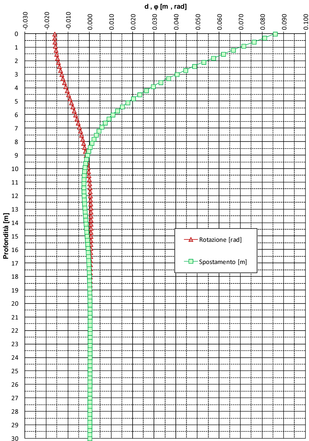
FIGURA 6-2: SPOSTAMENTI E ROTAZIONI (TAGLIO IN TESTA) – PALI TRIVELLATI φ 1000
