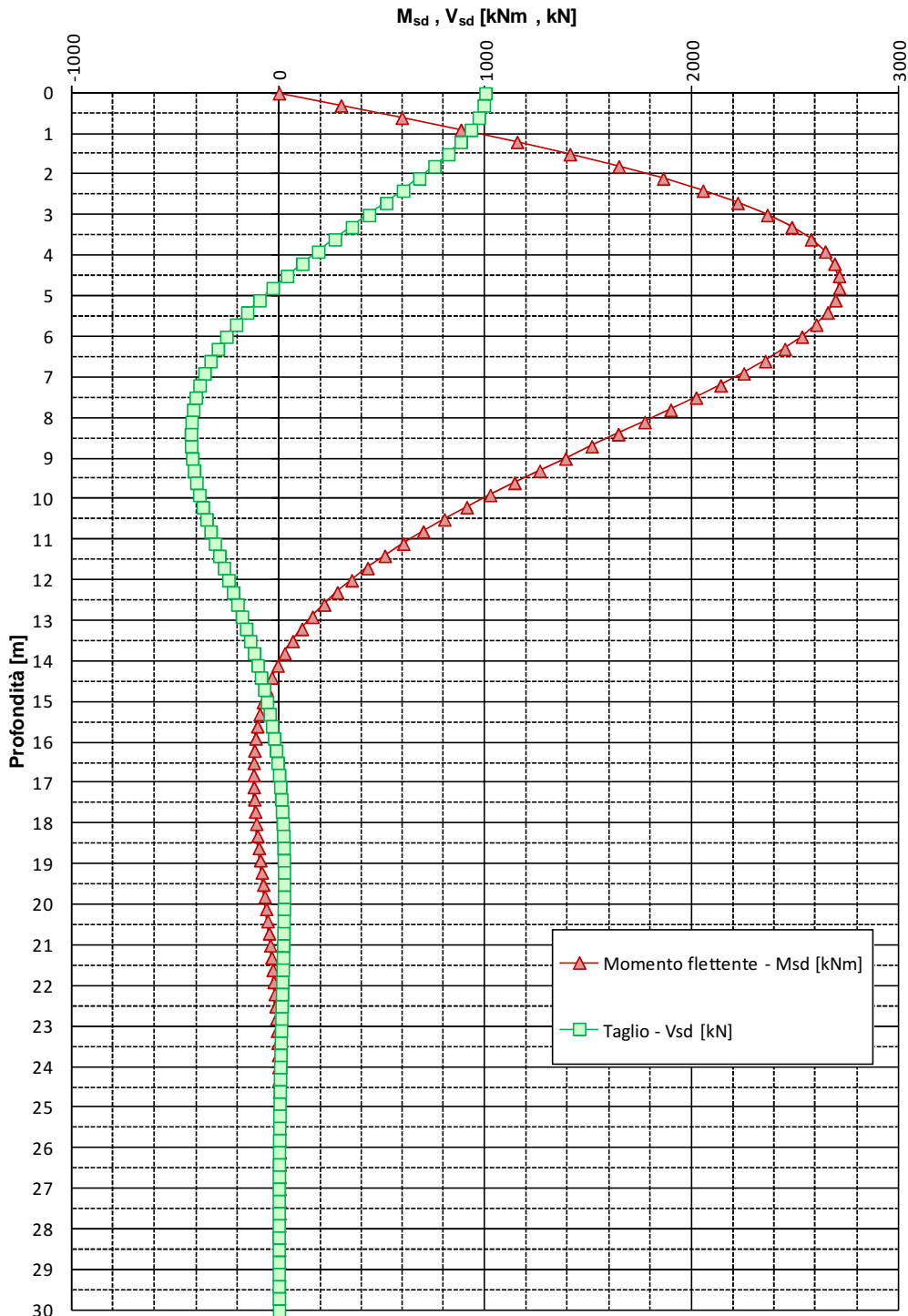
FIGURA 6-1: ANDAMENTO DELLE SOLLECITAZIONI FLETTENTE E TAGLIANTE (TAGLIO IN TESTA) – PALI TRIVELLATI \phi 1000
