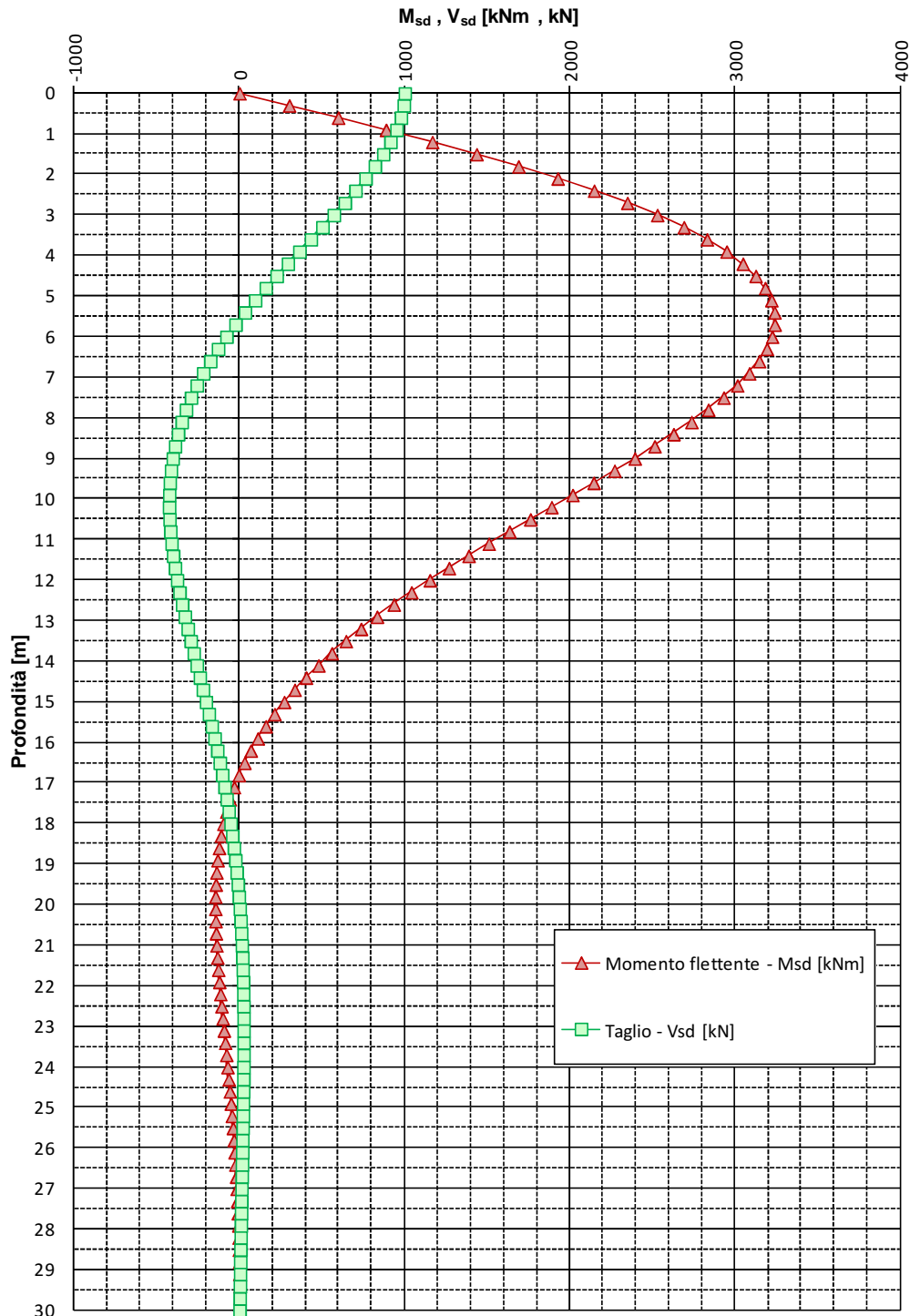
FIGURA 6-5: ANDAMENTO DELLE SOLLECITAZIONI FLETTENTE E TAGLIANTE (TAGLIO IN TESTA) – PALI TRIVELLATI \phi 1200
