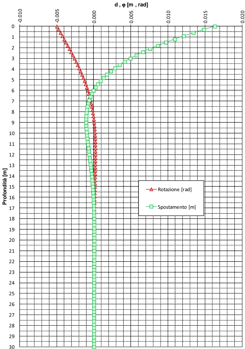
FIGURA 6-4: SPOSTAMENTI E ROTAZIONI (MOMENTO IN TESTA) – PALI TRIVELLATI \phi 1000
