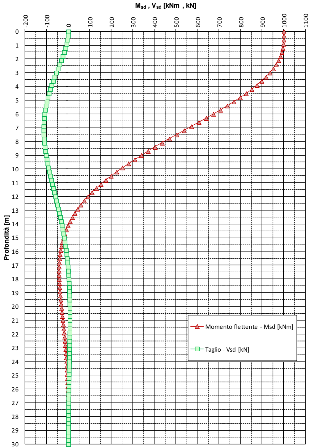
FIGURA 6-7: ANDAMENTO DELLE SOLLECITAZIONI FLETTENTE E TAGLIANTE (MOMENTO IN TESTA) – PALI TRIVELLATI \phi 1200
