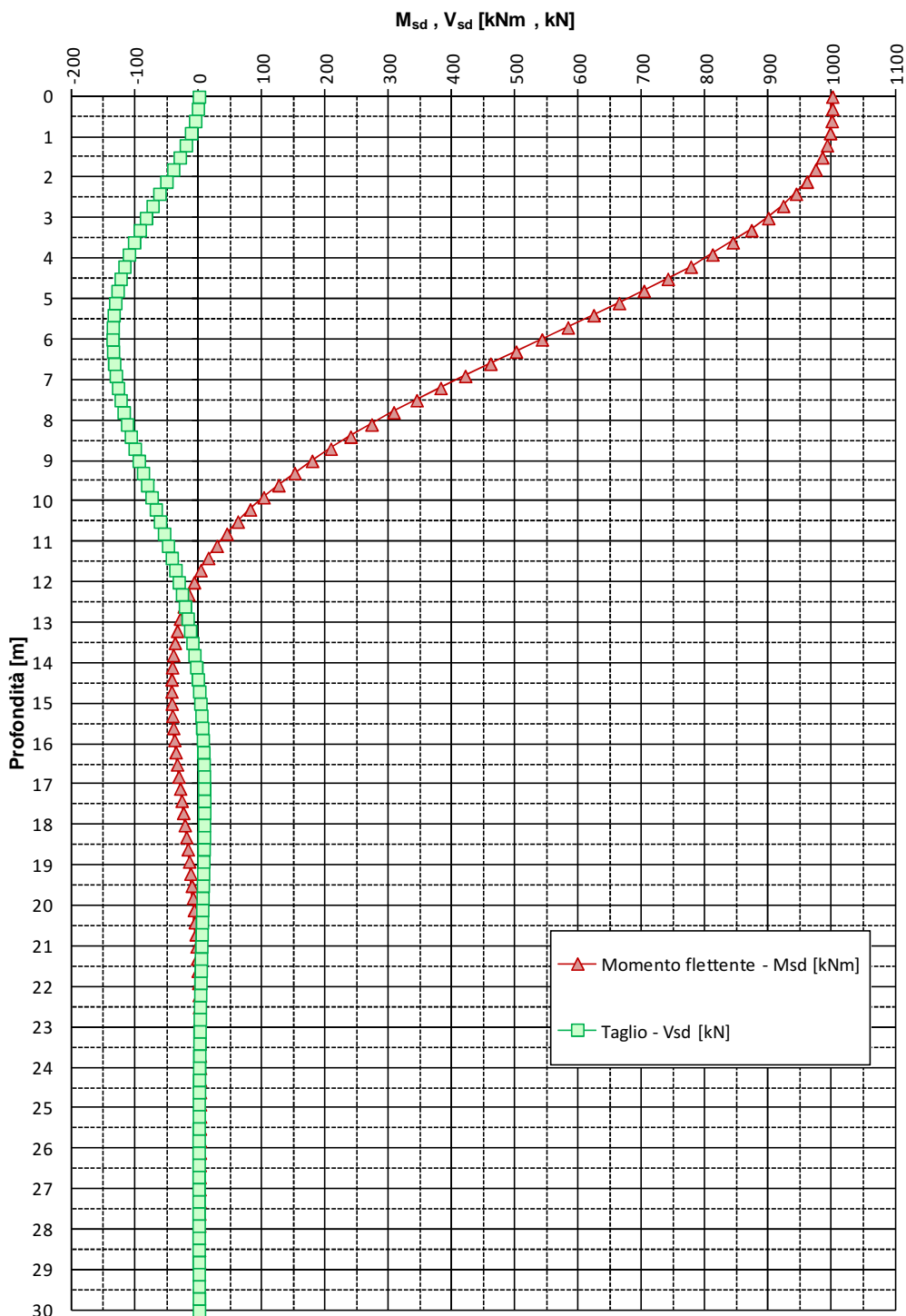
FIGURA 6-3: ANDAMENTO DELLE SOLLECITAZIONI FLETTENTE E TAGLIANTE (MOMENTO IN TESTA) – PALI TRIVELLATI \phi 1000
