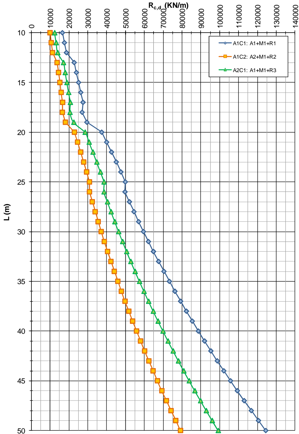
FIGURA 4-5: CAPACITÀ PORTANTE A COMPRESSIONE – POZZO DI DIAFRAMMI 12.5M X 7.0M
