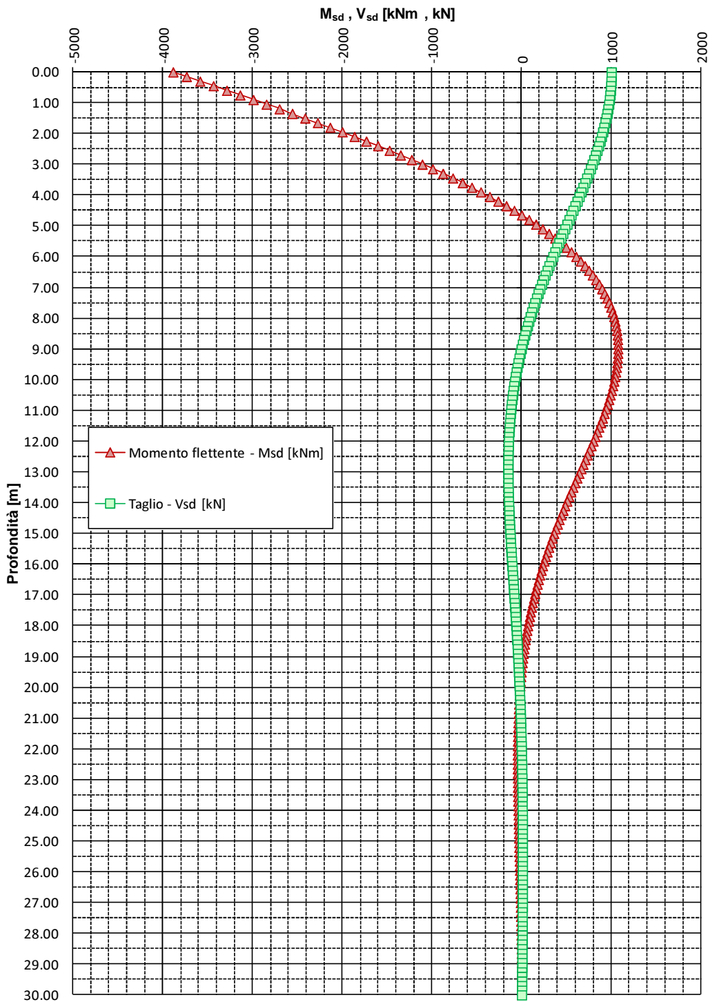
FIGURA 6-1: ANDAMENTO DELLE SOLLECITAZIONI FLETTENTE E TAGLIANTE – PALI TRIVELLATI \phi 1200
