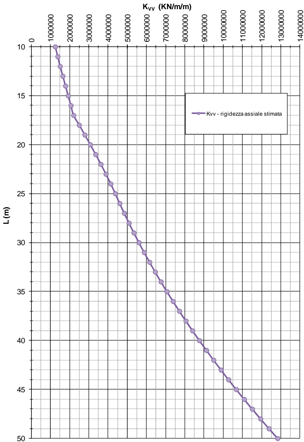
FIGURA 10-4: RIGIDEZZA VERTICALE – POZZO DI DIAFRAMMI 12.5M X 7.0M
