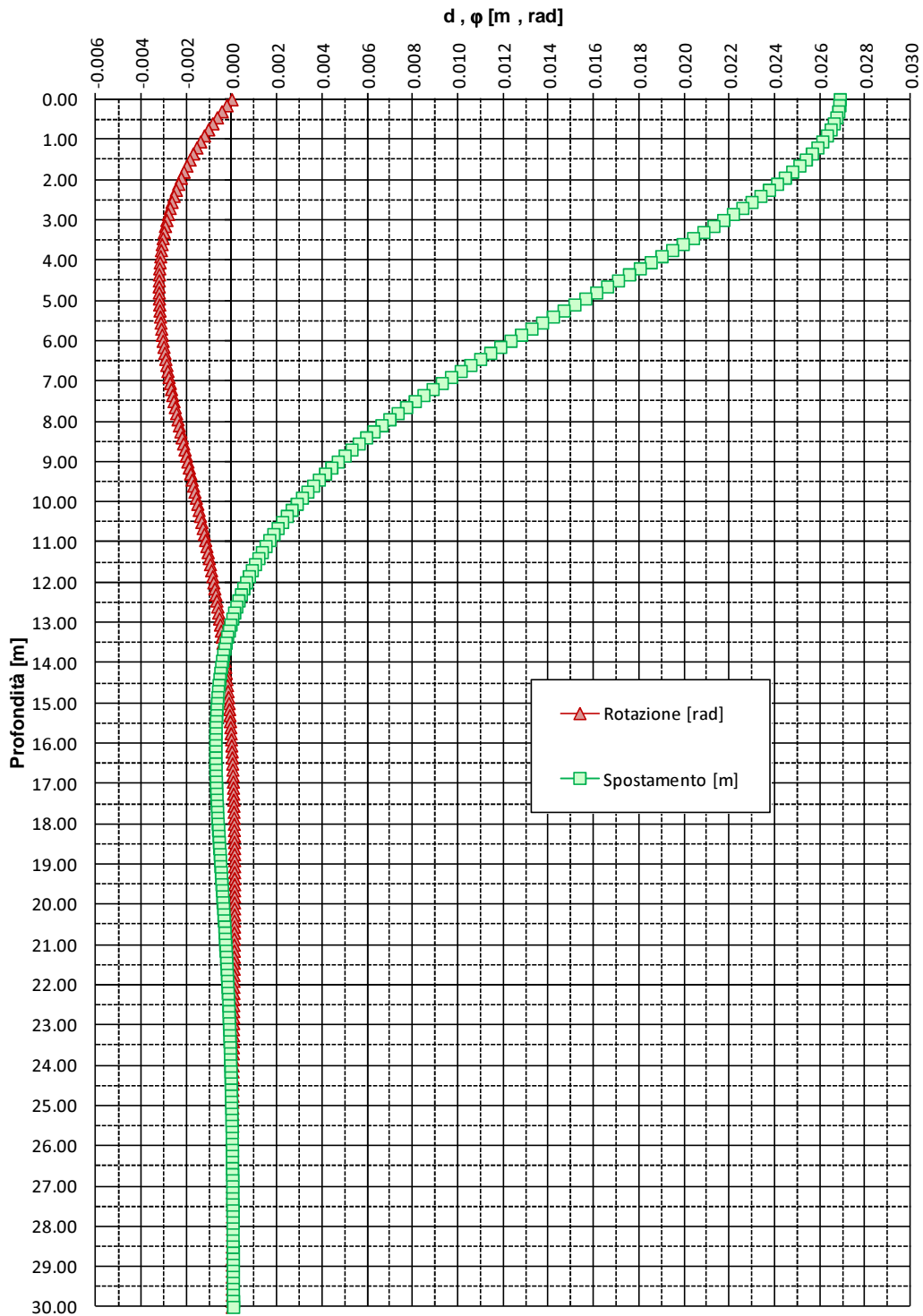
FIGURA 6-2: SPOSTAMENTI E ROTAZIONI – PALI TRIVELLATI φ 1200
