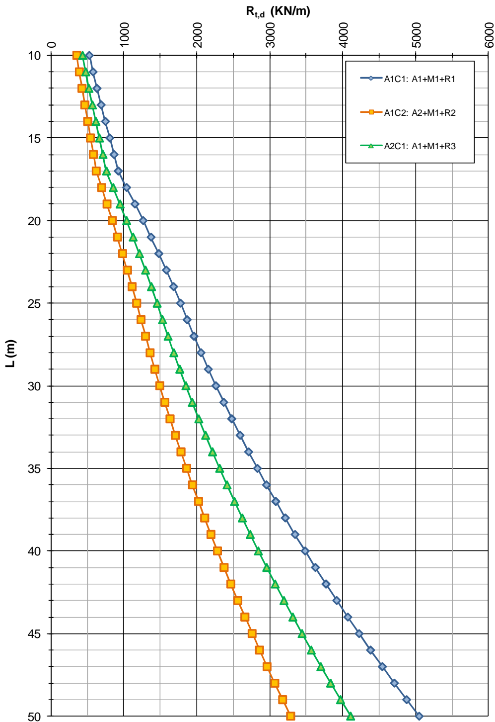
FIGURA 4-4: CAPACITÀ PORTANTE A TRAZIONE – DIAFRAMMI S 1000
