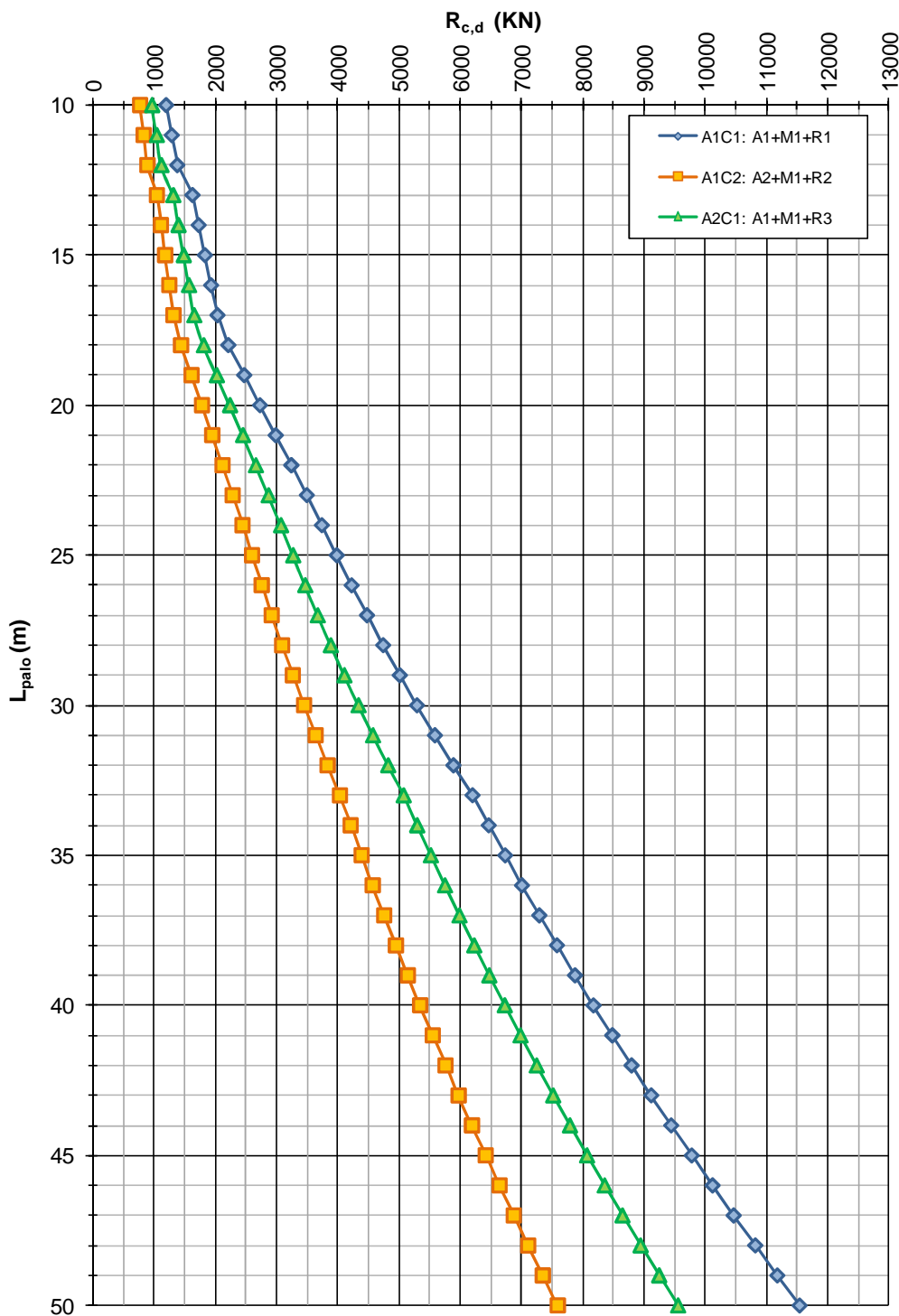
FIGURA 4-1: CAPACITÀ PORTANTE A COMPRESSIONE – PALI TRIVELLATI \phi 1200
