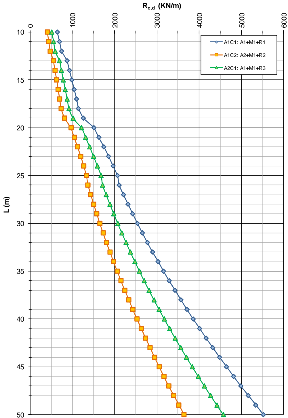
FIGURA 4-3: CAPACITÀ PORTANTE A COMPRESSIONE – DIAFRAMMI S 1000
