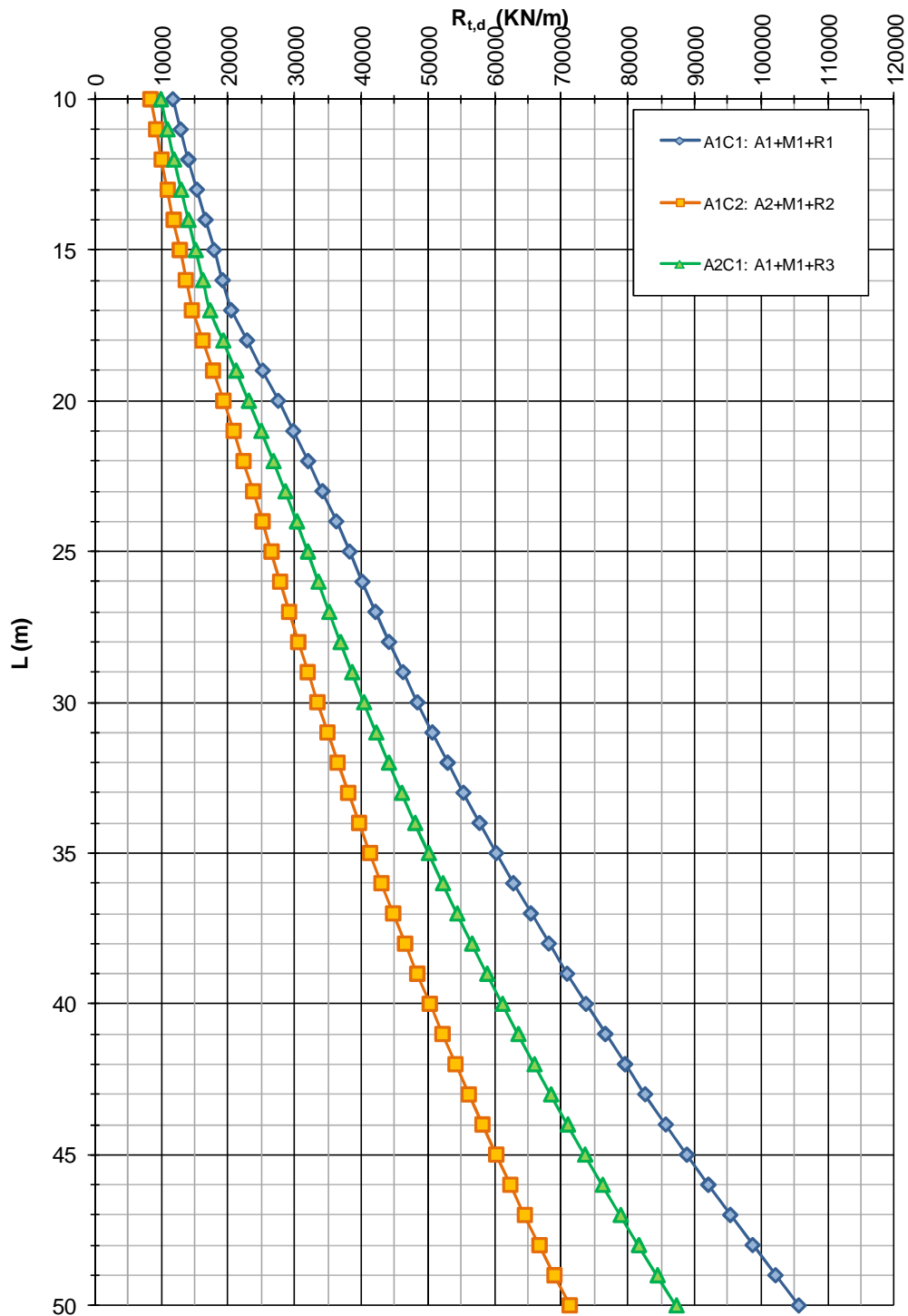
FIGURA 4-6: CAPACITÀ PORTANTE A TRAZIONE – POZZO DI DIAFRAMMI 12.5M X 7.0M
