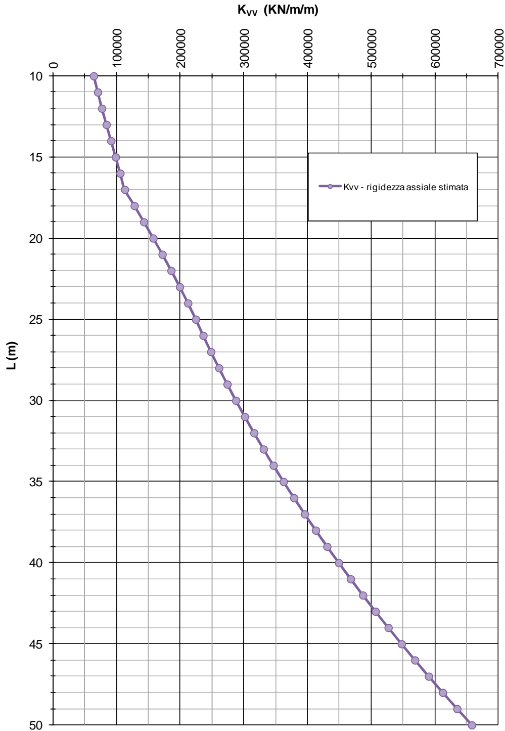
FIGURA 10-3: RIGIDEZZA VERTICALE – DIAFRAMMI S 1000
