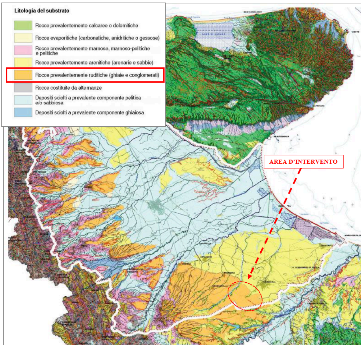
In figura: Inquadramento geologico regionale
