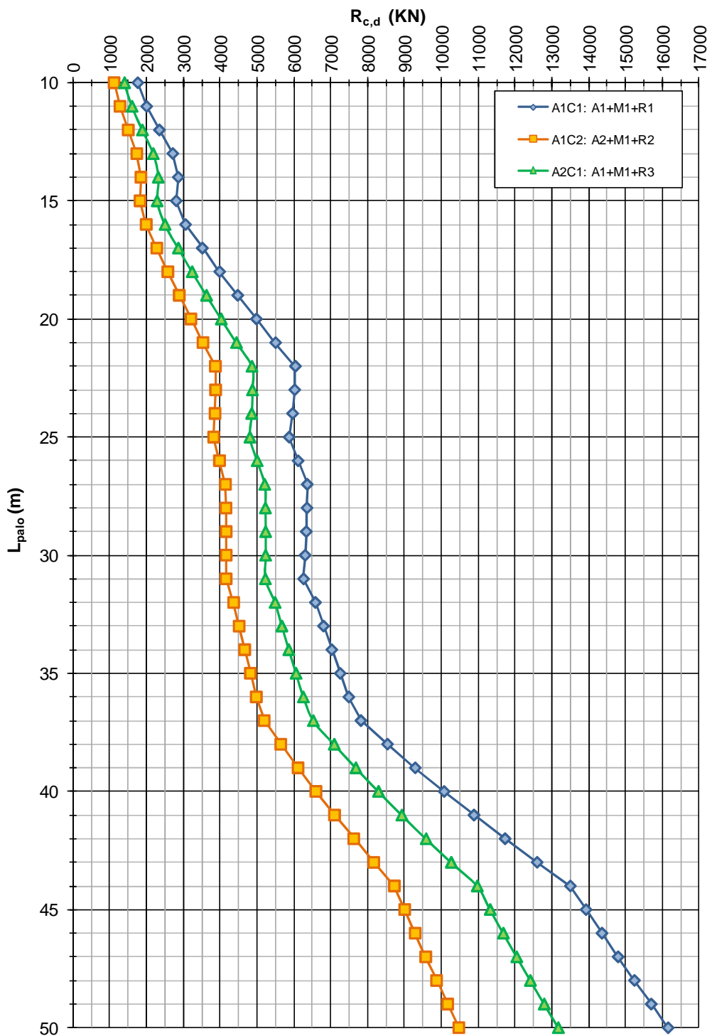
FIGURA 4-5: CAPACITÀ PORTANTE A COMPRESSIONE – PALI TRIVELLATI \phi 1500
