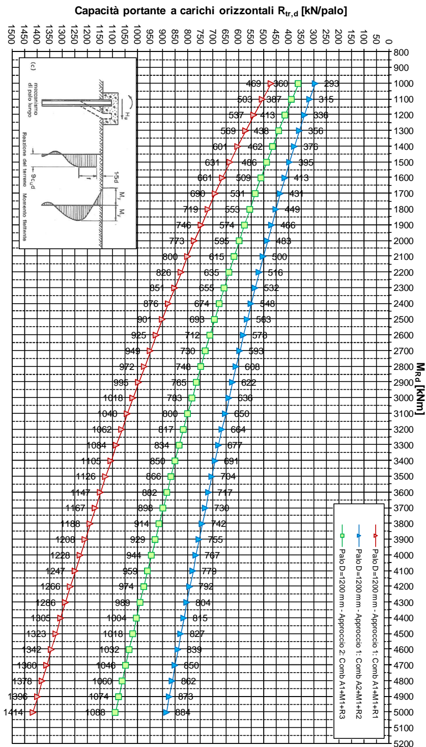
Capacità portante di progetto del singolo palo soggetto a carichi trasversali - R_{tr,d} D = 1200 mm - condizione di incastro in testa Pali di fondazione - Opera APO16 - ZO A
