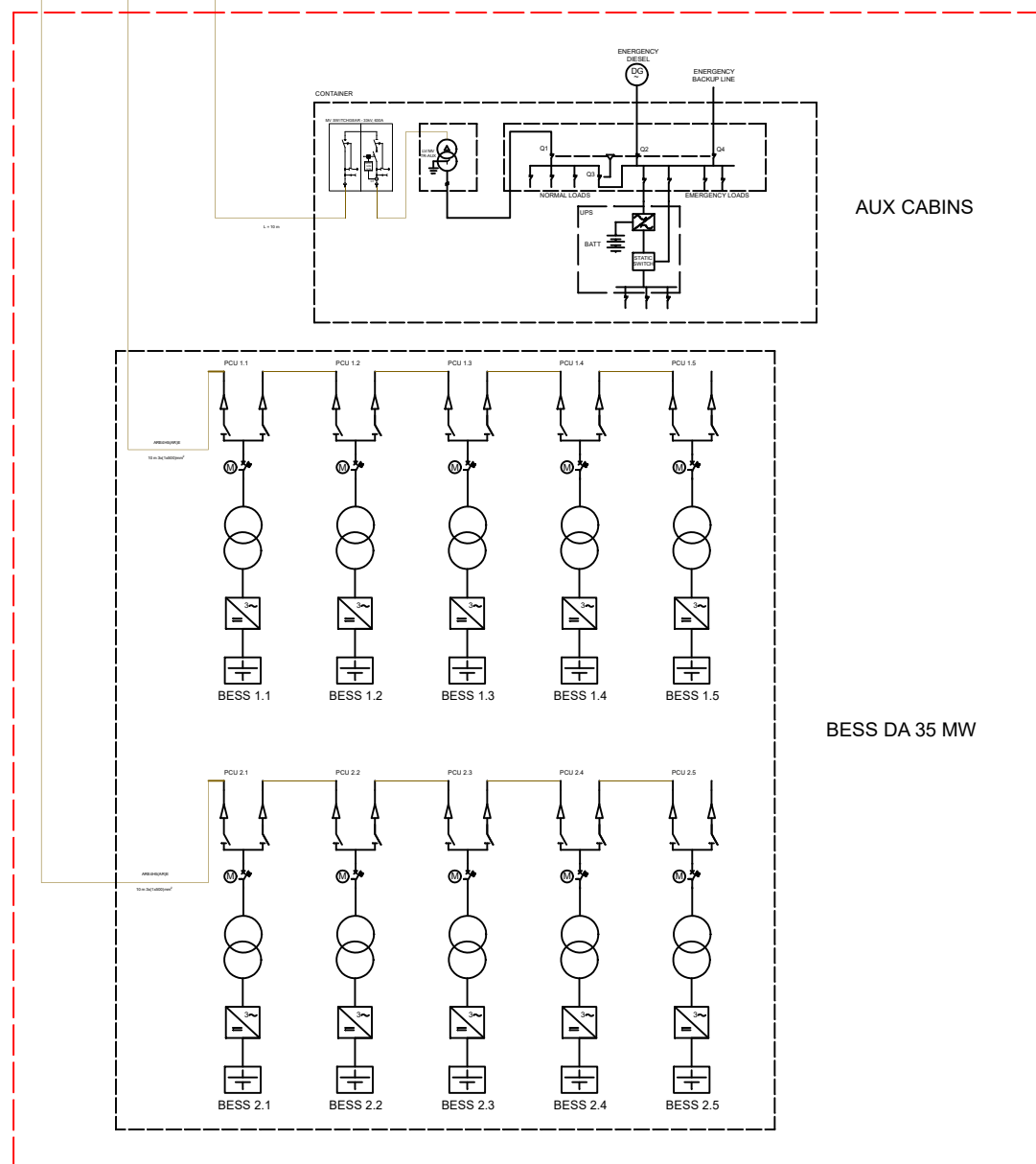
IMPIANTO BESS
