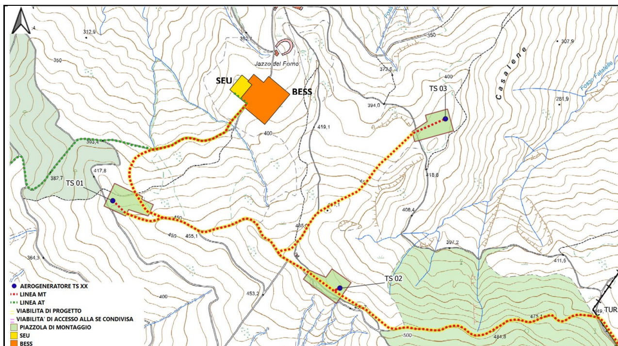
Figura 9.1: Localizzazione SEU 150/33 kV e BESS su CTR
