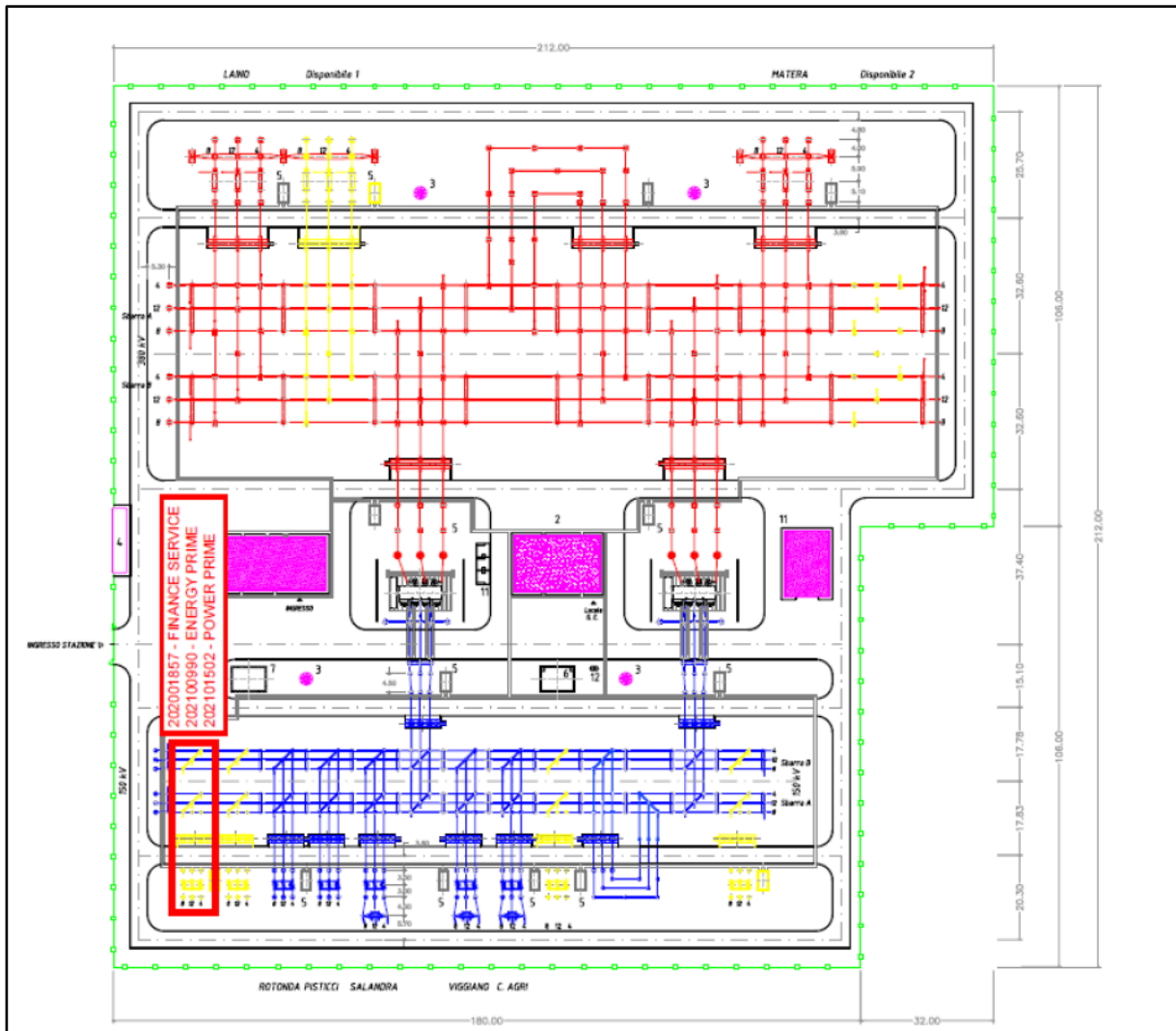
Figura 12.2: Planimetria della SE RTN a 380/150 kV con l'ubicazione dello stallo condiviso
