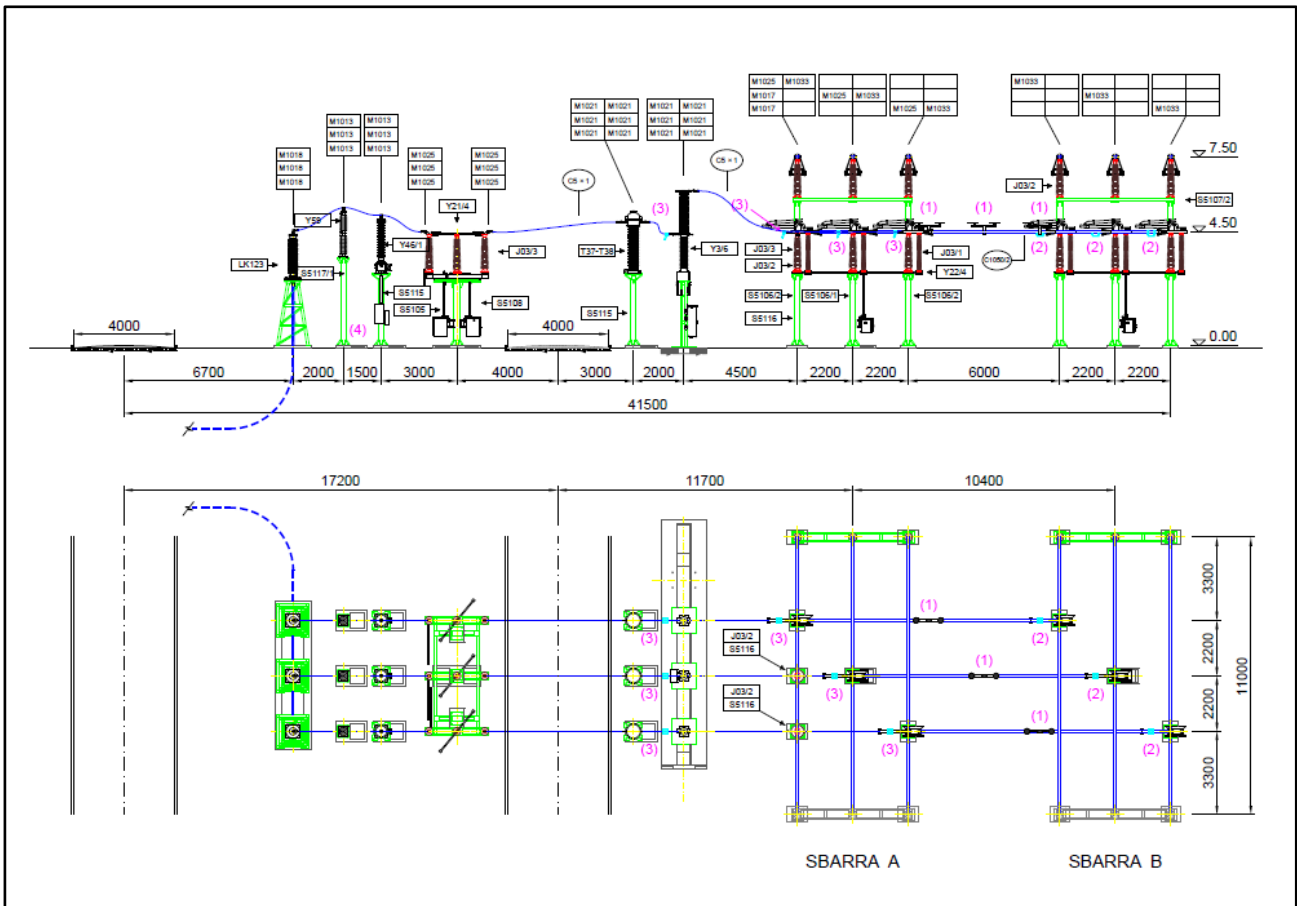
Figura 12.3: Planimetria e sezione elettromeccanica relativa alle apparecchiature dello stallo 150 kV nella stazione Terna
