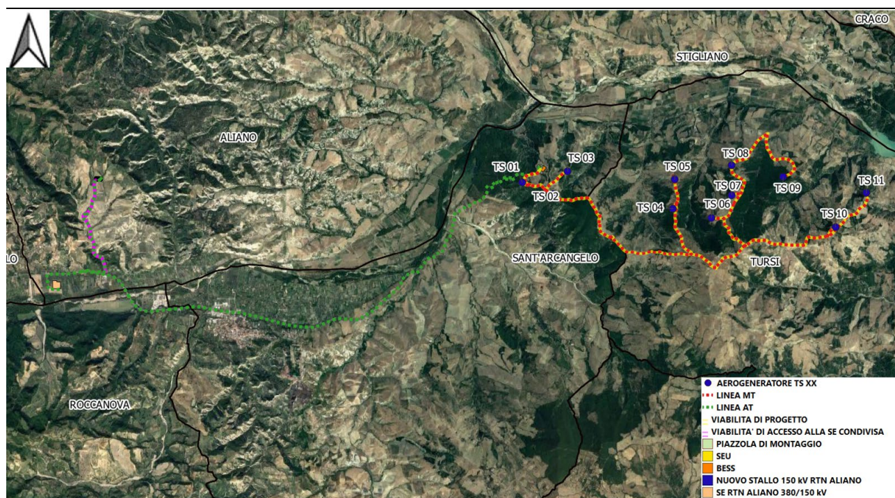
Figura 4.1: Layout d'impianto su ortofoto
