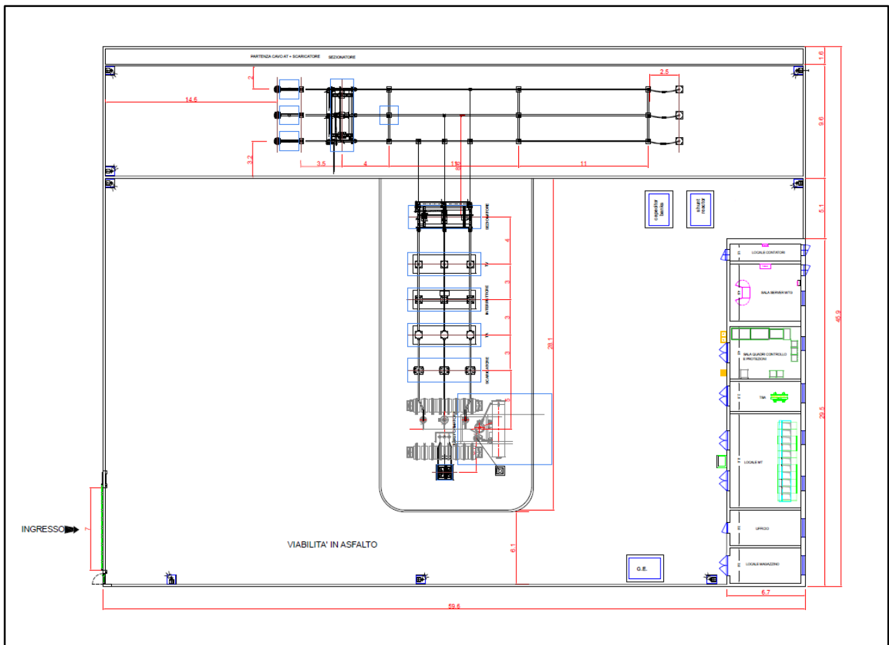
Figura 7.1: Planimetria elettromeccanica della Stazione di trasformazione 150/33 kV
