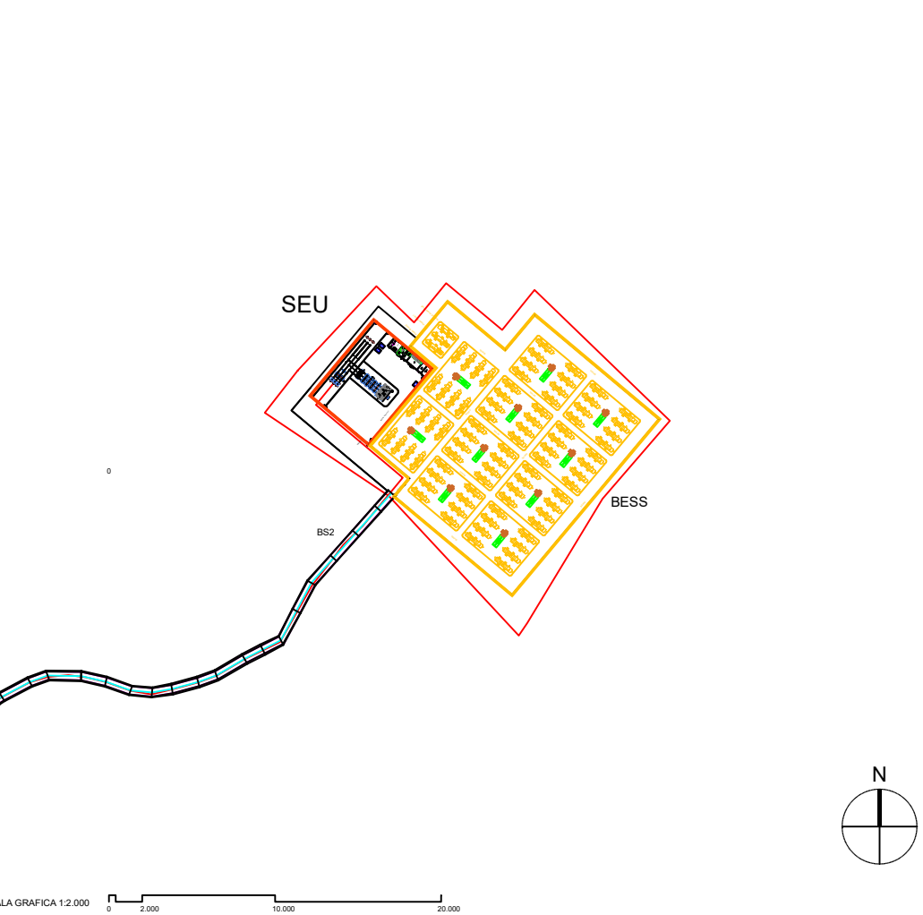
C_INQUADRAMENTO SEU SU CTR_SCALE 1:2.000
