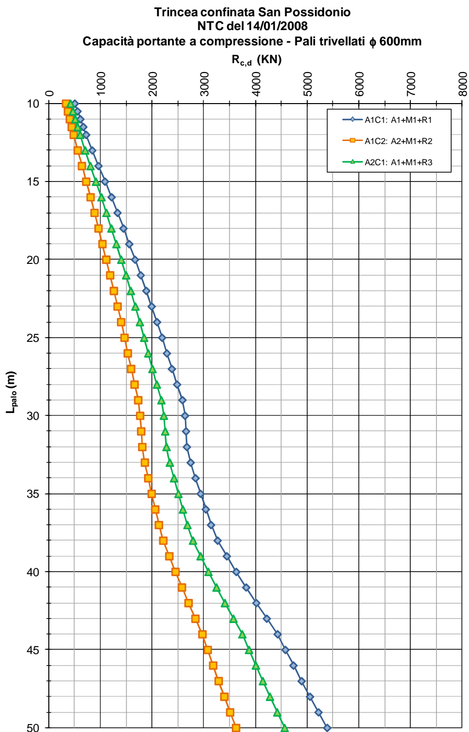
FIGURA 4-1: CAPACITÀ PORTANTE A COMPRESSIONE – PALI TRIVELLATI \phi 600
