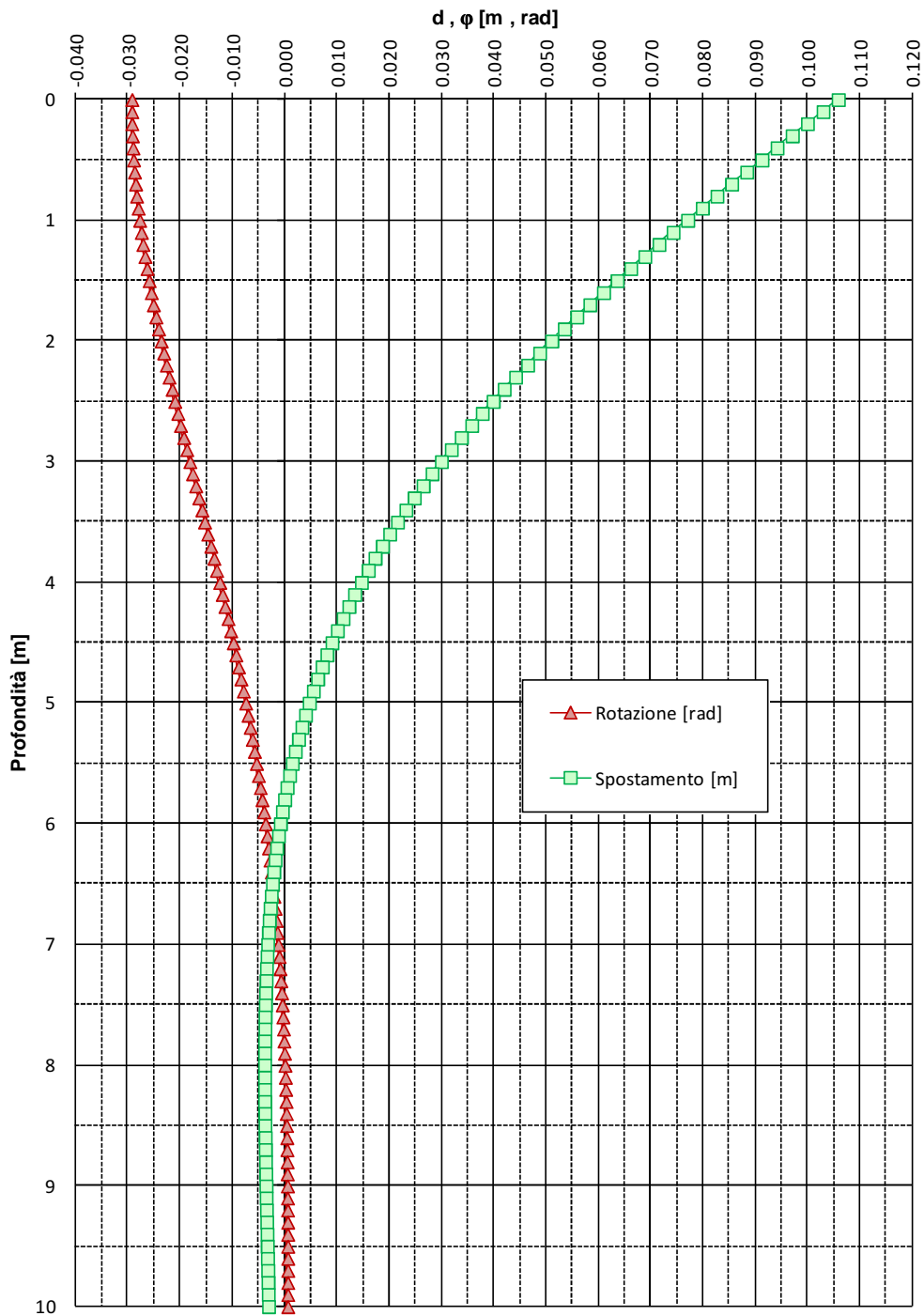
FIGURA 6-2: SPOSTAMENTI E ROTAZIONI – PALI TRIVELLATI \phi 600 (TAGLIO IN TESTA)
