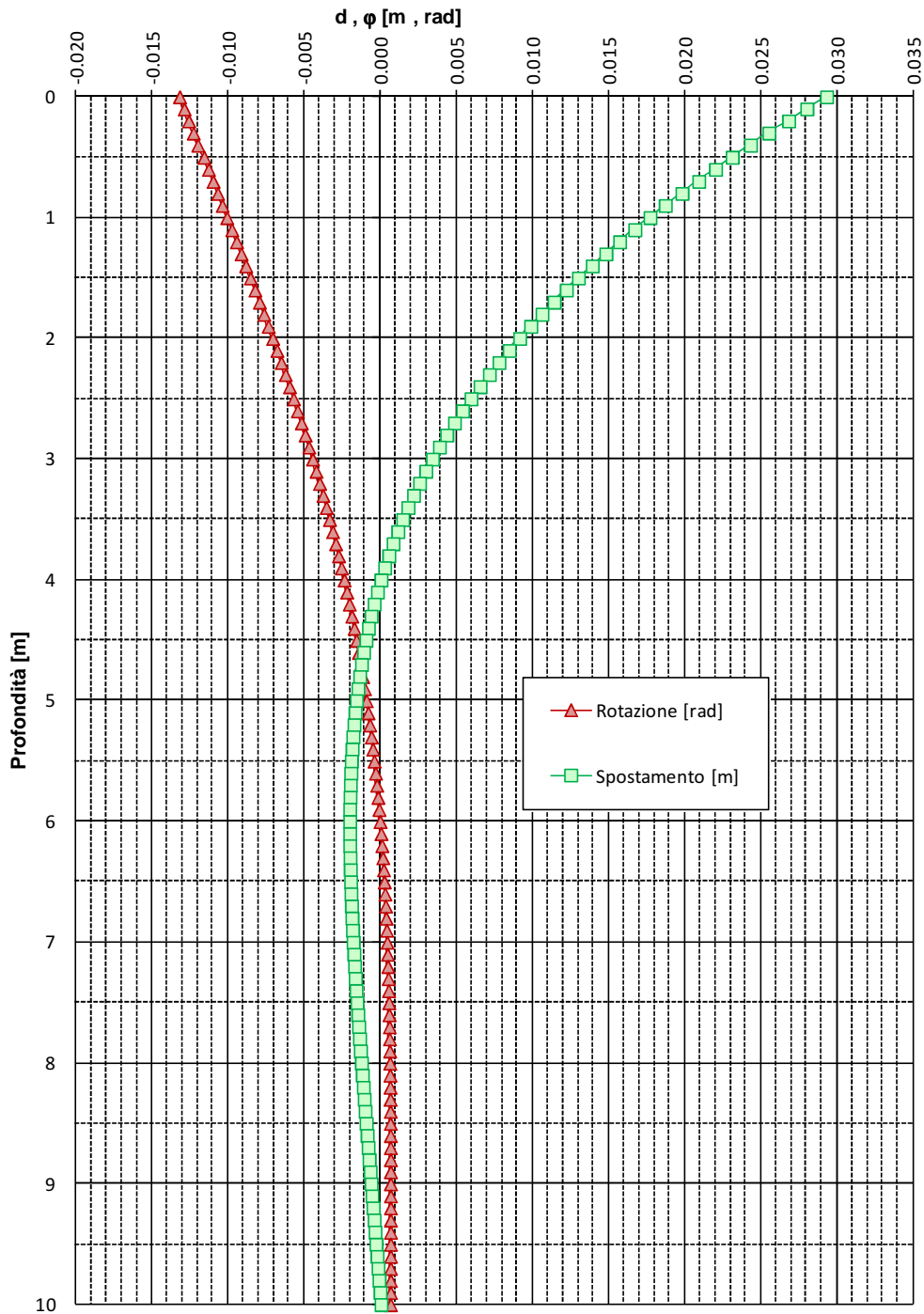
FIGURA 6-4: SPOSTAMENTI E ROTAZIONI – PALI TRIVELLATI \phi 600 (MOMENTO IN TESTA)
