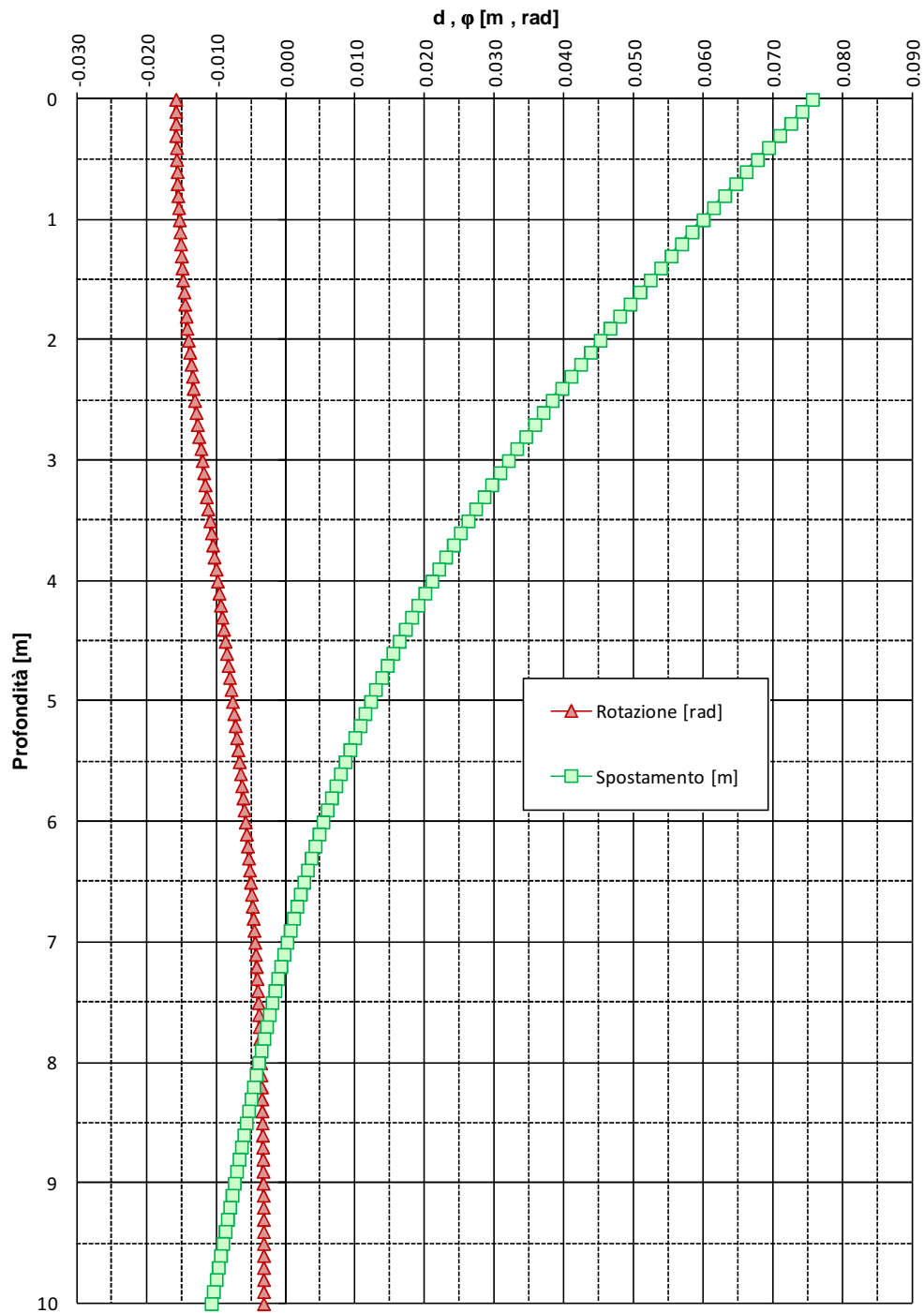
FIGURA 6-6: SPOSTAMENTI E ROTAZIONI – PALI TRIVELLATI \phi 800 (TAGLIO IN TESTA)
