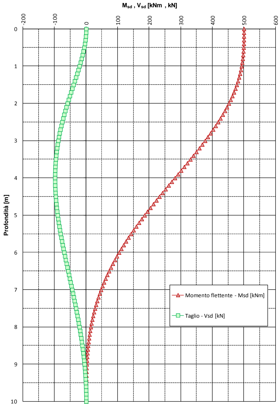
FIGURA 6-3: ANDAMENTO DELLE SOLLECITAZIONI FLETTENTE E TAGLIANTE – PALI TRIVELLATI \phi 600 (MOMENTO IN TESTA)
