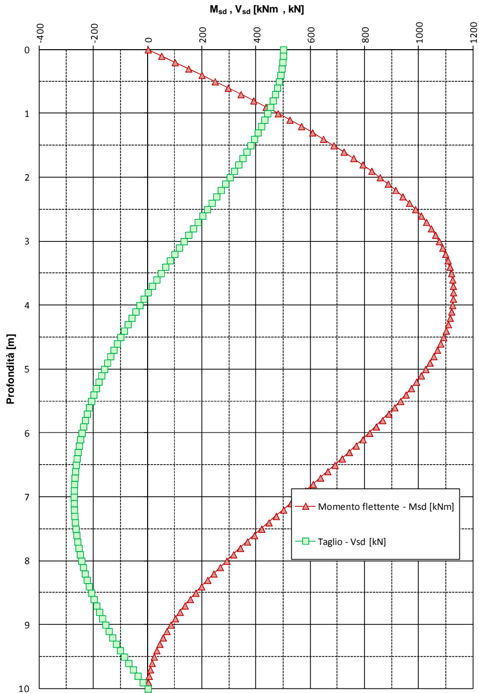
FIGURA 6-5: ANDAMENTO DELLE SOLLECITAZIONI FLETTENTE E TAGLIANTE – PALI TRIVELLATI \phi 800 (TAGLIO IN TESTA)
