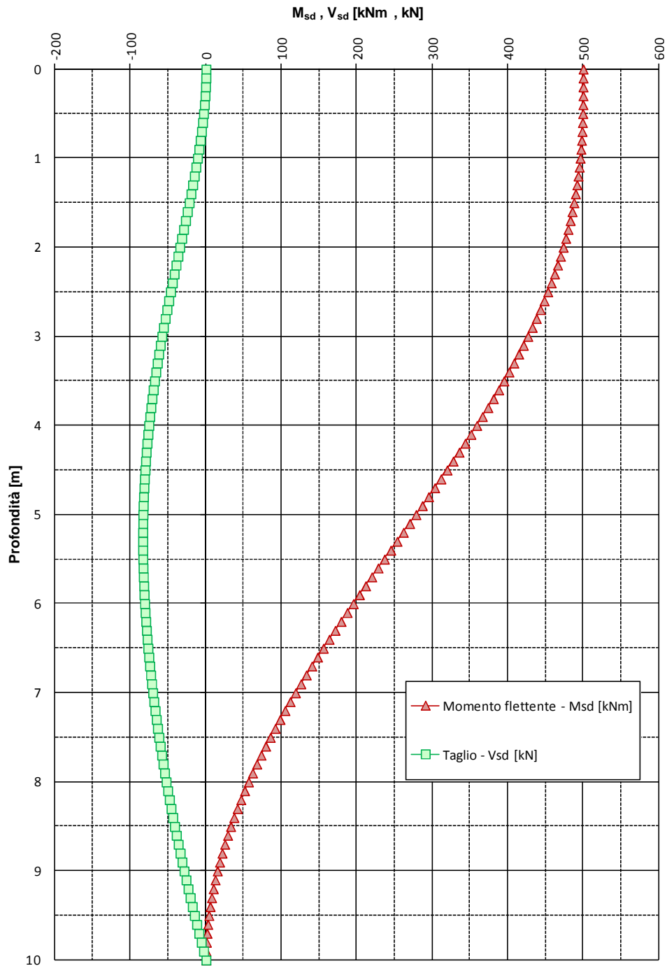
FIGURA 6-7: ANDAMENTO DELLE SOLLECITAZIONI FLETTENTE E TAGLIANTE – PALI TRIVELLATI \phi 800 (MOMENTO IN TESTA)
