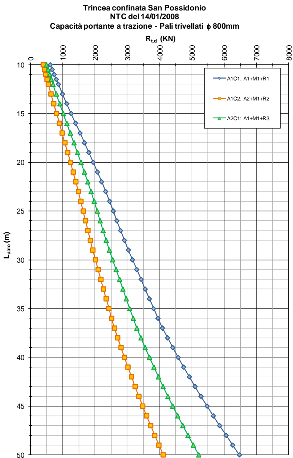
FIGURA 4-4: CAPACITÀ PORTANTE A TRAZIONE – PALI TRIVELLATI \phi 800
