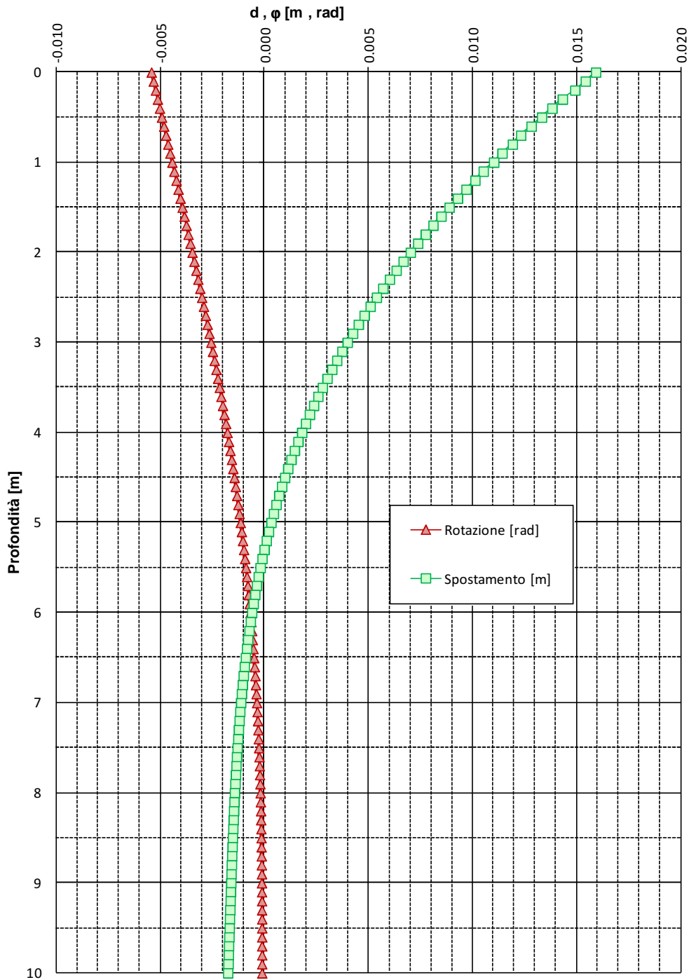
FIGURA 6-8: SPOSTAMENTI E ROTAZIONI – PALI TRIVELLATI \phi 800 (MOMENTO IN TESTA)
