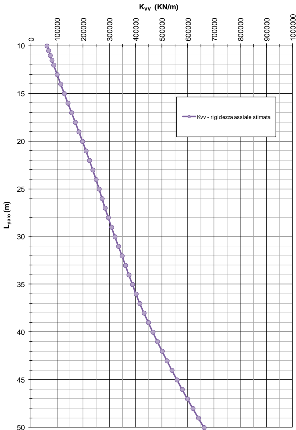
FIGURA 10_2: RIGIDEZZA VERTICALE – PALI TRIVELLATI \phi 600
