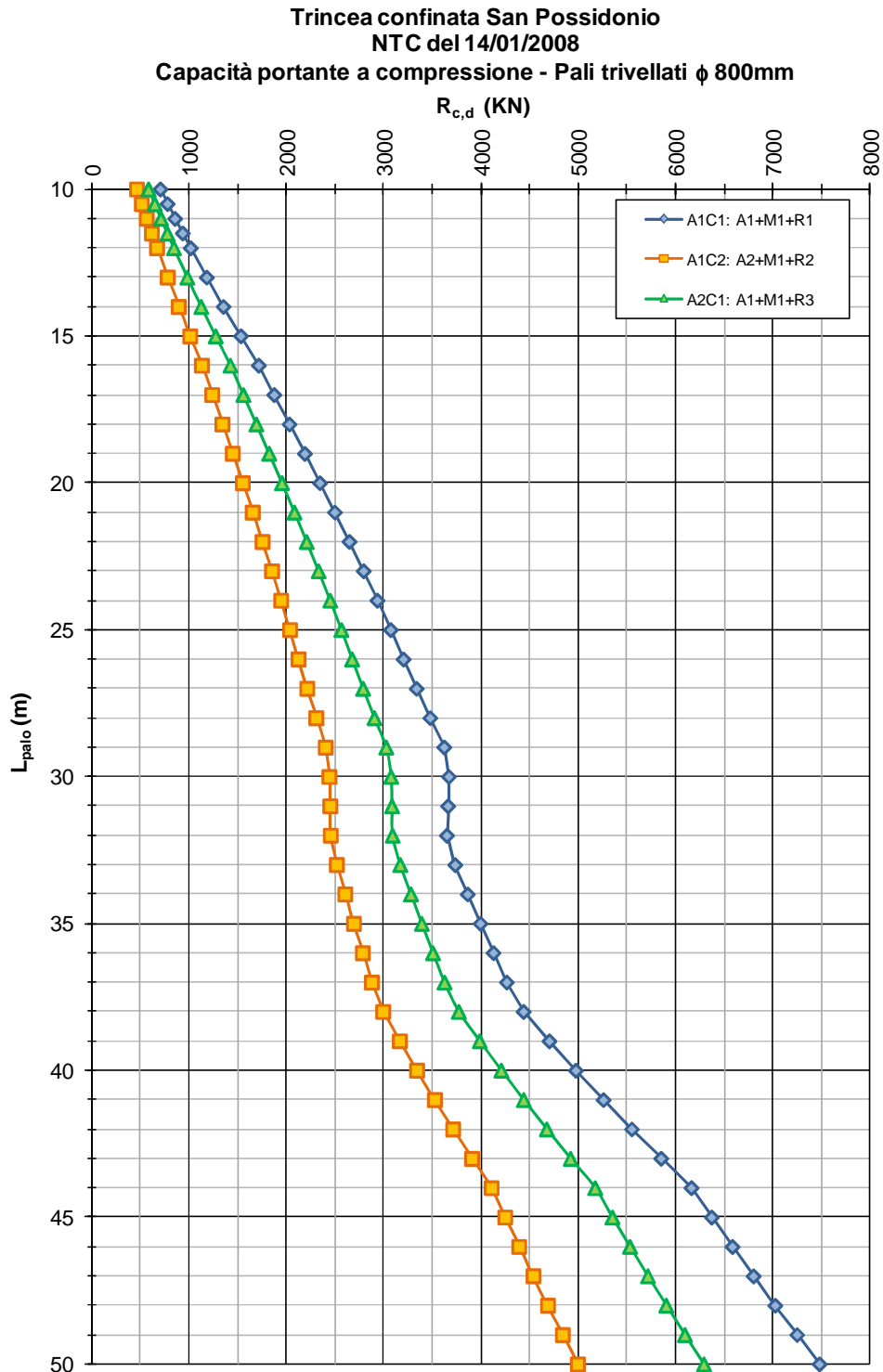
FIGURA 4-3: CAPACITÀ PORTANTE A COMPRESSIONE – PALI TRIVELLATI \phi 800
