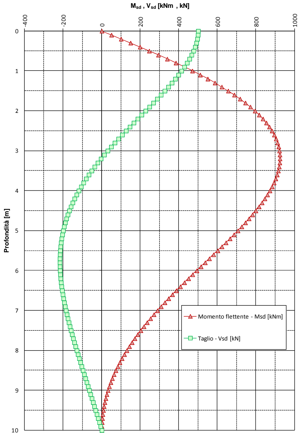
FIGURA 6-1: ANDAMENTO DELLE SOLLECITAZIONI FLETTENTE E TAGLIANTE – PALI TRIVELLATI \phi 600 (TAGLIO IN TESTA)
