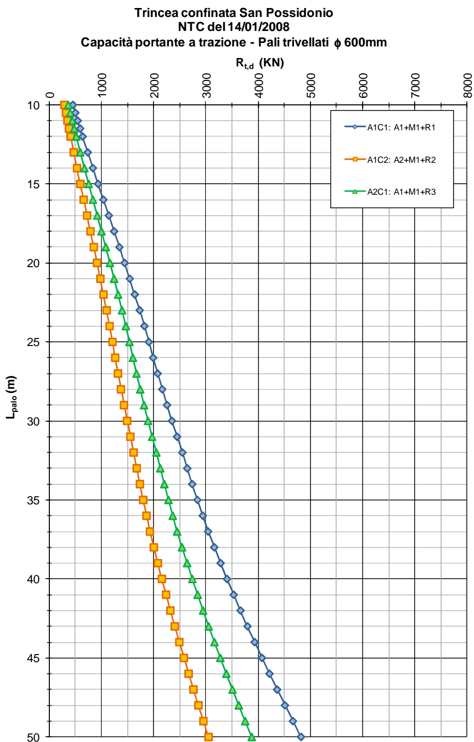
FIGURA 4-2: CAPACITÀ PORTANTE A TRAZIONE – PALI TRIVELLATI \phi 600
