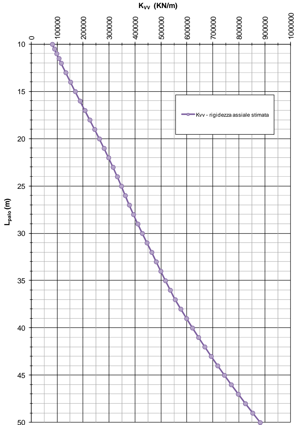
FIGURA 10_3: RIGIDEZZA VERTICALE – PALI TRIVELLATI \phi 800
