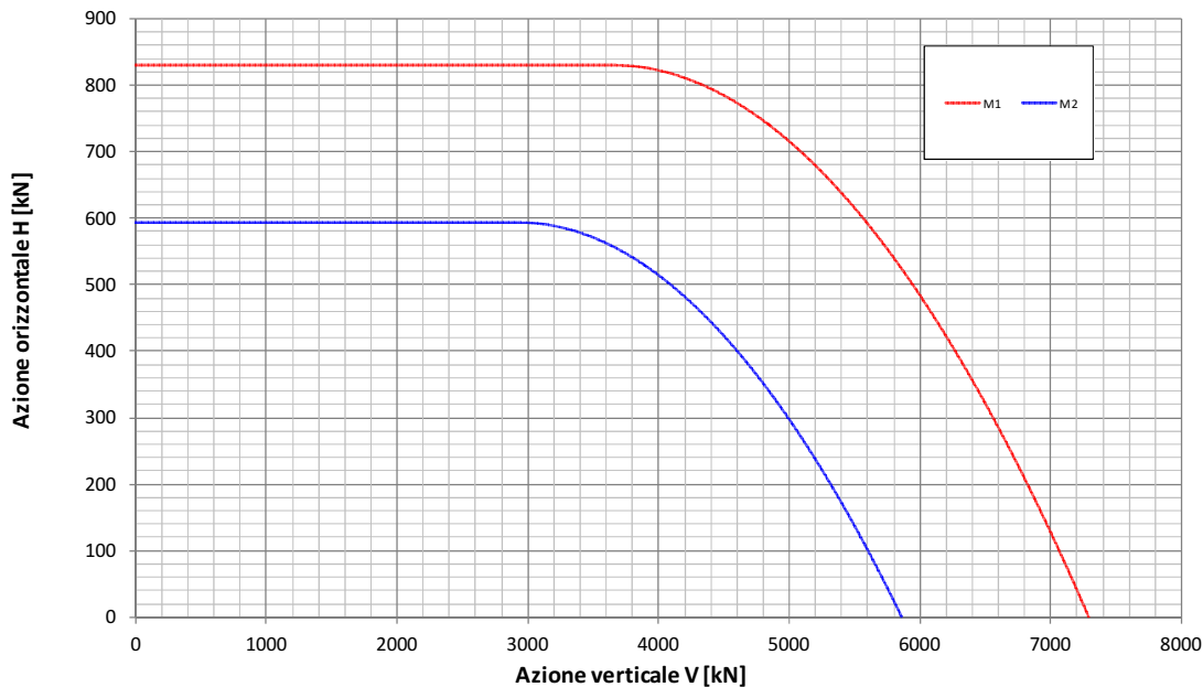
Fondazione B=16.6m - Approfondimento D=7.3m Condizione Statica Non Drenata Dominio di interazione nel piano V-H ( Gourvenec, 2007 )
