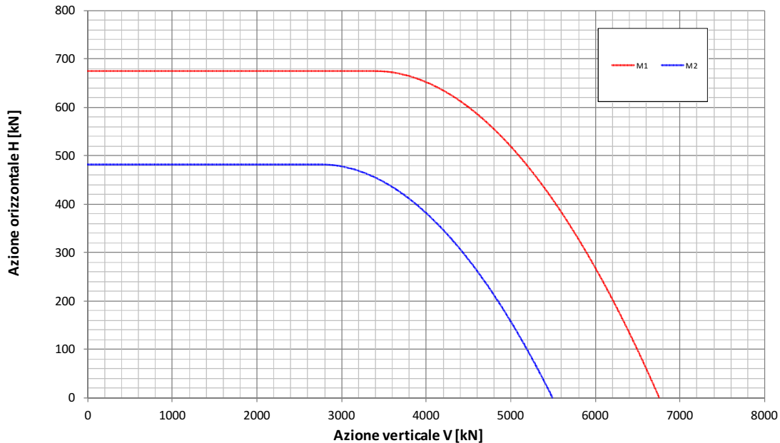
Fondazione B=13.5m - Approfondimento D=9.2m Condizione Statica Non Drenata Dominio di interazione nel piano V-H (Gourvenec, 2007)
