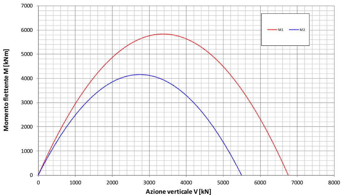
Fondazione B=13.5m - Approfondimento D=9.2m Condizione Sismica Non Drenata Dominio di interazione nel piano V-M ( Gourvenec, 2007 )
