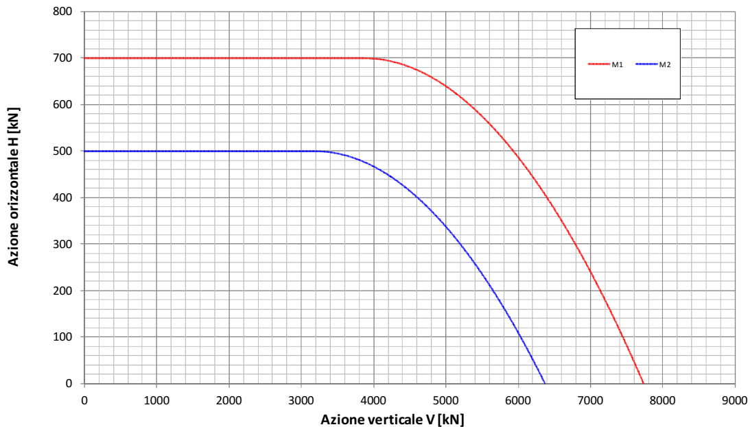
Fondazione B=14.0m - Approfondimento D=11.3m Condizione Statica Non Drenata Dominio di interazione nel piano V-H ( Gourvenec, 2007 )
