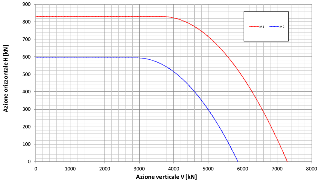
Fondazione B=16.6m - Approfondimento D=7.3m Condizione Sismica Non Drenata Dominio di interazione nel piano V-H (Gourvenec, 2007)
