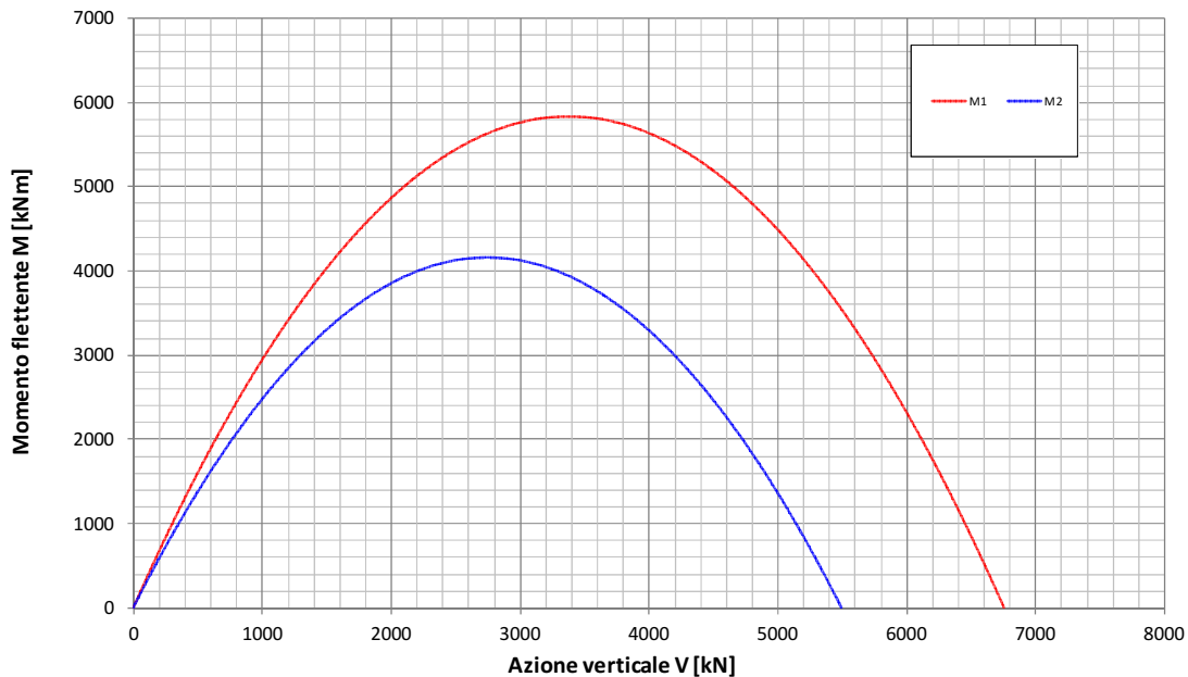
Fondazione B=13.5m - Approfondimento D=9.2m Condizione Statica Non Drenata Dominio di interazione nel piano V-M (Gourvenec, 2007)
