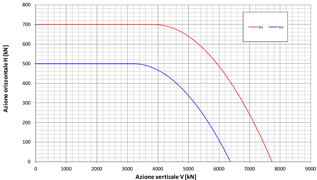
Fondazione B=14.0m - Approfondimento D=11.3m Condizione Sismica Non Drenata Dominio di interazione nel piano V-H ( Gourvenec, 2007 )
