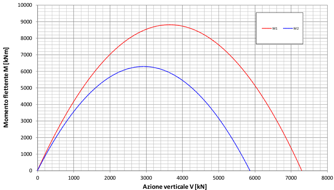
Fondazione B=16.6m - Approfondimento D=7.3m Condizione Sismica Non Drenata Dominio di interazione nel piano V-M (Gourvenec, 2007)
