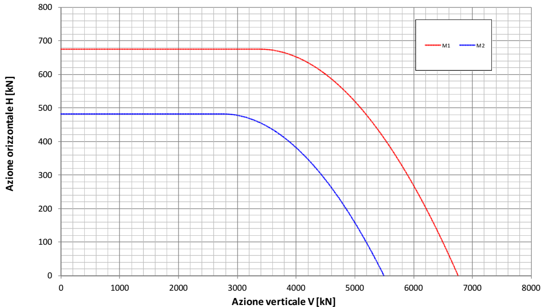
Fondazione B=13.5m - Approfondimento D=9.2m Condizione Sismica Non Drenata Dominio di interazione nel piano V-H ( Gourvenec, 2007 )
