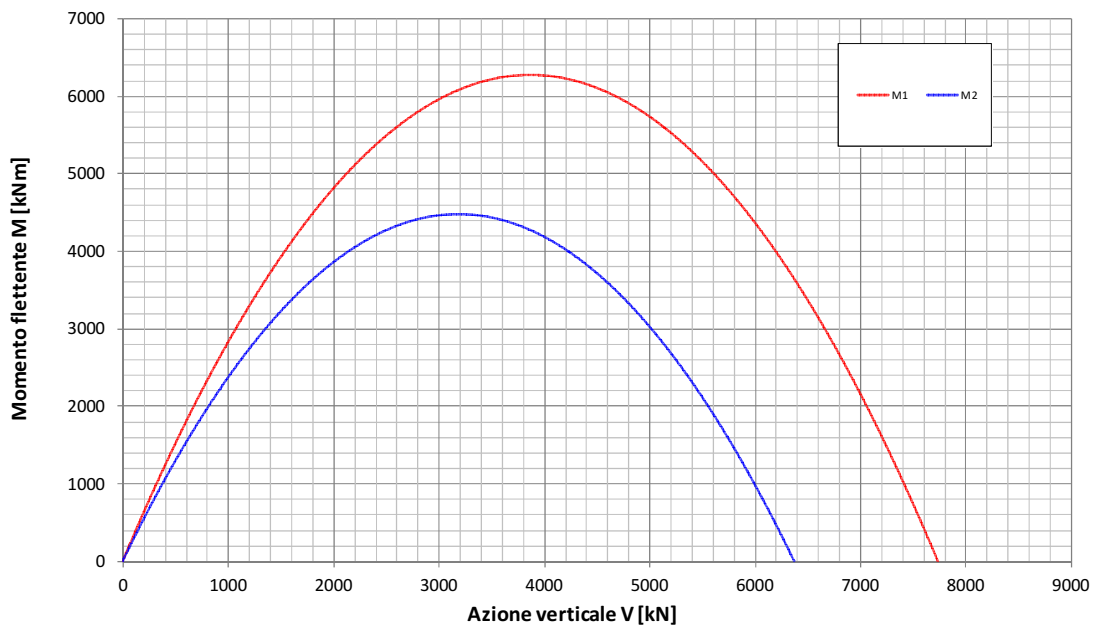
Fondazione B=14.0m - Approfondimento D=11.3m Condizione Statica Non Drenata Dominio di interazione nel piano V-M ( Gourvenec, 2007 )
