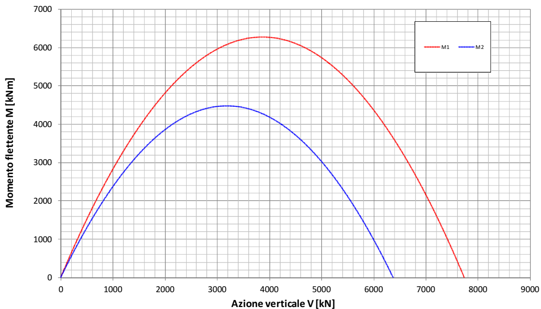
Fondazione B=14.0m - Approfondimento D=11.3m Condizione Sismica Non Drenata Dominio di interazione nel piano V-M ( Gourvenec, 2007 )
