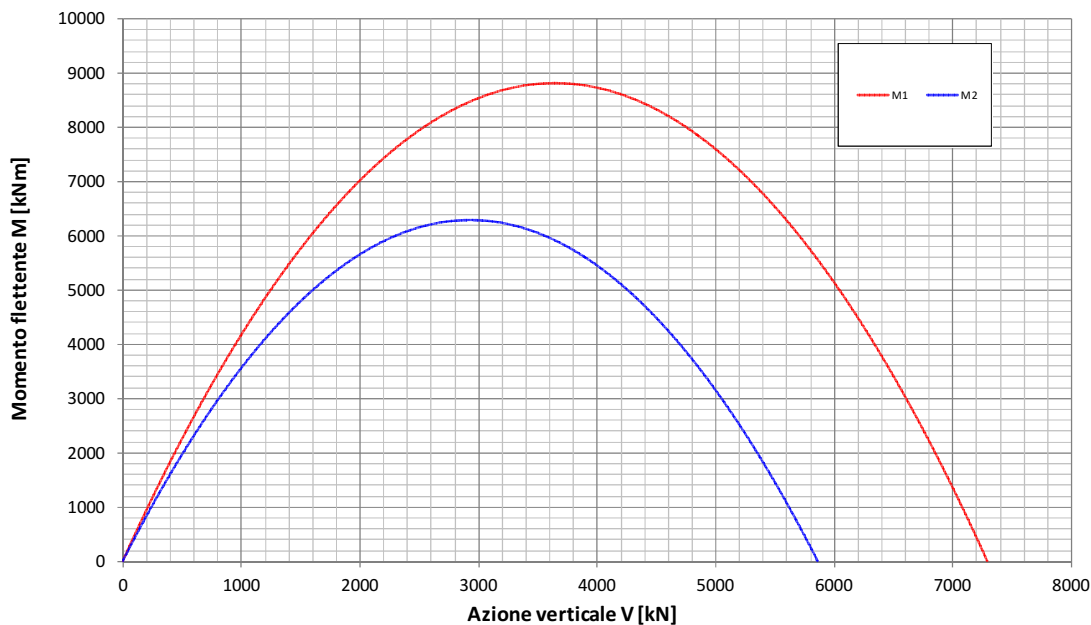
Fondazione B=16.6m - Approfondimento D=7.3m Condizione Statica Non Drenata Dominio di interazione nel piano V-M ( Gourvenec, 2007 )
