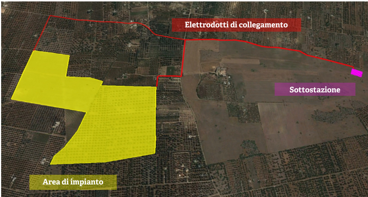
Figura 2 - Vista aerea dell'impianto fotovoltaico
