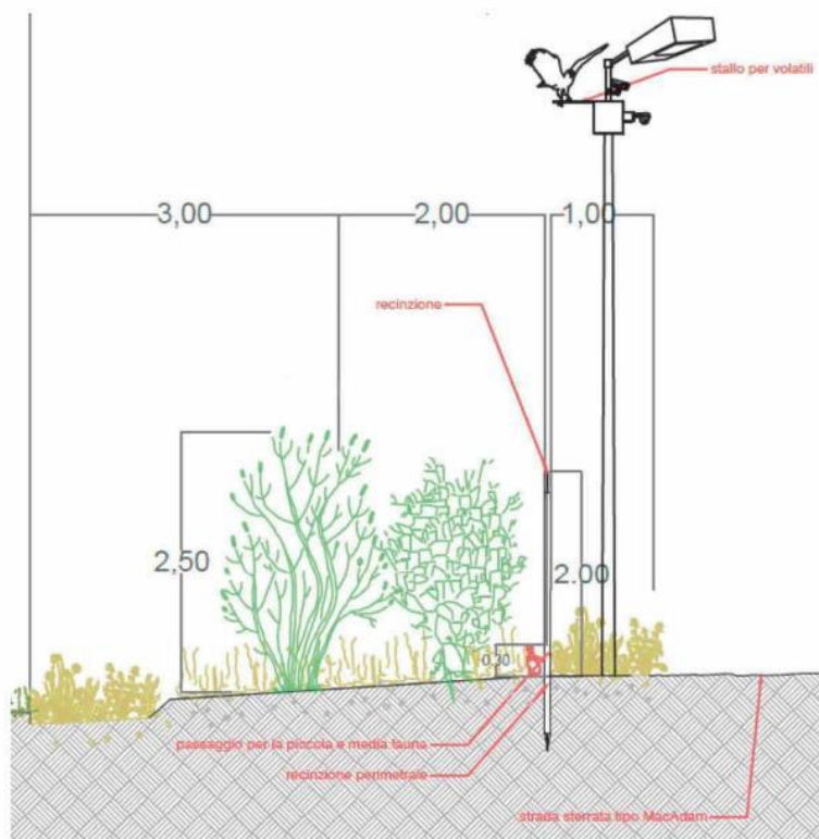
Figura 71 - Particolare dello stallo per volatili
