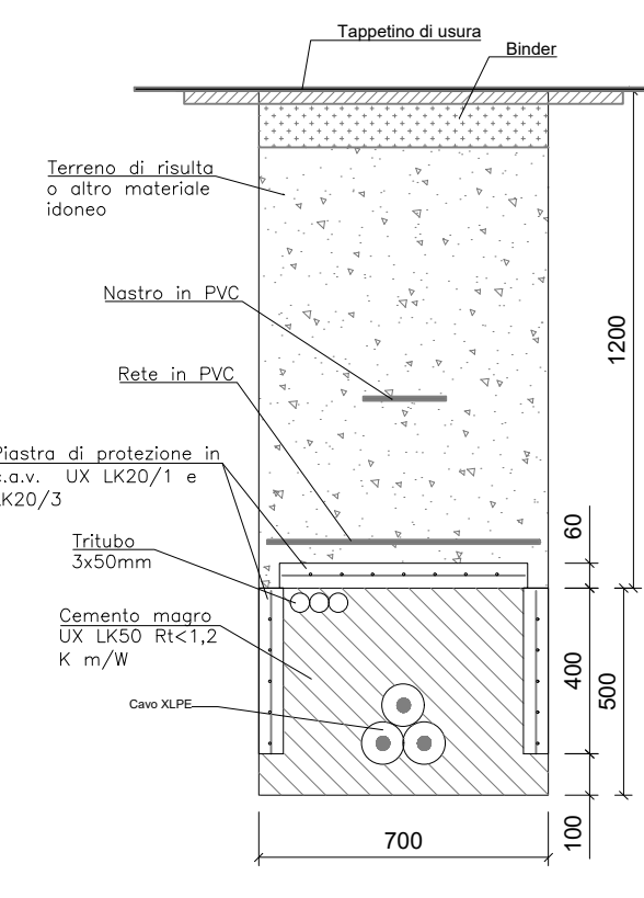
P-P ESEMPIO DI SEZIONE IN TRINCEA SU STRADA PER UNA TERZA
