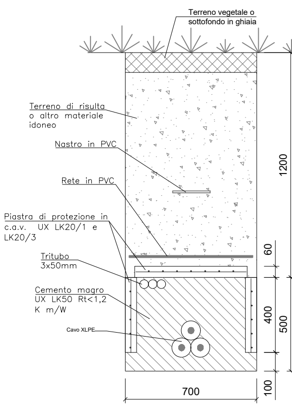
O-O ESEMPIO DI SEZIONE IN TRINCEA FUORI LA SEDE STRADALE
