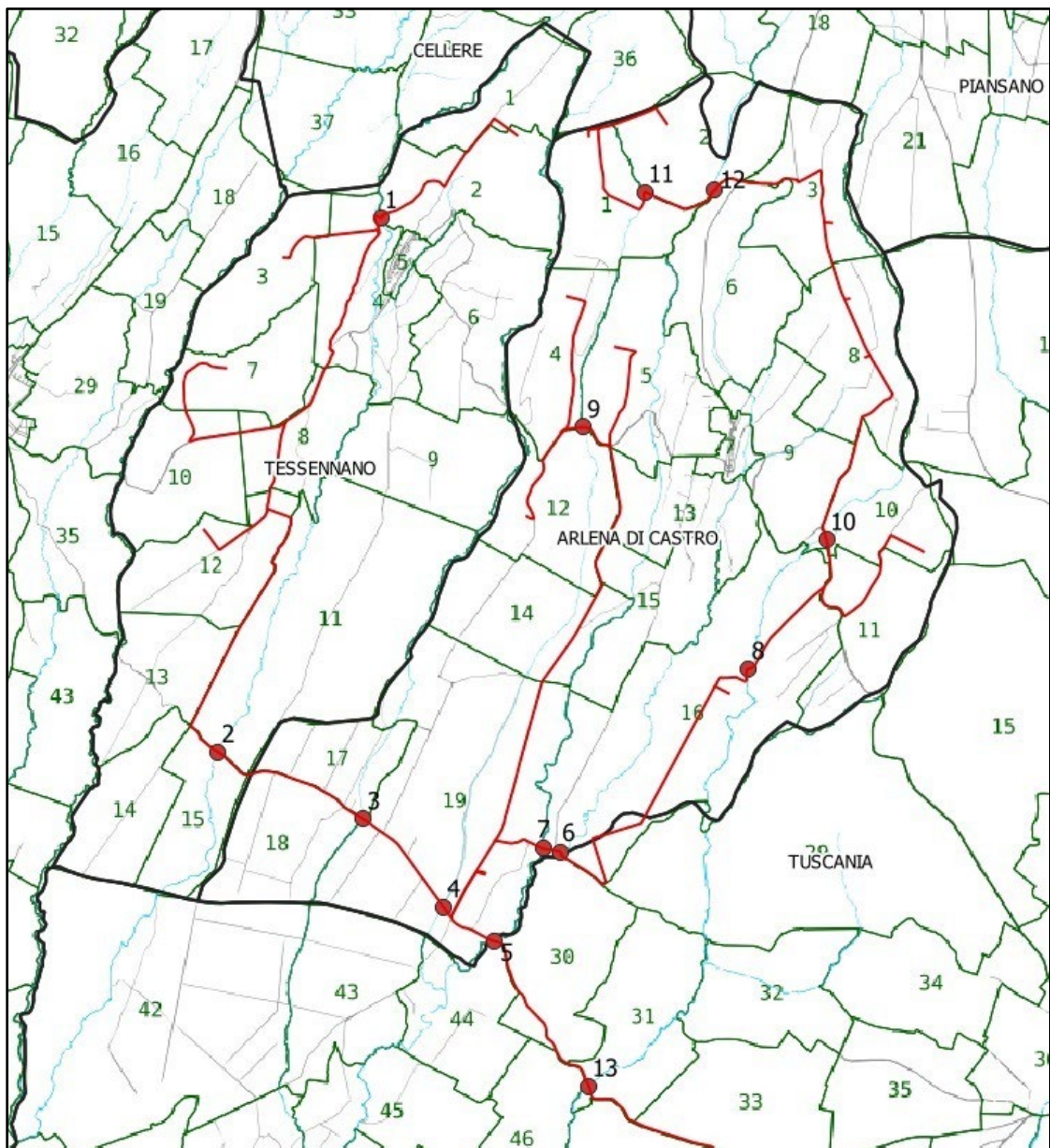
Figura 3 - Indicazione attraversamenti su planimetria catastale
