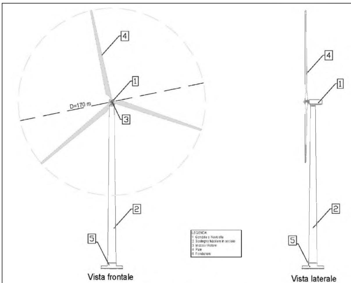
Figura 29 Prospetti dell'aerogeneratore
