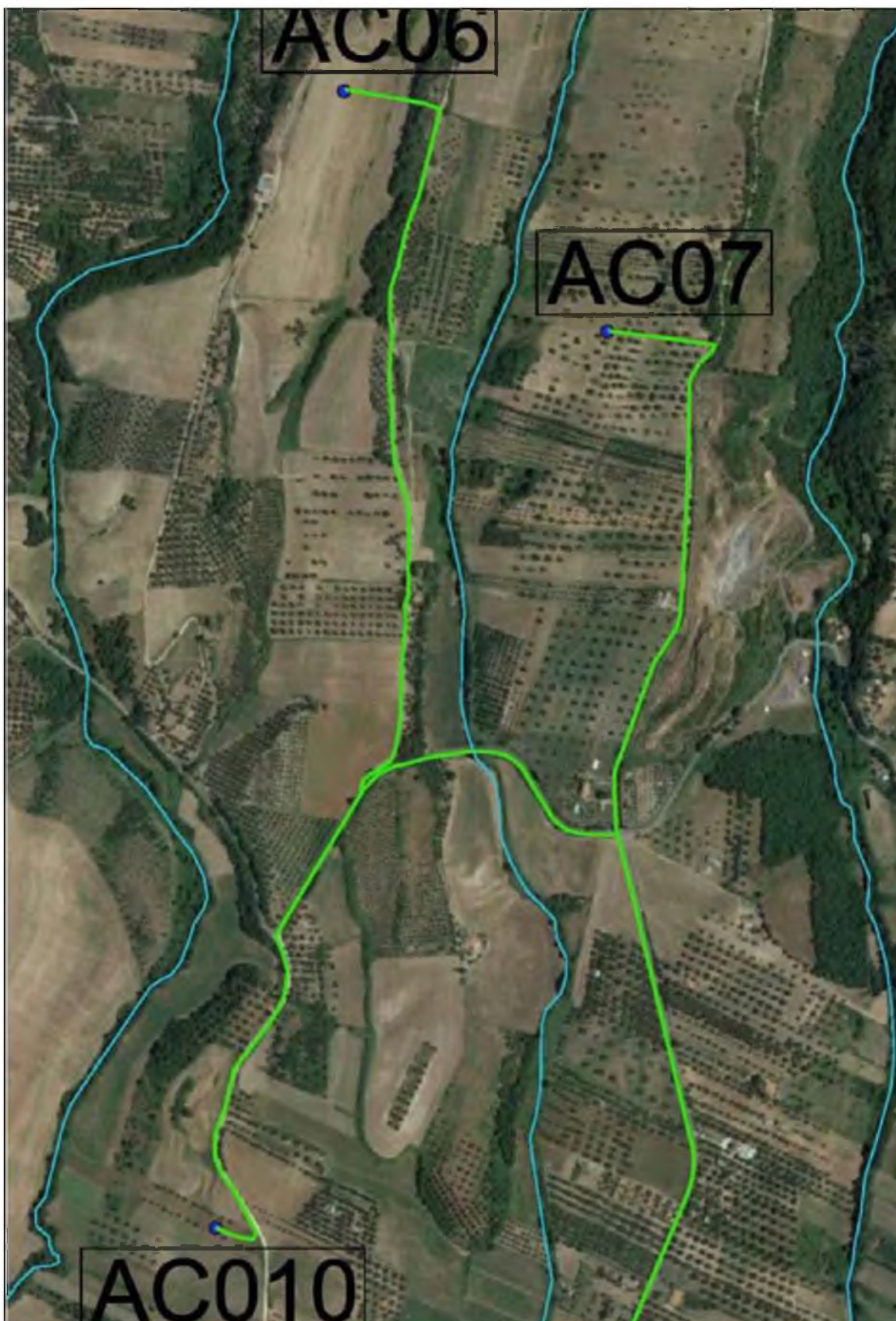
Figura 52 Intersezione del cavidotto con il reticolo idrografico so ortofoto (WTG AC06 – AC07 – AC10)
