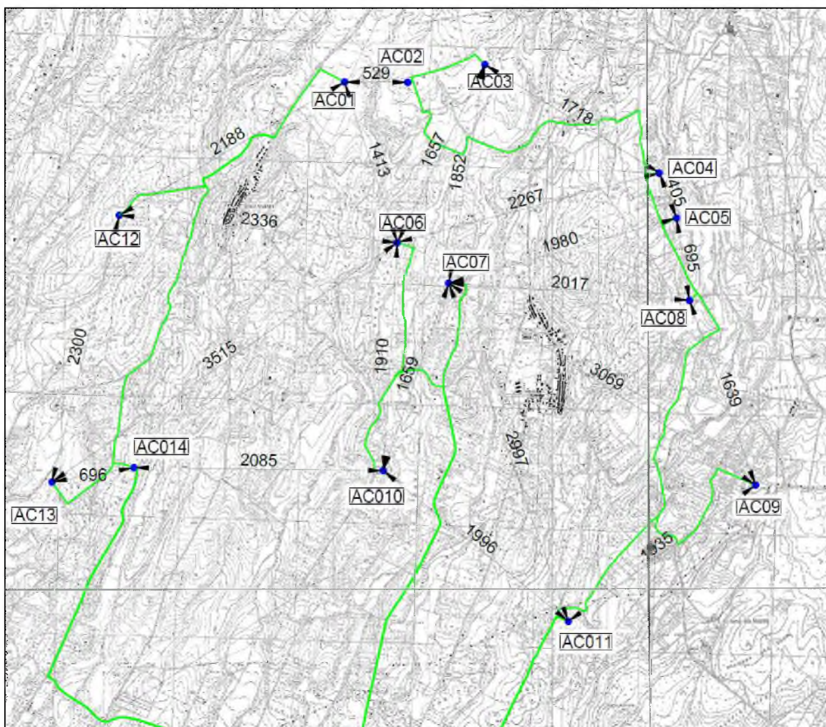
Figura 55 Distanze reciproche tra gli aerogeneratori in progetto
