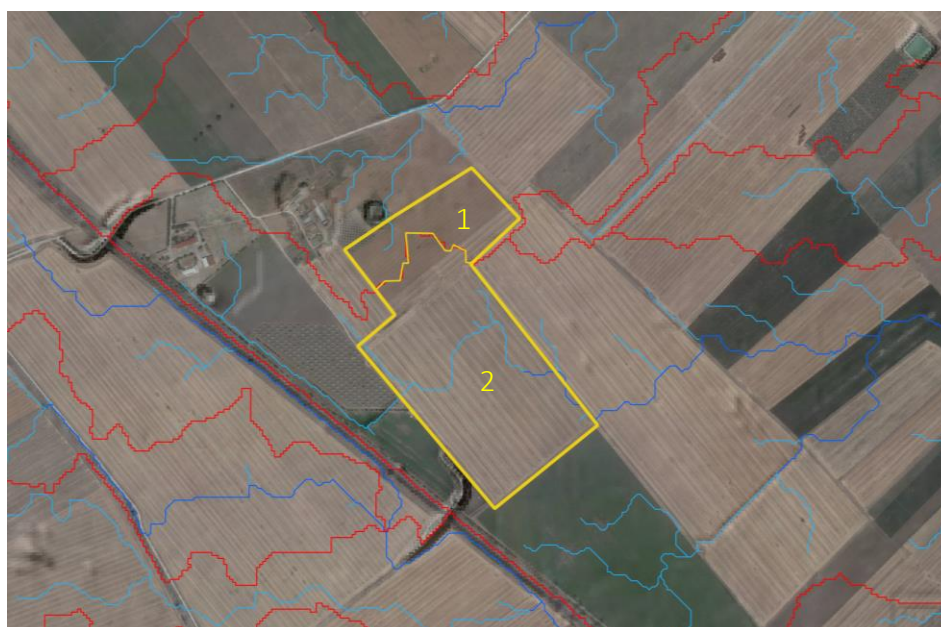
Figura 5.9: Delimitazione recinzione di impianto (giallo), rete di drenaggio naturale interna (blu) e spartiacque (rosso).
