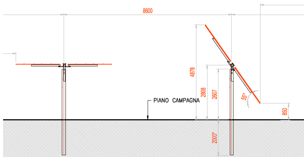
Figura 4.1: Particolare strutture di sostegno moduli, sezione trasversale.
