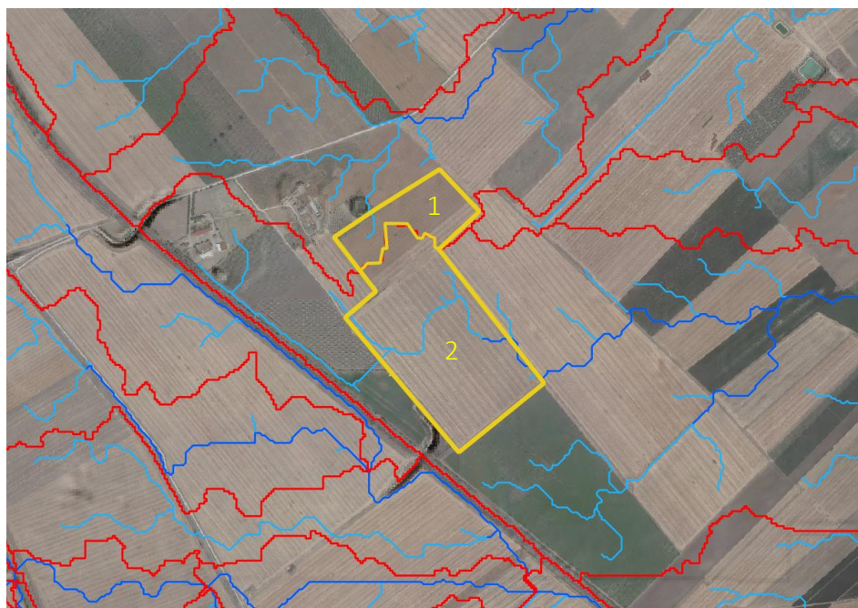
Figura 5.5: Delimitazione bacini scolanti e codifica (giallo), reticolo di drenaggio esterno ed interno alle sezioni di progetto (blu) e limiti bacini idrografici (rosso).
