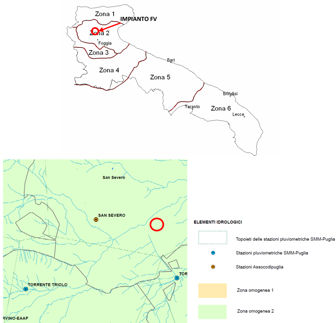
Figura 5.3: Sottostazioni pluviometriche omogenee (Zona 2) e area di progetto (rosso).
