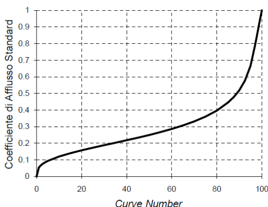
Figura 5.7: Correlazione da letteratura SCS-CN vs. coeff. afflusso/deflusso.
