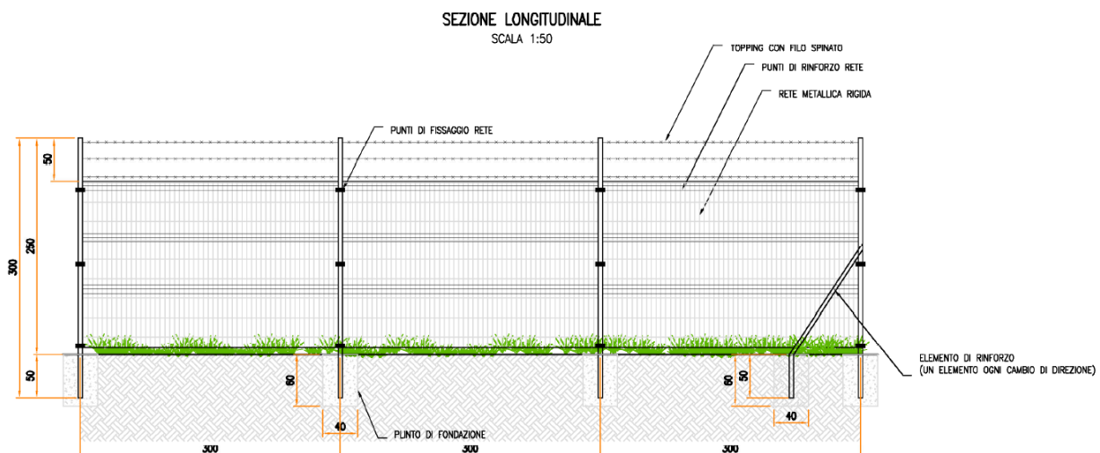
Figura 5.1: Tipico recinzione
