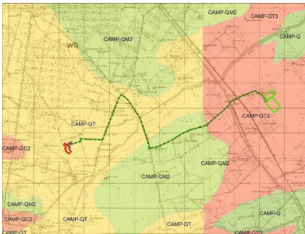
Fig. 5. Le opere in progetto in relazione alla Carta Geologica d'Italia su base IGM 1954.
