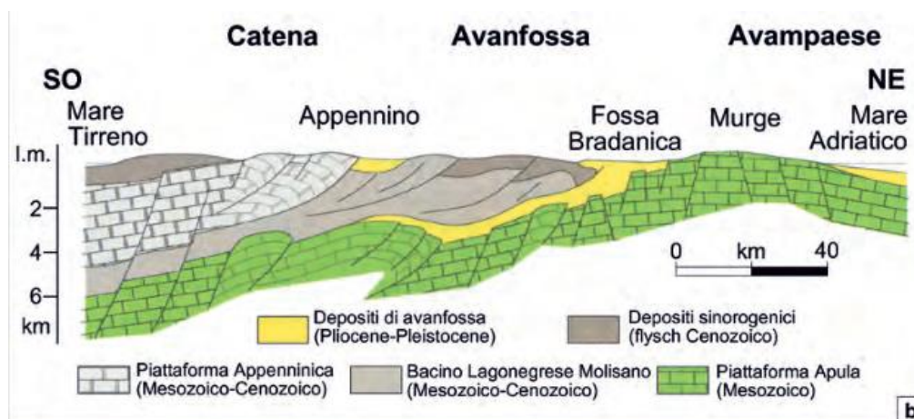
Figura 3.2: Sezione geologica schematica attraverso l'avanfossa appenninica.
