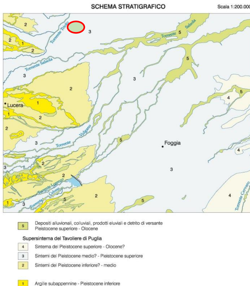
Figura 3.5: Schema stratigrafico.
