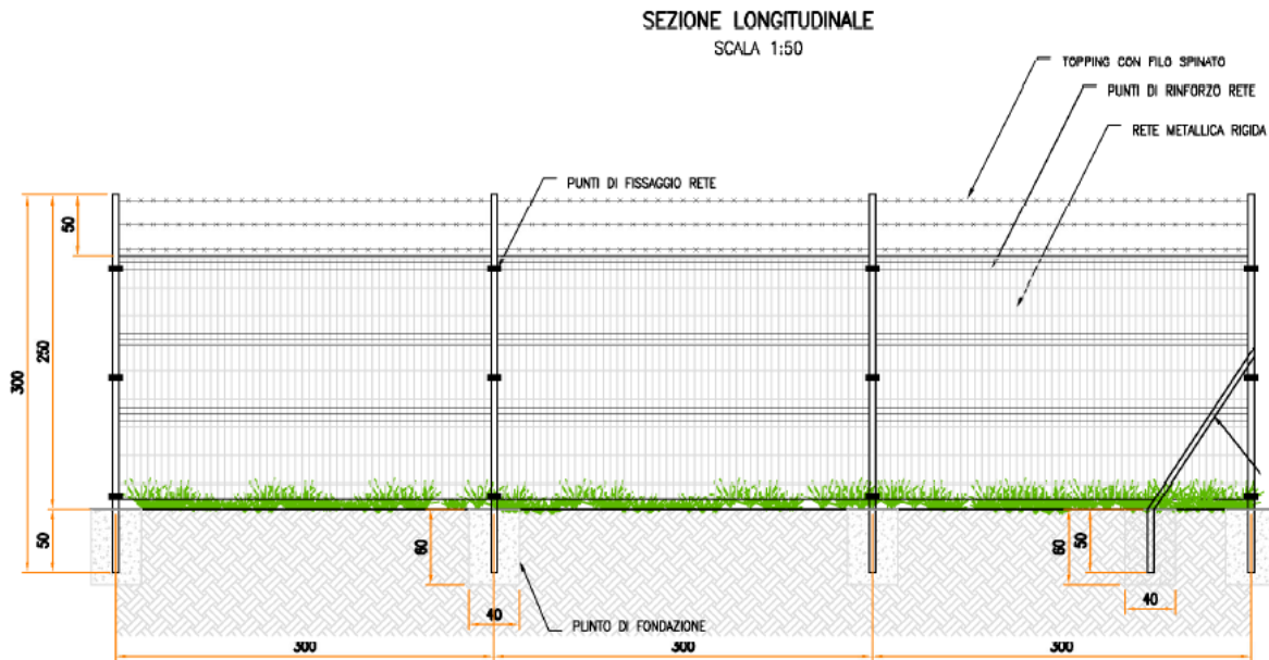
Figura 2.9: Particolare recinzione
