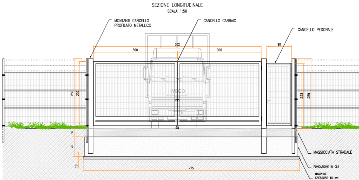
Figura 2.11: Particolare accesso
