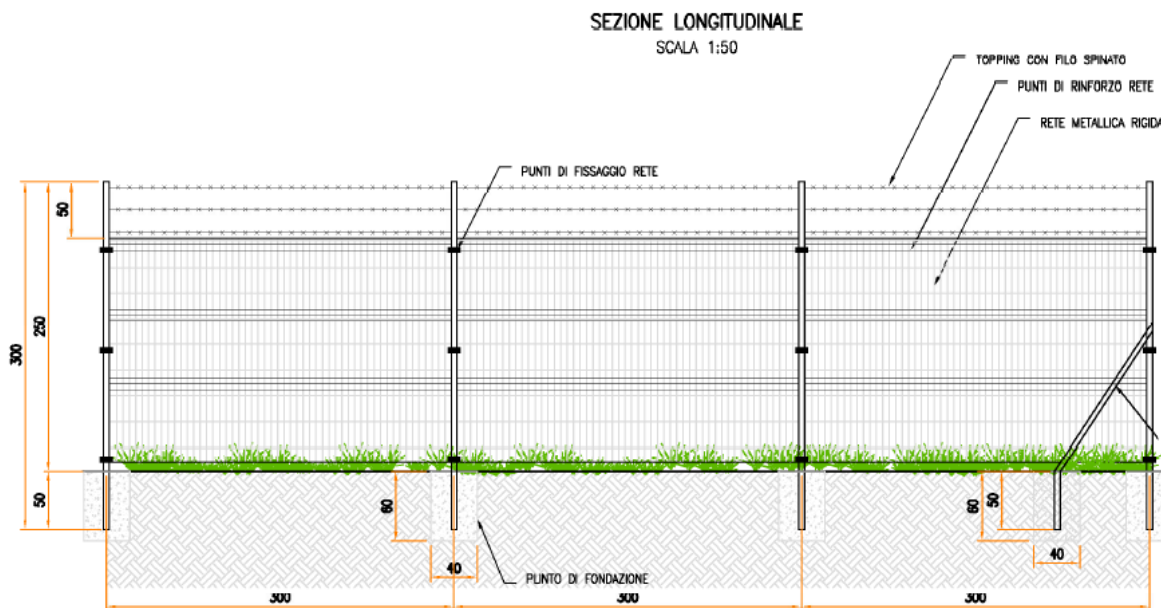
Figura 2.9: Particolare recinzione
