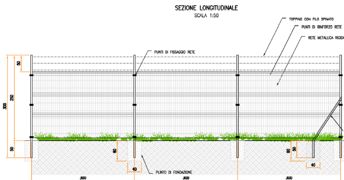
Figura 2.44: Particolare recinzione
