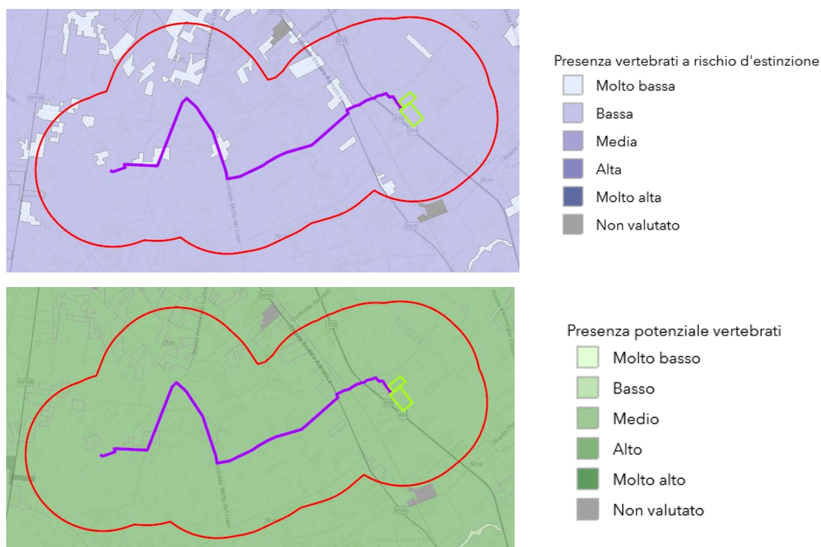
Figura 4.24: Indicatore di presenza effettiva di Vertebrati a rischio di estinzione e presenza potenziale di specie di Vertebrati nell'area di studio (fonte: ISPRA Dati del Sistema Informativo di Carta della Natura)
