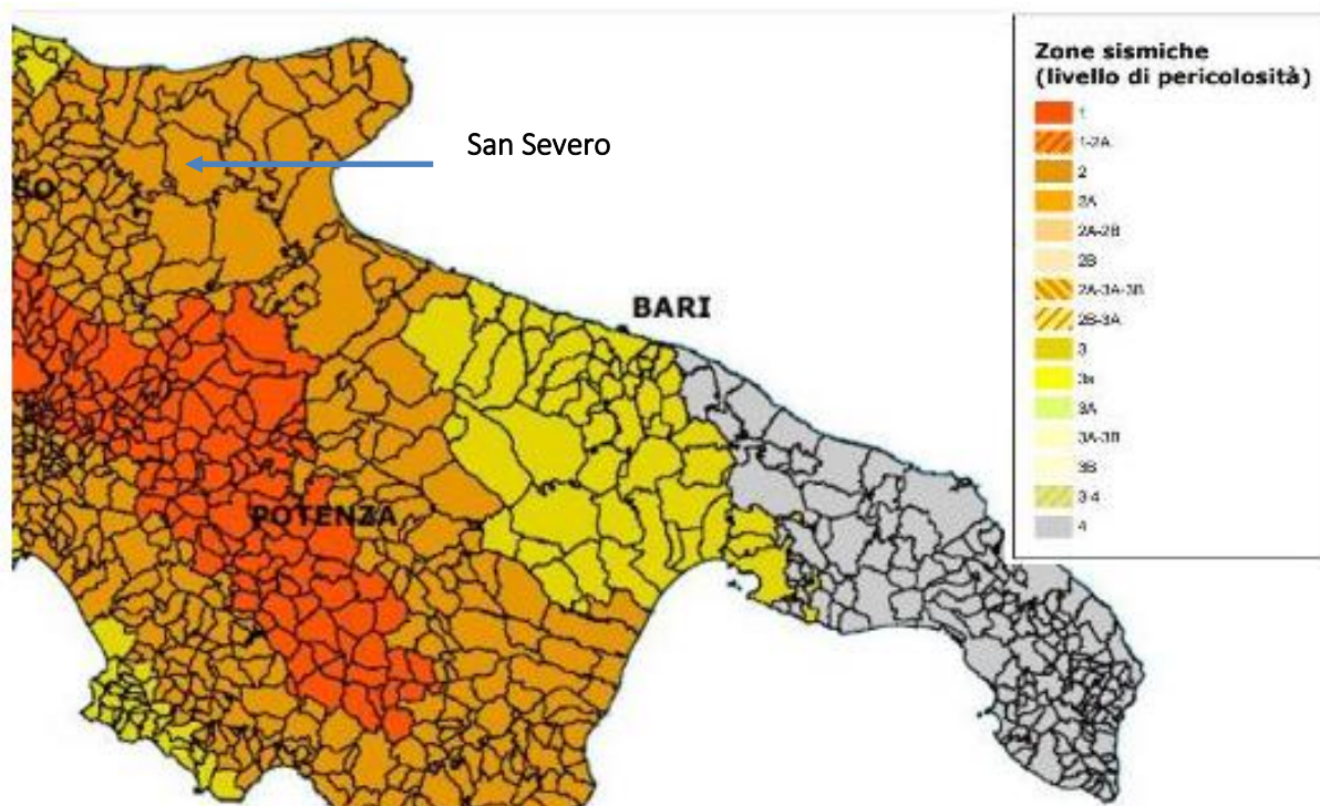
Figura 4.39 – Classificazione sismica del gennaio 2019.
