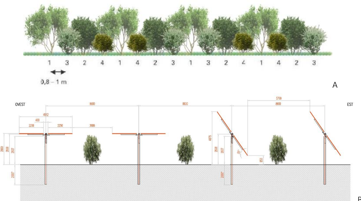
Figura 2.60:A – Tipologico filare di mitigazione; B - Tipologico dell'impianto Olivicolo
