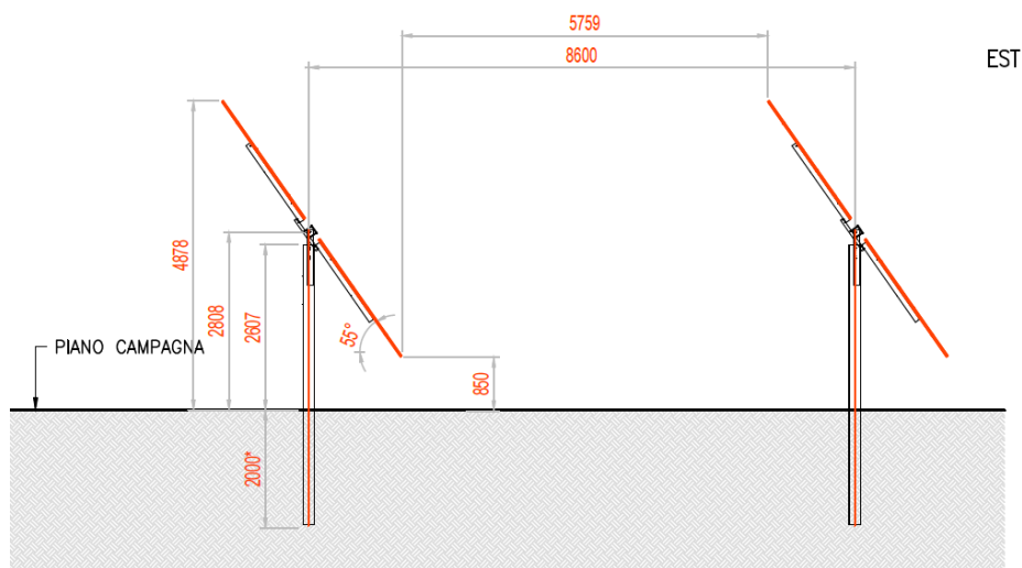
Figura 2.42: Particolare strutture di sostegno moduli.
