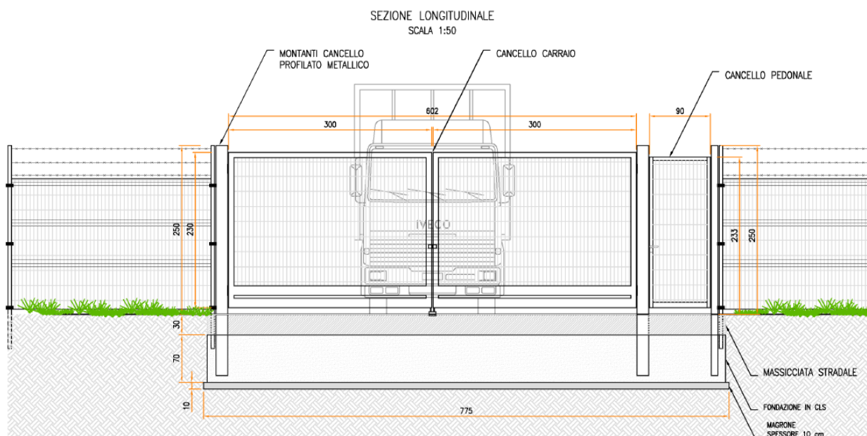
Figura 2.46: Particolare accesso
