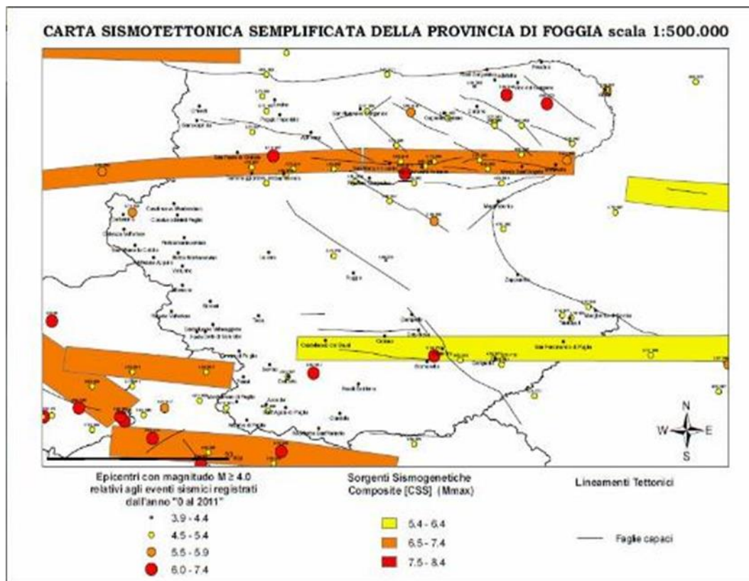
Figura 4.41 – Carta sismotettonica della Provincia di Foggia
