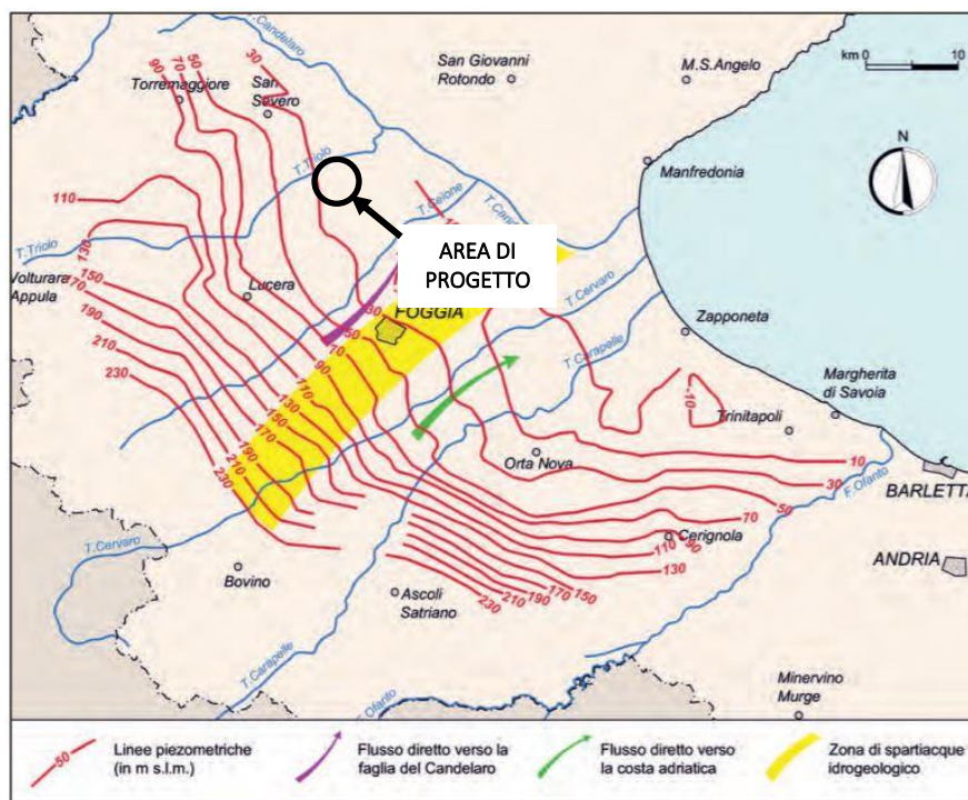
Figura 4.38: Isopieziche della falda superficiale del Tavoliere relativa all'anno 2003 con indicazione delle zone ove è ubicato lo spartiacque idrogeologico (fonte ISPRA), insieme all'area di progetto.
