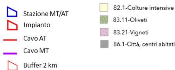
Figura 4.19: Carta degli Habitat, estratto sull'area di progetto (buffer 2 km). Fonte: ISPRA Dati del Sistema Informativo di Carta della Natura
