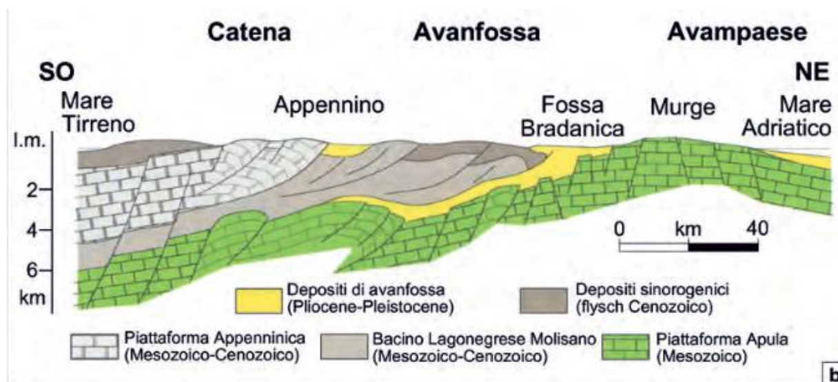
Figura 4.34: Sezione geologica schematica attraverso l'avanfossa appenninica.
