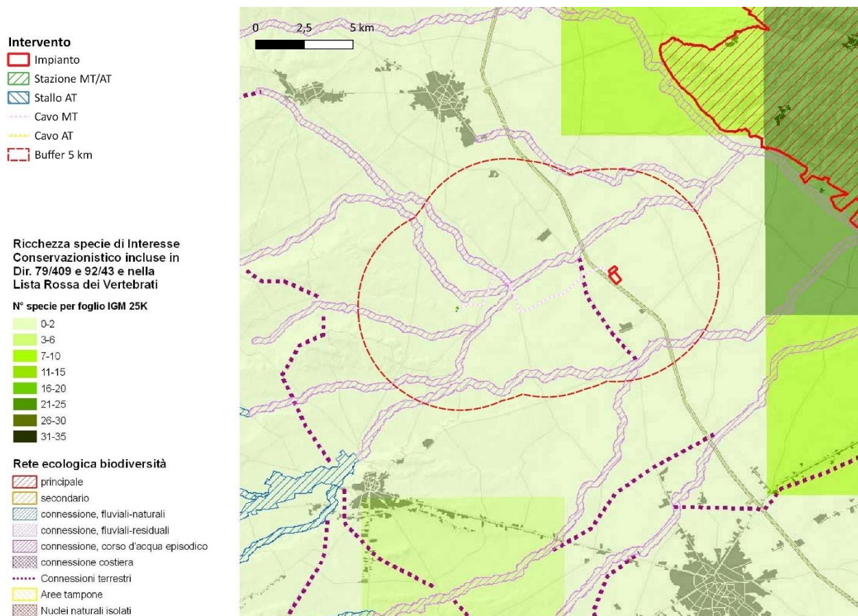
Figura 4.25: Ricchezza di specie di Vertebrati di interesse conservazionistico in Regione Puglia, dettaglio sull'area di studio – fonte: tavole PPTR Regione Puglia
