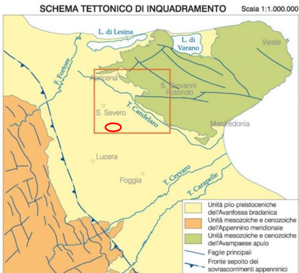
Figura 4.33: Schema geologico e strutturale dell'area del Tavoliere e del Subappennino Dauno – Area di cantiere nel cerchio rosso
