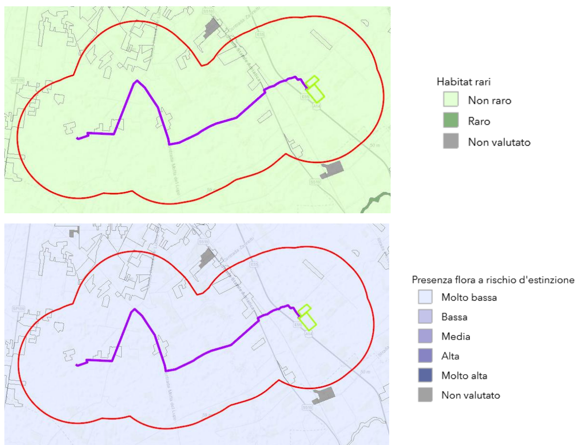
Figura 4.23: Habitat rari e presenza potenziale di flora a rischio di estinzione nell'area di studio (fonte: ISPRA Dati del Sistema Informativo di Carta della Natura)
