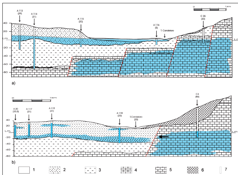
Figura 4.37: Sezioni idrogeologiche. Legenda 1) Depositi d'alveo (Olocene); 2) depositi della pianura alluvionale (Olocene – Pleistocene sup.); 3) argille grigio- azzurrognole con intercalazioni sabbiose (Pleistocene inf. – Pliocene sup.) 4) Calcarene (Pliocene sup. – Miocene); calcari della piattaforma carbonatica apula (Cretaceo); 6) Conoidi detritiche (Olocene – Pleistocene sup.) 7) Pozzo (in tratteggio, se proiettato).
