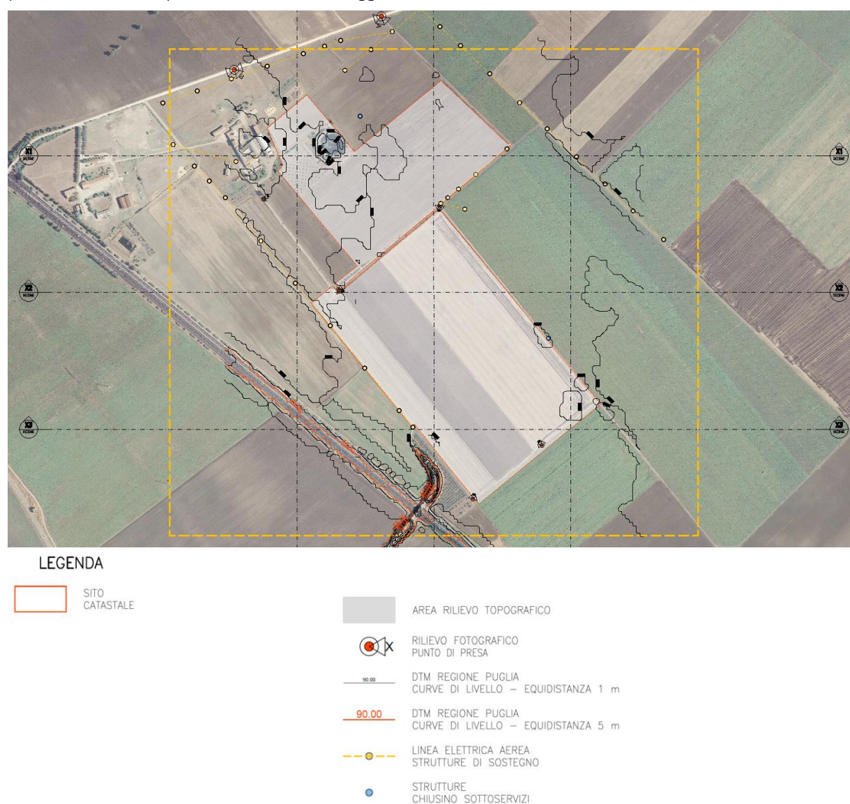
Figura 2.2: Stato di fatto dell'area di progetto
