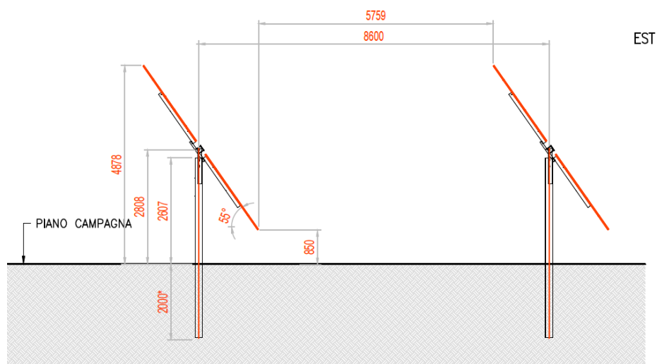
Figura 2.7: Particolare strutture di sostegno moduli.
