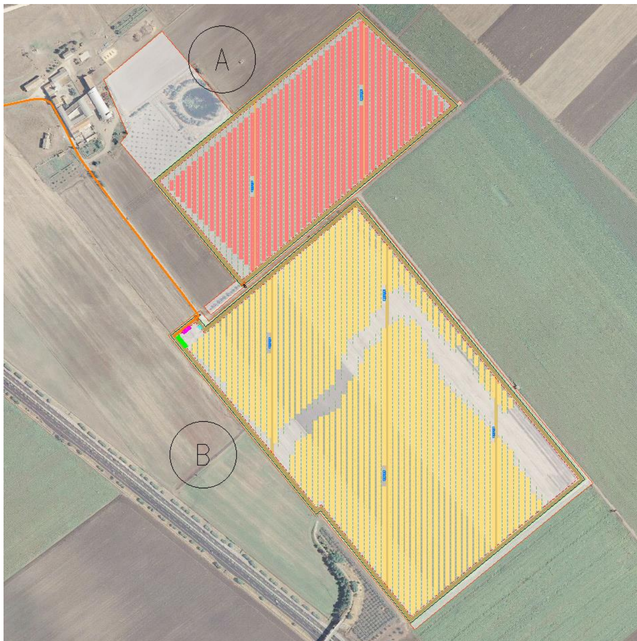
Figura 2.4: Layout di progetto
