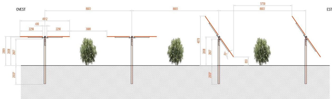
Figura 2.15: Tipologico – Vista Planimetrica dell'impianto Olivicolo
