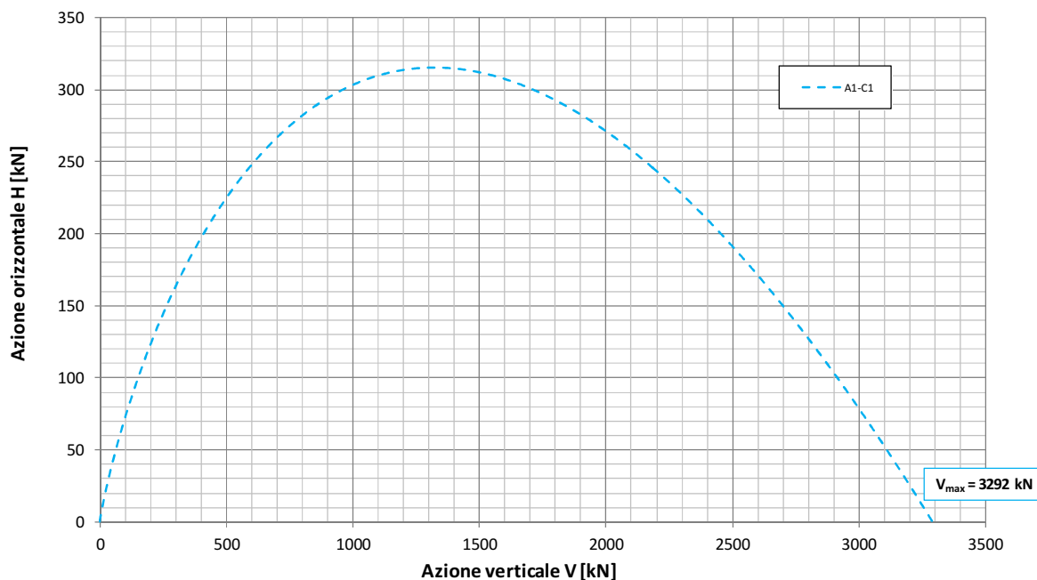
Fondazione B=7.8m - Approfondimento D=7.35m Condizione Sismica - Approccio 1 - Combinazione 1 - A1-M1-R1 Dominio di interazione nel piano V-H ( Brinch Hansen, 1970 )
