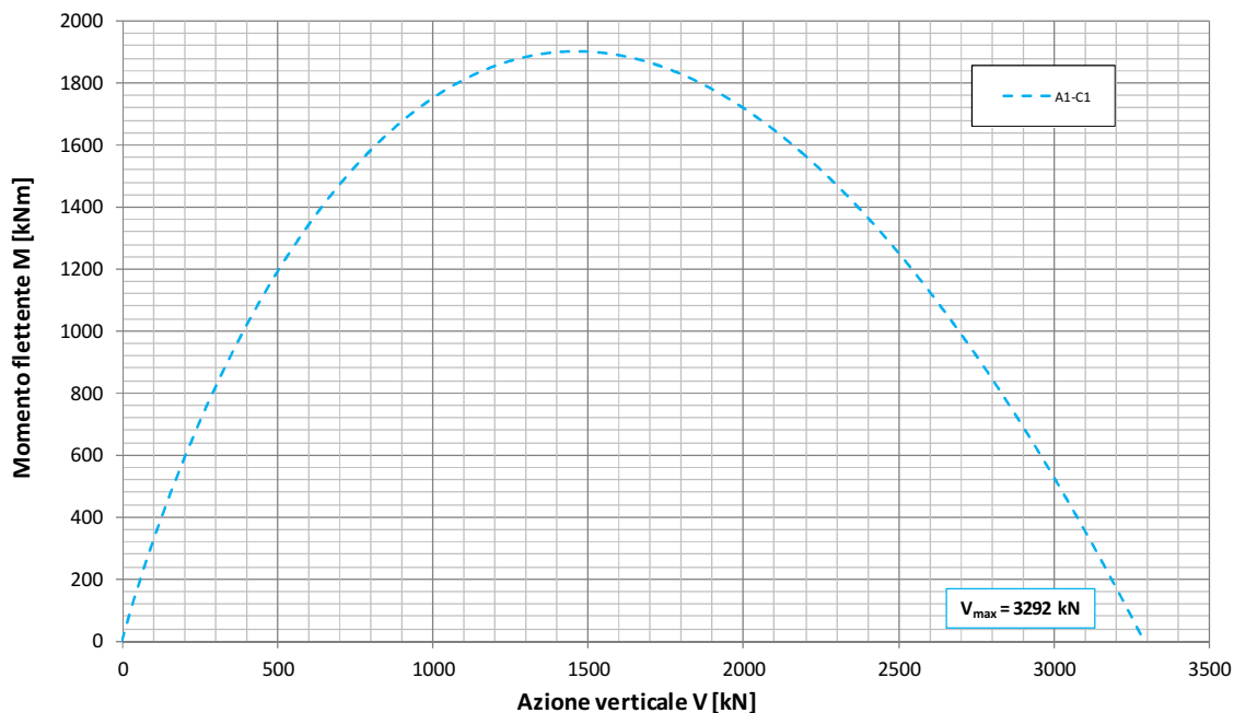
Fondazione B=7.8m - Approfondimento D=7.35m Condizione Sismica - Approccio 1 - Combinazione 1 - A1-M1-R1 Dominio di interazione nel piano V-M ( Meyerhof, 1953 )
