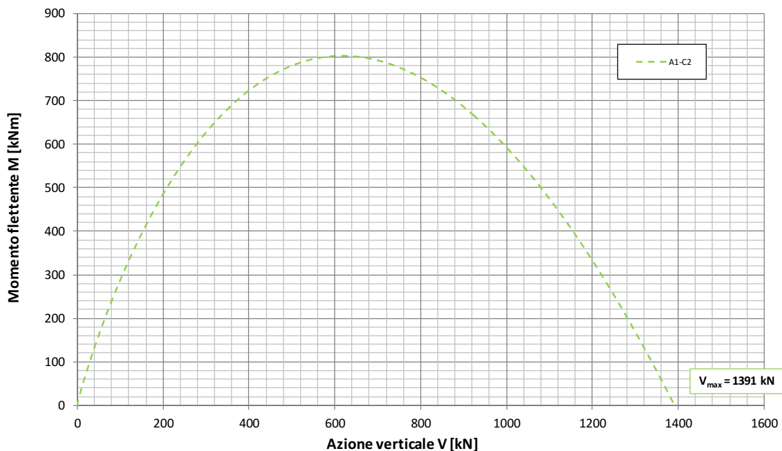
Fondazione B=7.8m - Approfondimento D=7.35m Condizione Sismica - Approccio 1 - Combinazione 2 - A2-M2-R2 Dominio di interazione nel piano V-M ( Meyerhof, 1953 )
