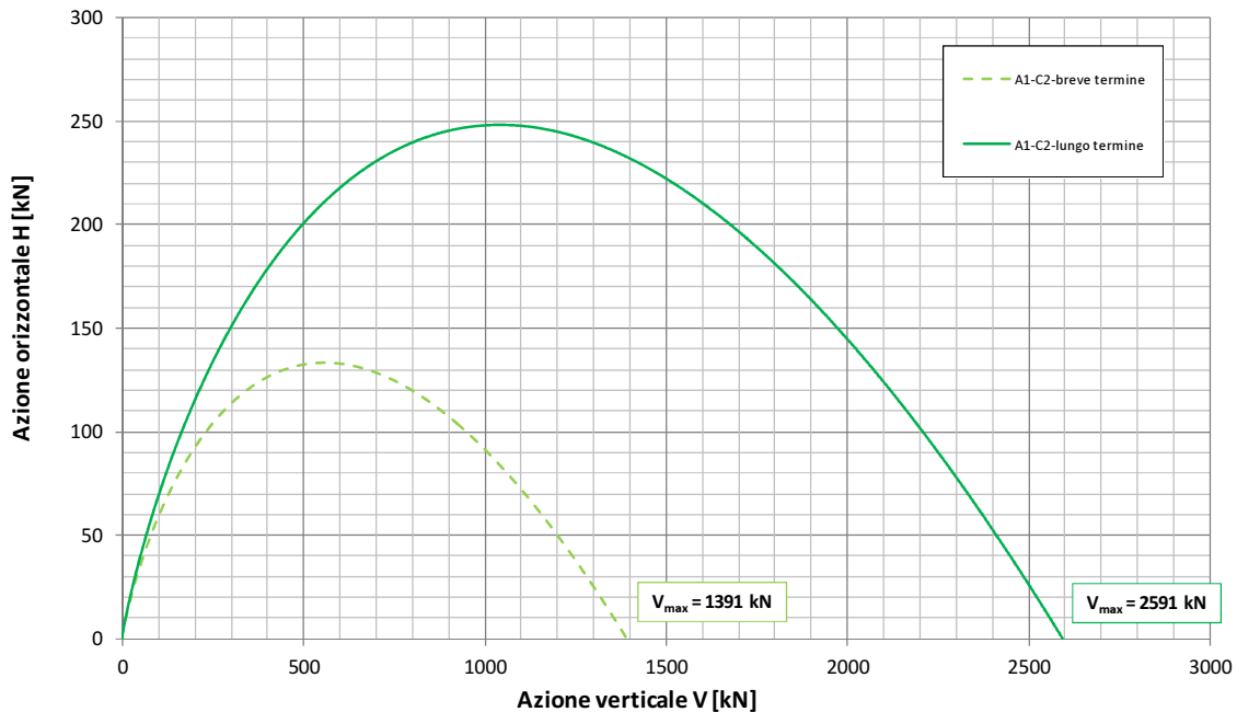
Fondazione B=7.8m - Approfondimento D=7.35m Condizione Statica - Approccio 1 - Combinazione 2 - A2-M2-R2 Dominio di interazione nel piano V-H ( Brinch Hansen, 1970 )
