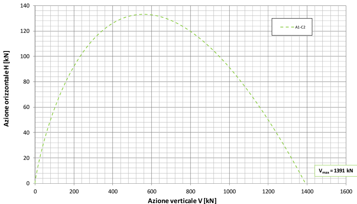
Fondazione B=7.8m - Approfondimento D=7.35m Condizione Sismica - Approccio 1 - Combinazione 2 - A2-M2-R2 Dominio di interazione nel piano V-H ( Brinch Hansen, 1970 )
