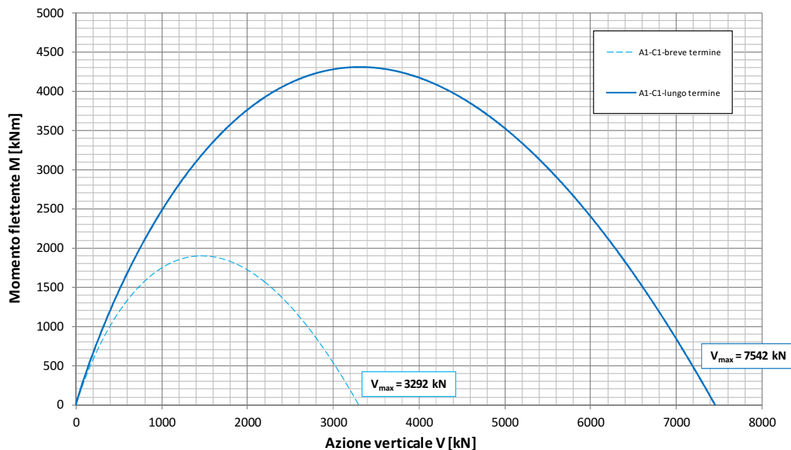
Fondazione B=7.8m - Approfondimento D=7.35m Condizione Statica - Approccio 1 - Combinazione 1 - A1-M1-R1 Dominio di interazione nel piano V-M ( Meyerhof, 1953 )
