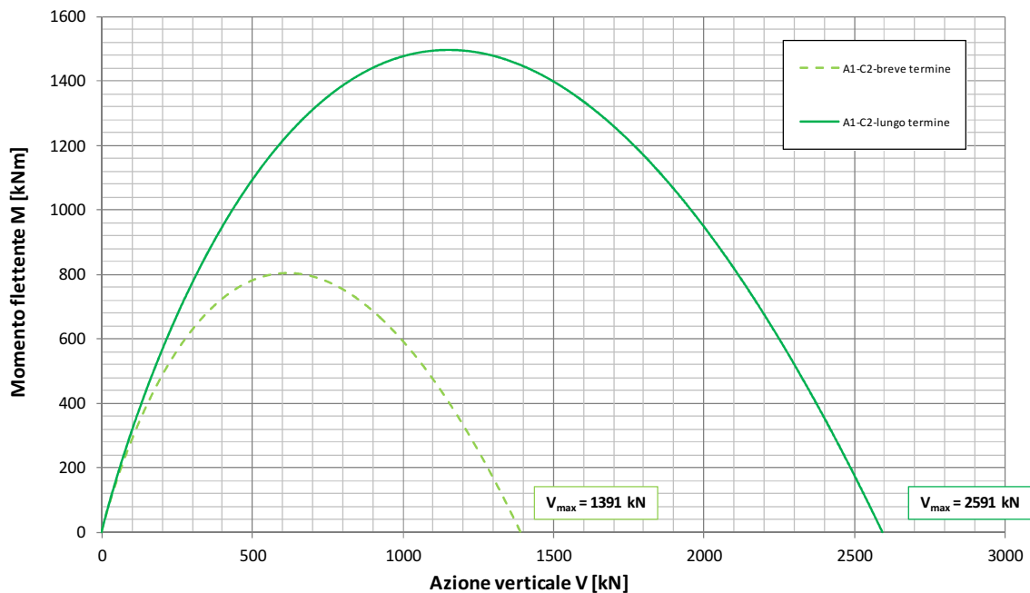
Fondazione B=7.8m - Approfondimento D=7.35m Condizione Statica - Approccio 1 - Combinazione 2 - A2-M2-R2 Dominio di interazione nel piano V-M ( Meyerhof, 1953 )
