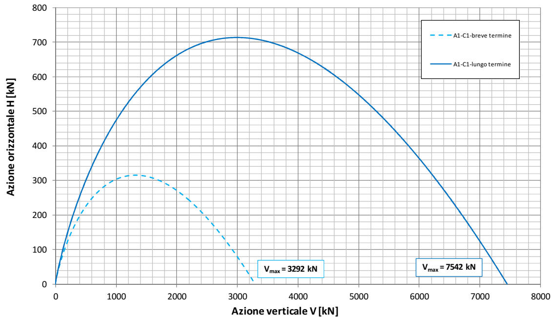
Fondazione B=7.8m - Approfondimento D=7.35m Condizione Statica - Approccio 1 - Combinazione 1 - A1-M1-R1 Dominio di interazione nel piano V-H ( Brinch Hansen, 1970 )
