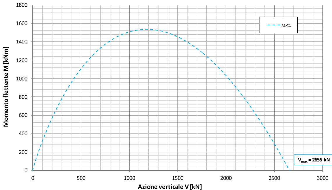
Fondazione B=7.8m - Approfondimento D=1.10m Condizione Sismica - Approccio 1 - Combinazione 1 - A1-M1-R1 Dominio di interazione nel piano V-M ( Meyerhof, 1953 )
