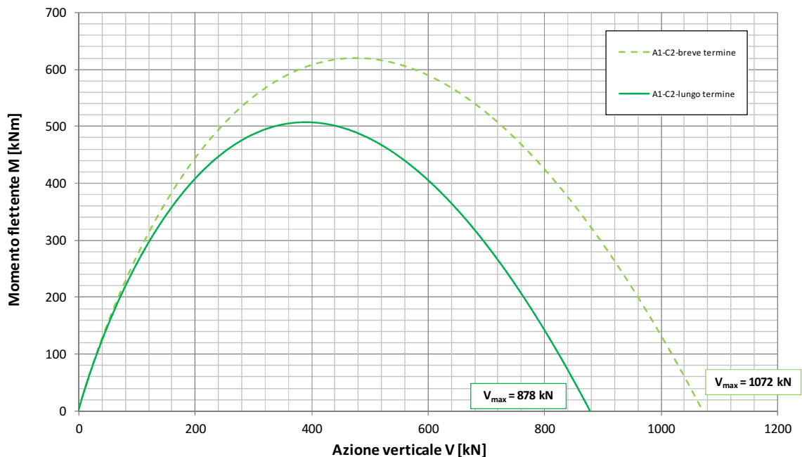
Fondazione B=7.8m - Approfondimento D=1.10m Condizione Statica - Approccio 1 - Combinazione 2 - A2-M2-R2 Dominio di interazione nel piano V-M ( Meyerhof, 1953 )
