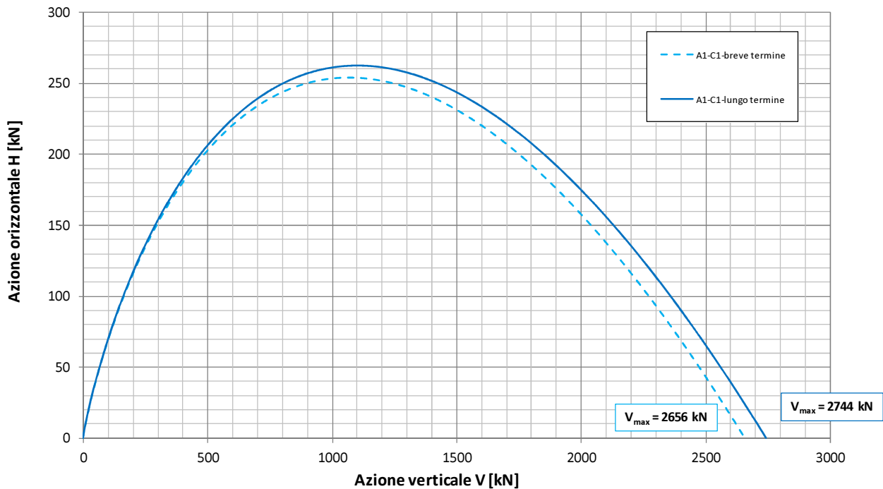
Fondazione B=7.8m - Approfondimento D=1.10m Condizione Statica - Approccio 1 - Combinazione 1 - A1-M1-R1 Dominio di interazione nel piano V-H ( Brinch Hansen, 1970 )
