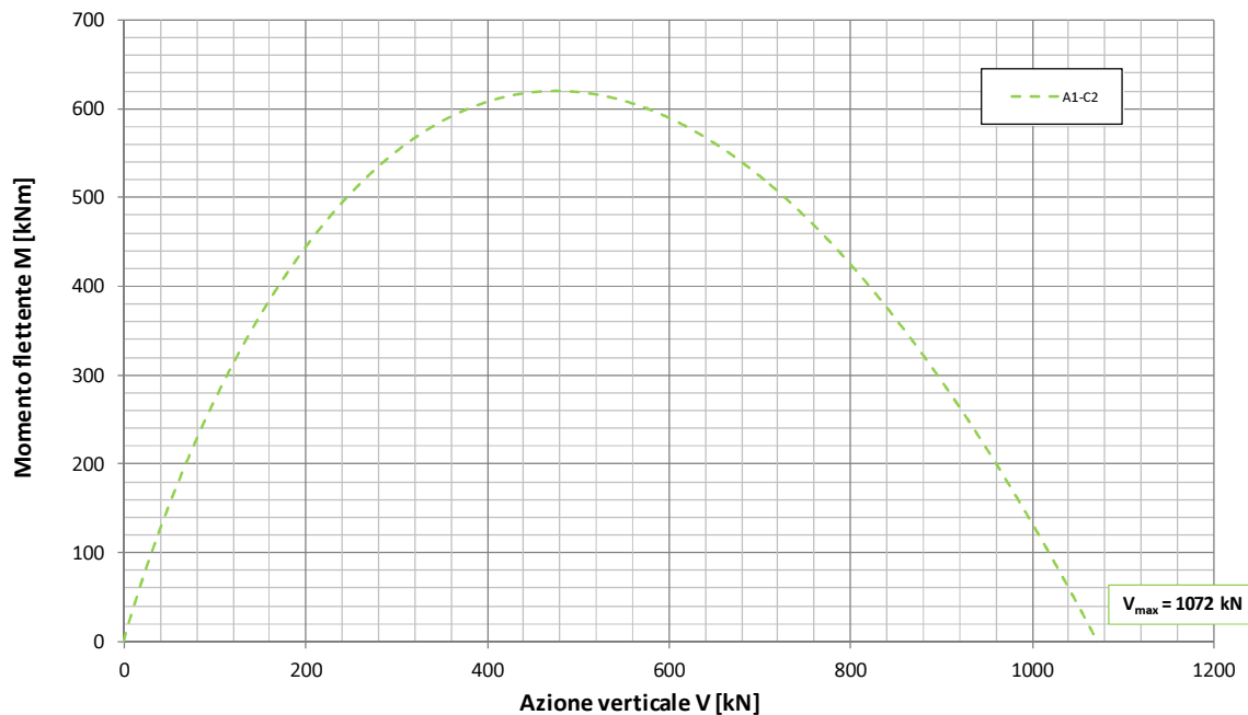
Fondazione B=7.8m - Approfondimento D=1.10m Condizione Sismica - Approccio 1 - Combinazione 2 - A2-M2-R2 Dominio di interazione nel piano V-M ( Meyerhof, 1953 )
