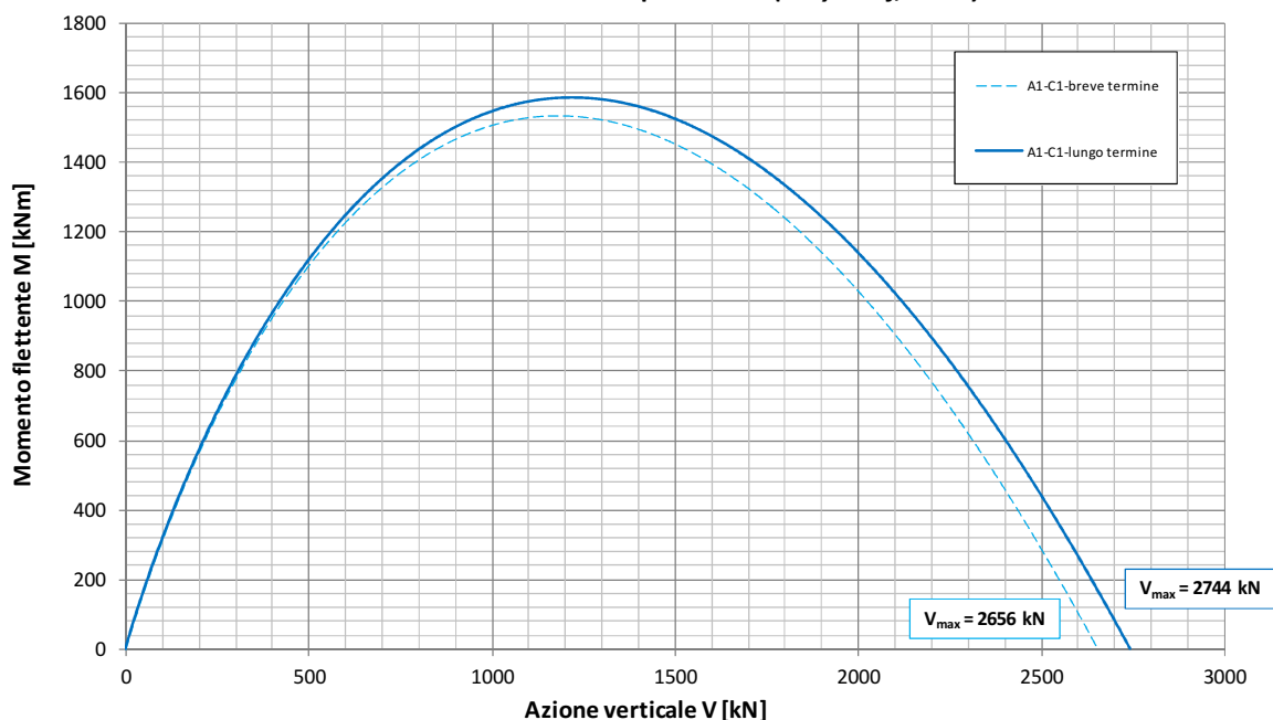
Fondazione B=7.8m - Approfondimento D=1.1m Condizione Statica - Approccio 1 - Combinazione 1 - A1-M1-R1 Dominio di interazione nel piano V-M ( Meyerhof, 1953 )
