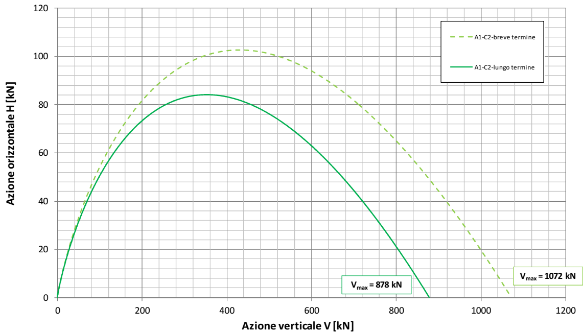
Fondazione B=7.8m - Approfondimento D=1.10m Condizione Statica - Approccio 1 - Combinazione 2 - A2-M2-R2 Dominio di interazione nel piano V-H ( Brinch Hansen, 1970 )
