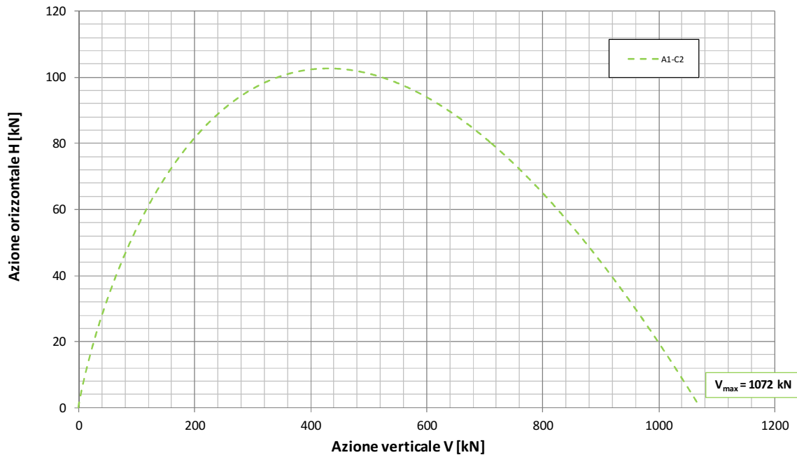
Fondazione B=7.8m - Approfondimento D=1.10m Condizione Sismica - Approccio 1 - Combinazione 2 - A2-M2-R2 Dominio di interazione nel piano V-H ( Brinch Hansen, 1970 )
