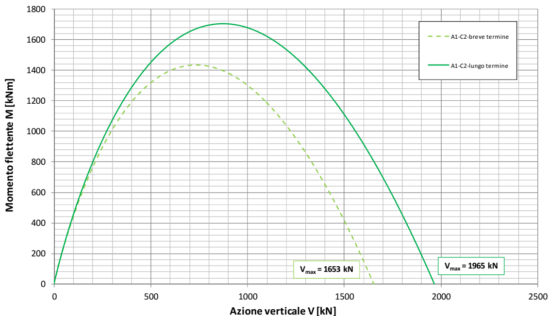
Fondazione B=11.7m - Approfondimento D=1.7m Condizione Statica - Approccio 1 - Combinazione 2 - A2-M2-R2 Dominio di interazione nel piano V-M ( Meyerhof, 1953 )
