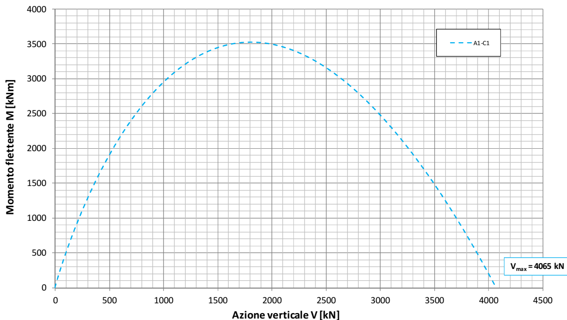
Fondazione B=11.7m - Approfondimento D=1.7m Condizione Sismica - Approccio 1 - Combinazione 1 - A1-M1-R1 Dominio di interazione nel piano V-M ( Meyerhof, 1953 )
