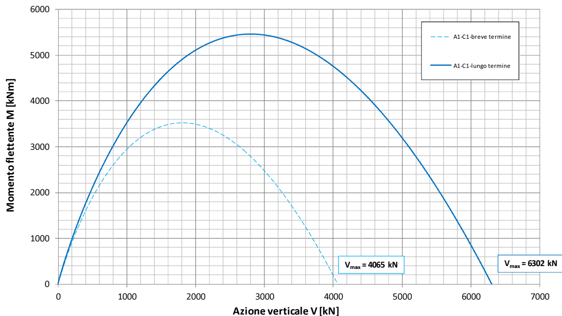
Fondazione B=11.7m - Approfondimento D=1.7m Condizione Statica - Approccio 1 - Combinazione 1 - A1-M1-R1 Dominio di interazione nel piano V-M ( Meyerhof, 1953 )
