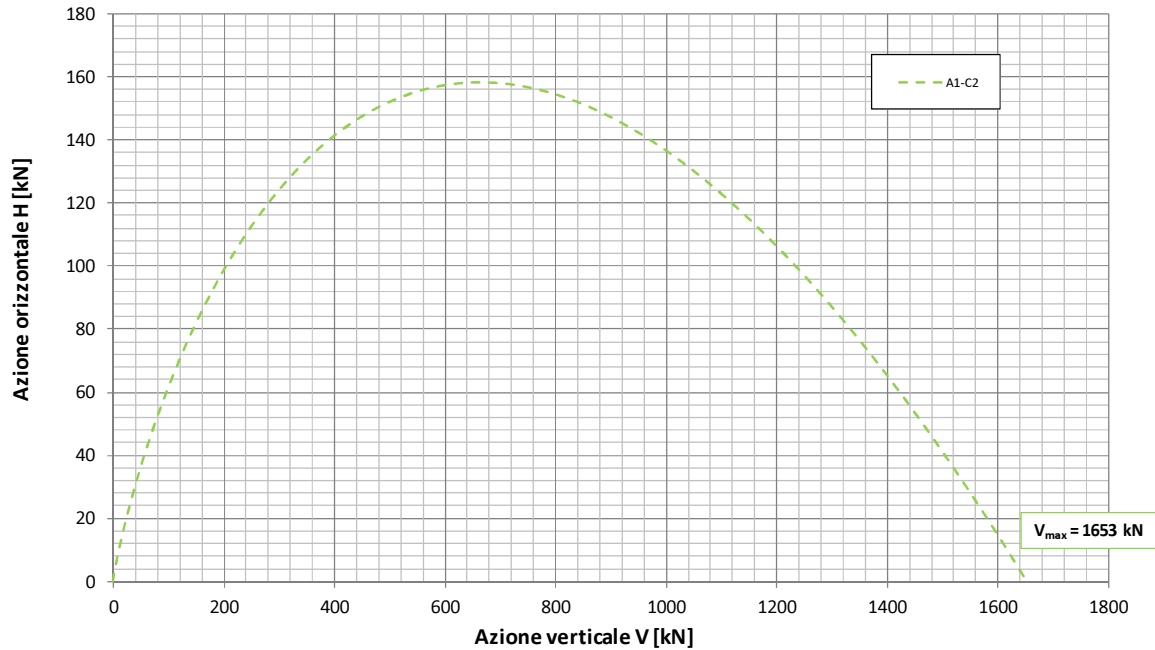
Fondazione B=11.7m - Approfondimento D=1.7m Condizione Sismica - Approccio 1 - Combinazione 2 - A2-M2-R2 Dominio di interazione nel piano V-H ( Brinch Hansen, 1970 )
