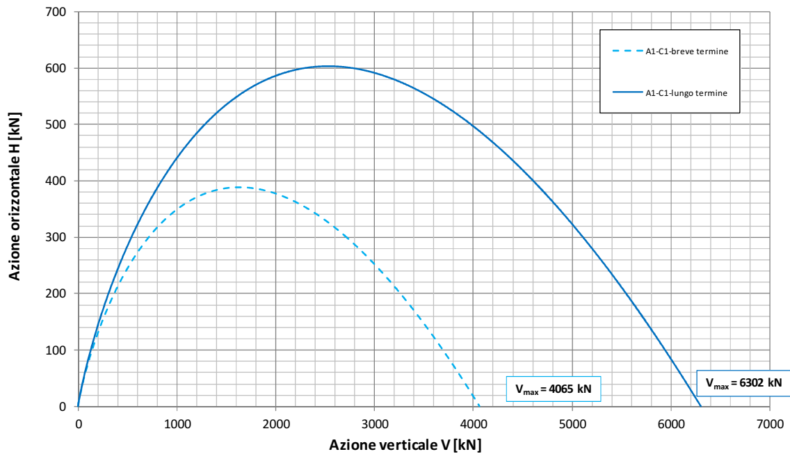
Fondazione B=11.7m - Approfondimento D=1.7m Condizione Statica - Approccio 1 - Combinazione 1 - A1-M1-R1 Dominio di interazione nel piano V-H ( Brinch Hansen, 1970 )
