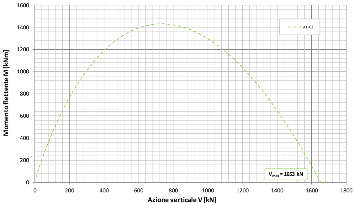
Fondazione B=11.7m - Approfondimento D=1.7m Condizione Sismica - Approccio 1 - Combinazione 2 - A2-M2-R2 Dominio di interazione nel piano V-M ( Meyerhof, 1953 )
