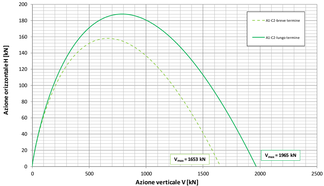
Fondazione B=11.7m - Approfondimento D=1.7m Condizione Statica - Approccio 1 - Combinazione 2 - A2-M2-R2 Dominio di interazione nel piano V-H ( Brinch Hansen, 1970 )
