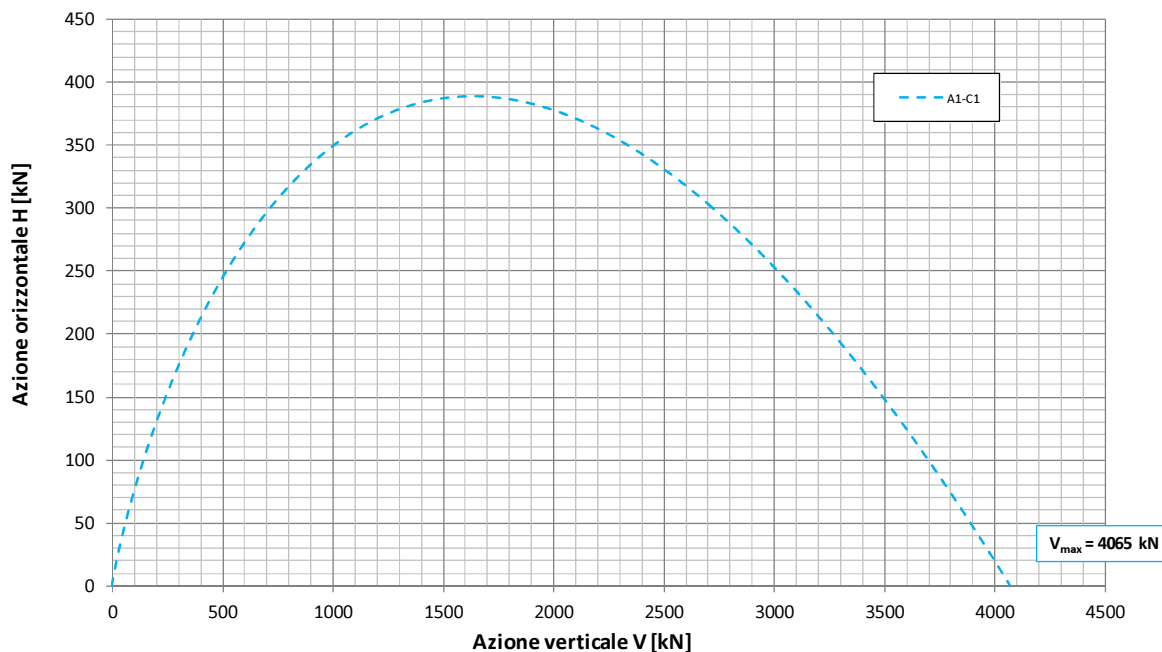
Fondazione B=11.7m - Approfondimento D=1.7m Condizione Sismica - Approccio 1 - Combinazione 1 - A1-M1-R1 Dominio di interazione nel piano V-H ( Brinch Hansen, 1970 )
