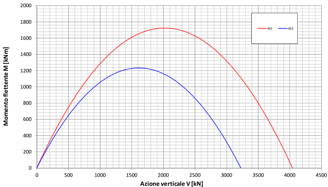
Fondazione B=6.7m - Approfondimento D=9.6m Condizione Statica Non Drenata Dominio di interazione nel piano V-M (Gourvenec, 2007)
