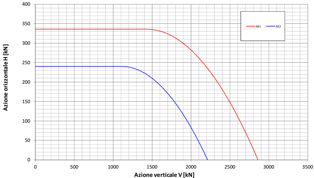
Fondazione B=5.6m - Approfondimento D=5.7m Condizione Statica Non Drenata Dominio di interazione nel piano V-H (Gourvenec, 2007)
