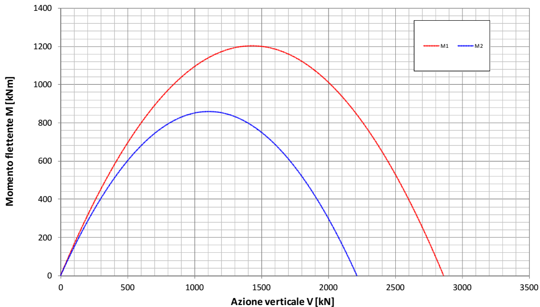
Fondazione B=5.6m - Approfondimento D=5.7m Condizione Statica Non Drenata Dominio di interazione nel piano V-M (Gourvenec, 2007)
