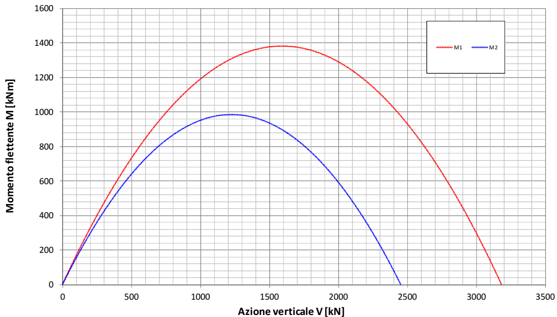
Fondazione B=6.0m - Approfondimento D=5.7m Condizione Sismica Non Drenata Dominio di interazione nel piano V-M (Gourvenec, 2007)
