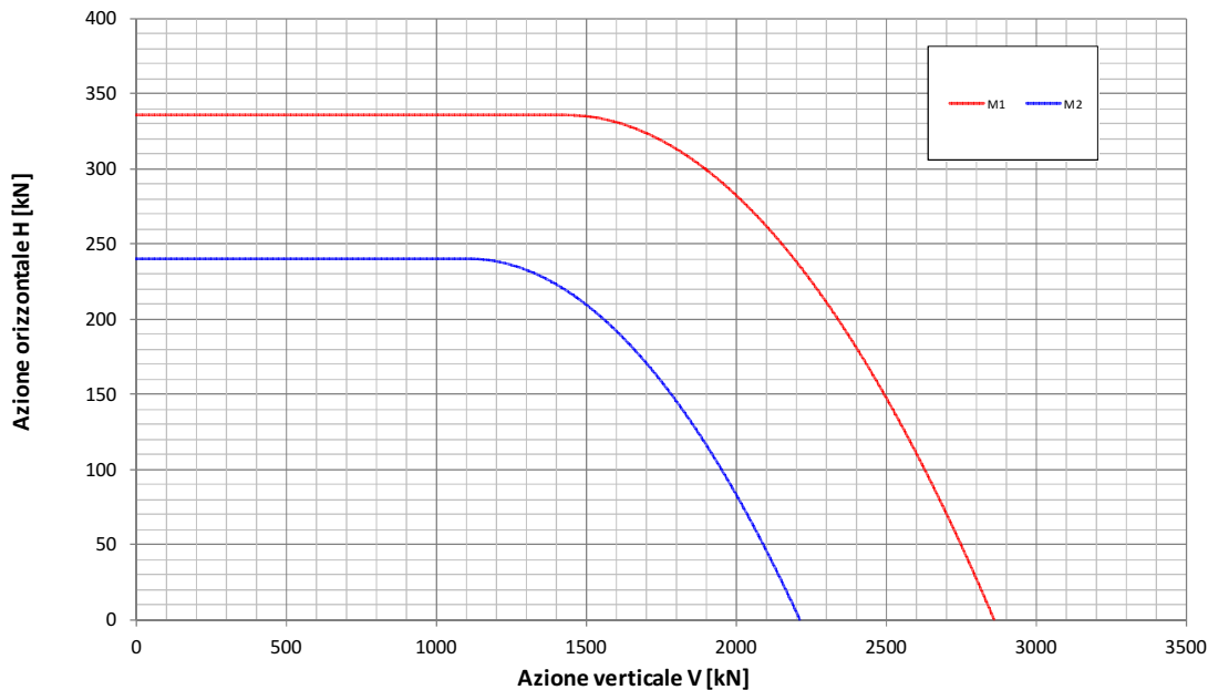
Fondazione B=5.6m - Approfondimento D=5.7m Condizione Sismica Non Drenata Dominio di interazione nel piano V-H ( Gourvenec, 2007 )
