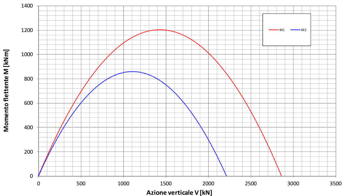
Fondazione B=5.6m - Approfondimento D=5.7m Condizione Sismica Non Drenata Dominio di interazione nel piano V-M ( Gourvenec, 2007 )
