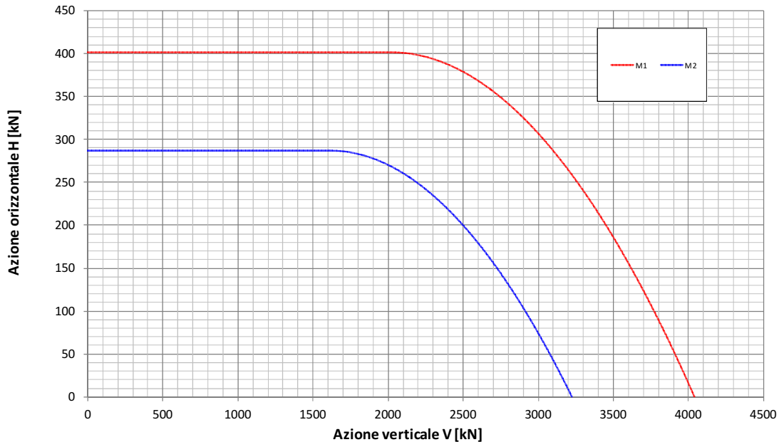
Fondazione B=6.7m - Approfondimento D=9.6m Condizione Sismica Non Drenata Dominio di interazione nel piano V-H (Gourvenec, 2007)
