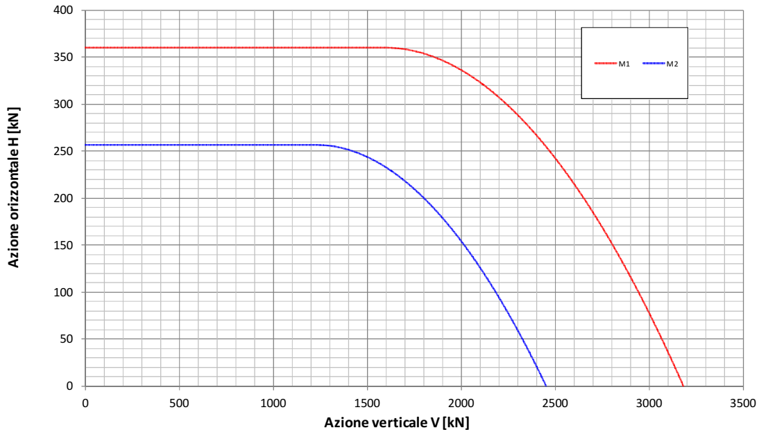
Fondazione B=6.0m - Approfondimento D=5.7m Condizione Sismica Non Drenata Dominio di interazione nel piano V-H (Gourvenec, 2007)
