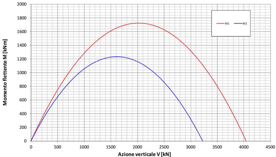
Fondazione B=6.7m - Approfondimento D=9.6m Condizione Sismica Non Drenata Dominio di interazione nel piano V-M (Gourvenec, 2007)
