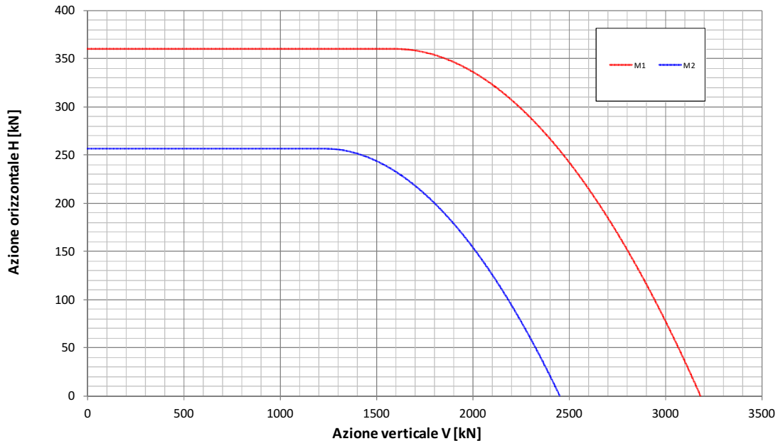
Fondazione B=6.0m - Approfondimento D=5.7m Condizione Statica Non Drenata Dominio di interazione nel piano V-H ( Gourvenec, 2007 )
