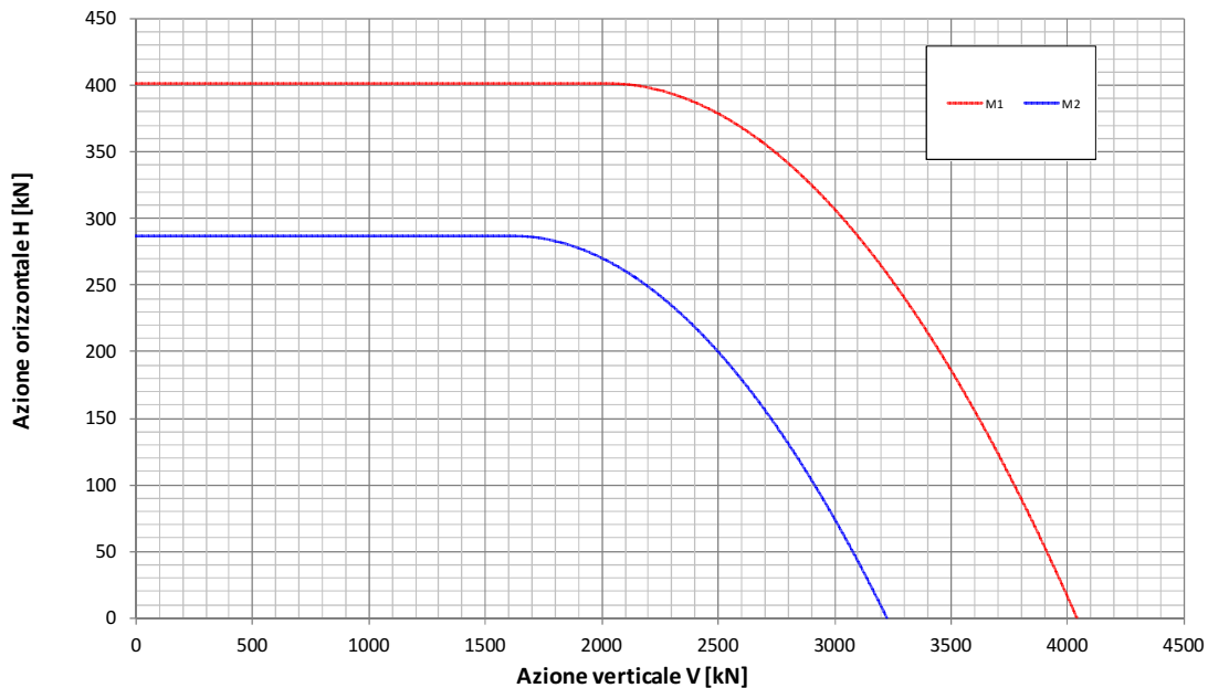
Fondazione B=6.7m - Approfondimento D=9.6m Condizione Statica Non Drenata Dominio di interazione nel piano V-H (Gourvenec, 2007)
