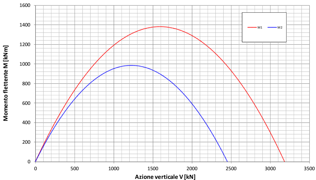
Fondazione B=6.0m - Approfondimento D=5.7m Condizione Statica Non Drenata Dominio di interazione nel piano V-M ( Gourvenec, 2007 )
