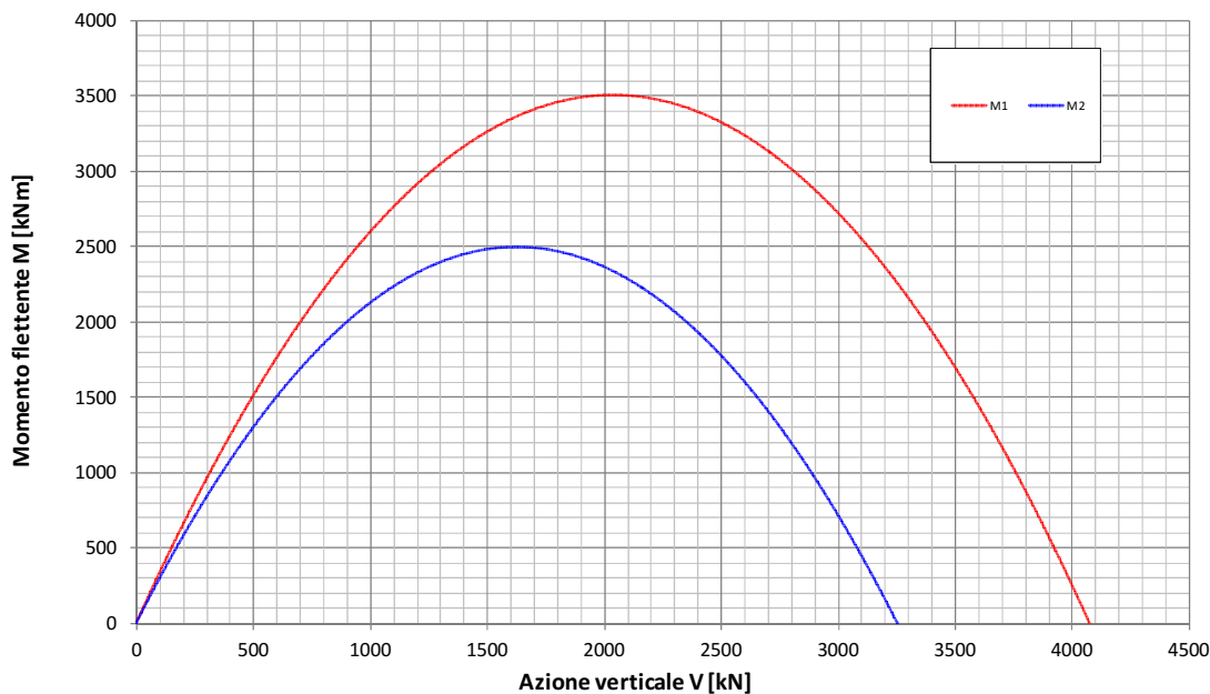
Fondazione B=11.7m - Approfondimento D=5.7m Condizione Statica Non Drenata Dominio di interazione nel piano V-M ( Gourvenec, 2007 )
