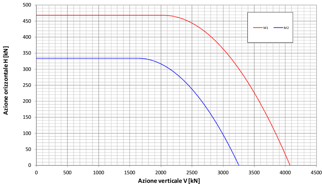
Fondazione B=11.7m - Approfondimento D=5.7m Condizione Statica Non Drenata Dominio di interazione nel piano V-H ( Gourvenec, 2007 )
