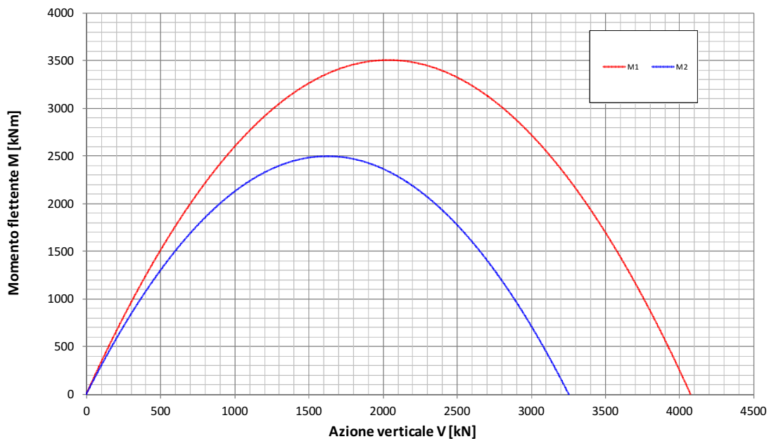
Fondazione B=11.7m - Approfondimento D=5.7m Condizione Sismica Non Drenata Dominio di interazione nel piano V-M ( Gourvenec, 2007 )
