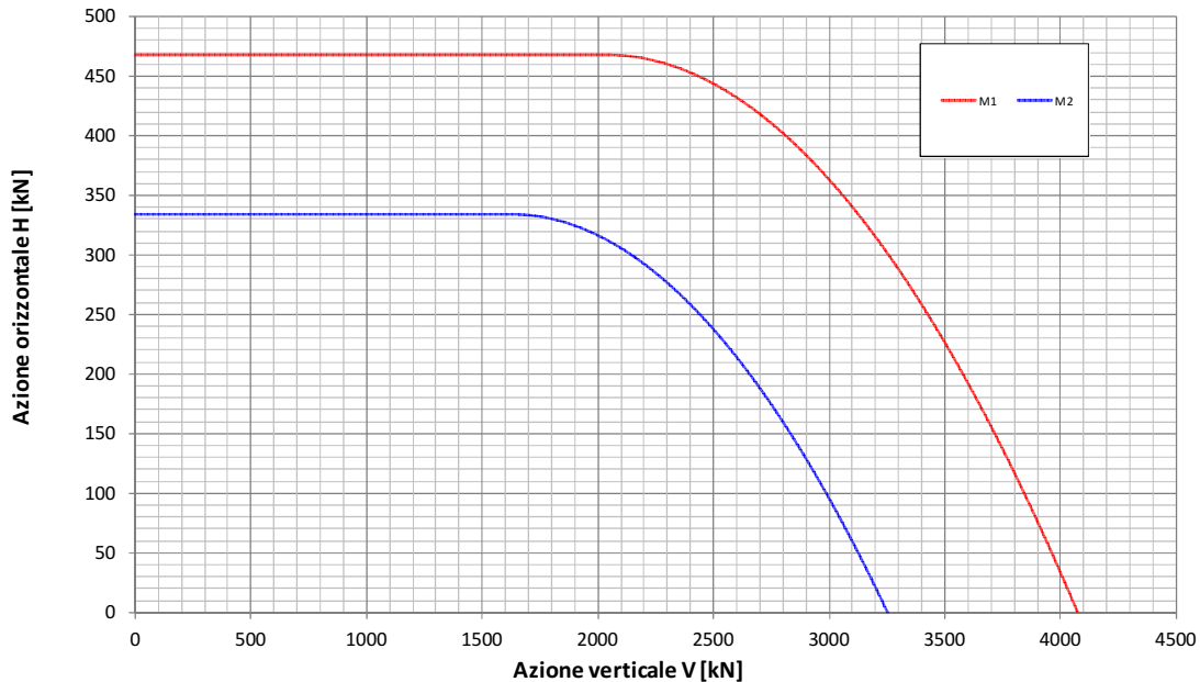
Fondazione B=11.7m - Approfondimento D=5.7m Condizione Sismica Non Drenata Dominio di interazione nel piano V-H ( Gourvenec, 2007 )
