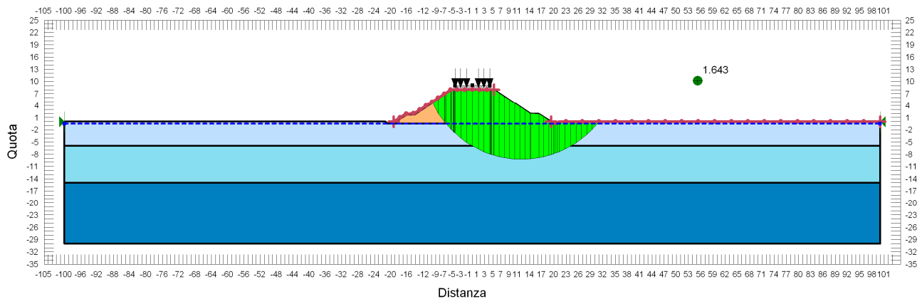
FIGURA 11-8: VERIFICA DI STABILITÀ GLOBALE RILEVATO DI H=8.00 M - CONDIZIONE SISMA-.
