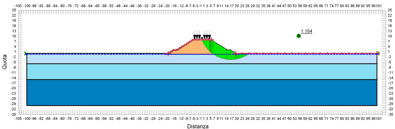
FIGURA 11-6: VERIFICA DI STABILITÀ GLOBALE RILEVATO DI H=8.00 M - CONDIZIONE STATICA DRENATA.
