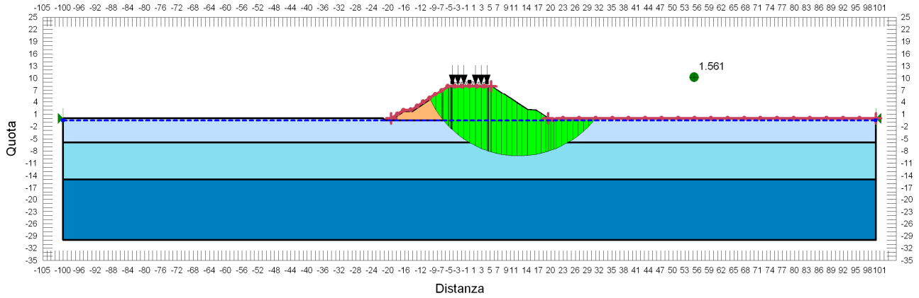
FIGURA 11-7: VERIFICA DI STABILITÀ GLOBALE RILEVATO DI H=8.00 M - CONDIZIONE SISMA+.
