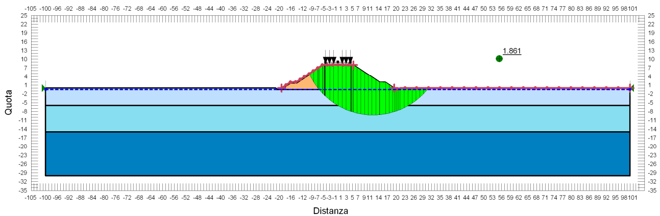
FIGURA 11-5: VERIFICA DI STABILITÀ GLOBALE RILEVATO DI H=8.00 M - CONDIZIONE STATICA NON DRENATA.
