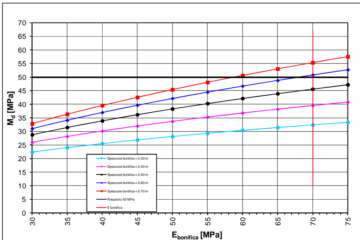
FIGURA 14-2: HRIL \leq 1 M – DETERMINAZIONE SPESSORE DI BONIFICA.
