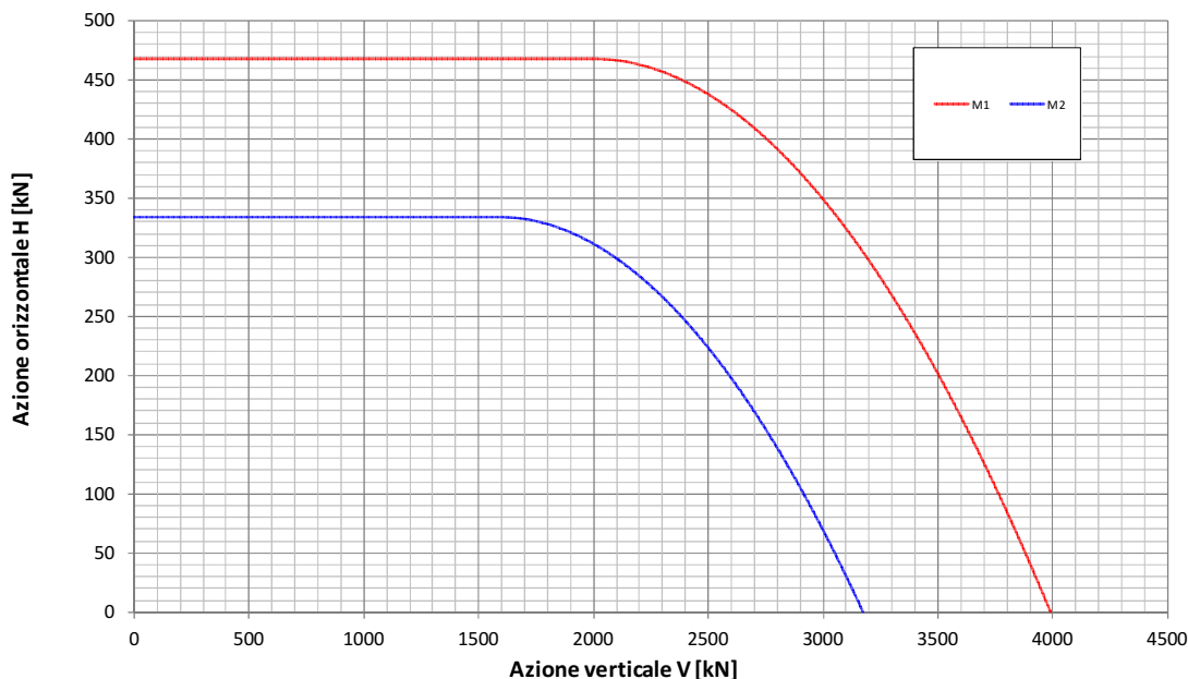
Fondazione B=11.7m - Approfondimento D=5.4m Condizione Statica Non Drenata Dominio di interazione nel piano V-H ( Gourvenec, 2007 )
