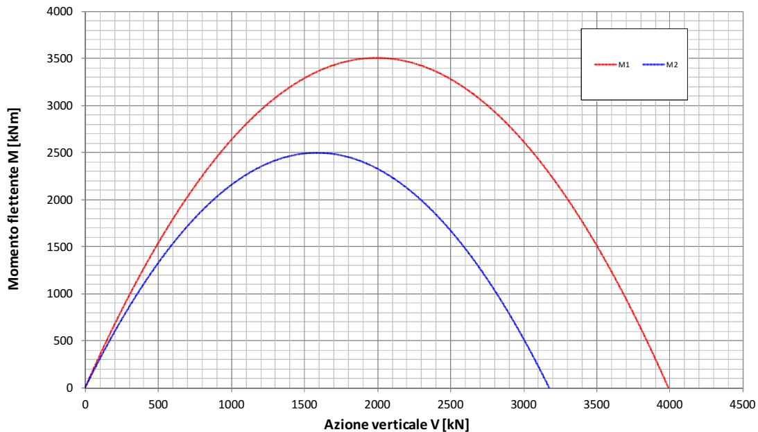
Fondazione B=11.7m - Approfondimento D=5.4m Condizione Sismica Non Drenata Dominio di interazione nel piano V-M ( Gourvenec, 2007 )
