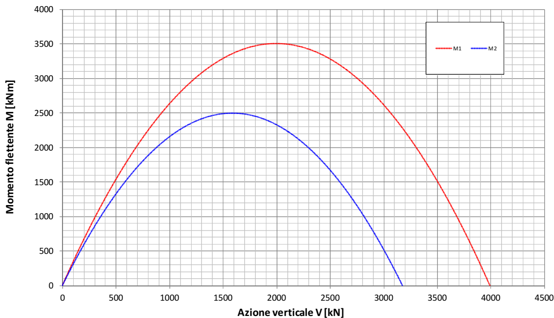
Fondazione B=11.7m - Approfondimento D=5.4m Condizione Statica Non Drenata Dominio di interazione nel piano V-M ( Gourvenec, 2007 )
