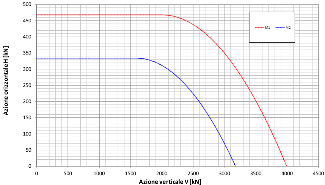
Fondazione B=11.7m - Approfondimento D=5.4m Condizione Sismica Non Drenata Dominio di interazione nel piano V-H ( Gourvenec, 2007 )
