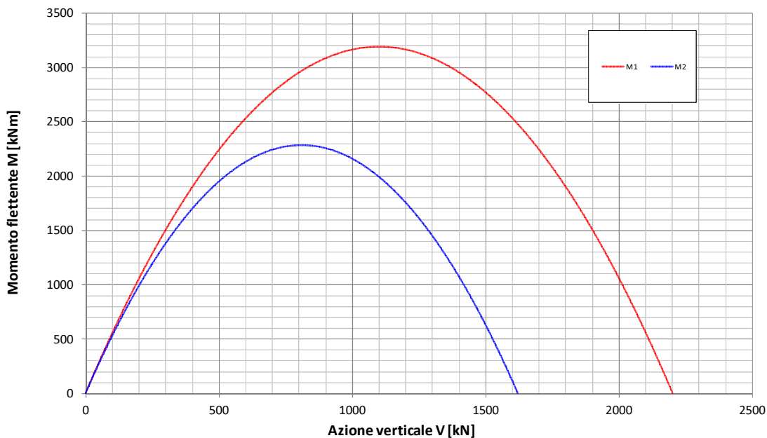
Fondazione B=12.9m - Approfondimento D=0.7m Condizione Statica Non Drenata Dominio di interazione nel piano V-M (Gourvenec, 2007)
