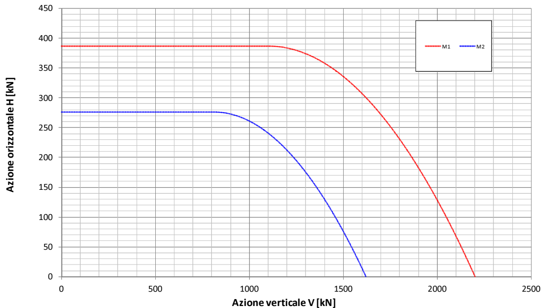
Fondazione B=12.9m - Approfondimento D=0.7m Condizione Sismica Non Drenata Dominio di interazione nel piano V-H ( Gourvenec, 2007 )
