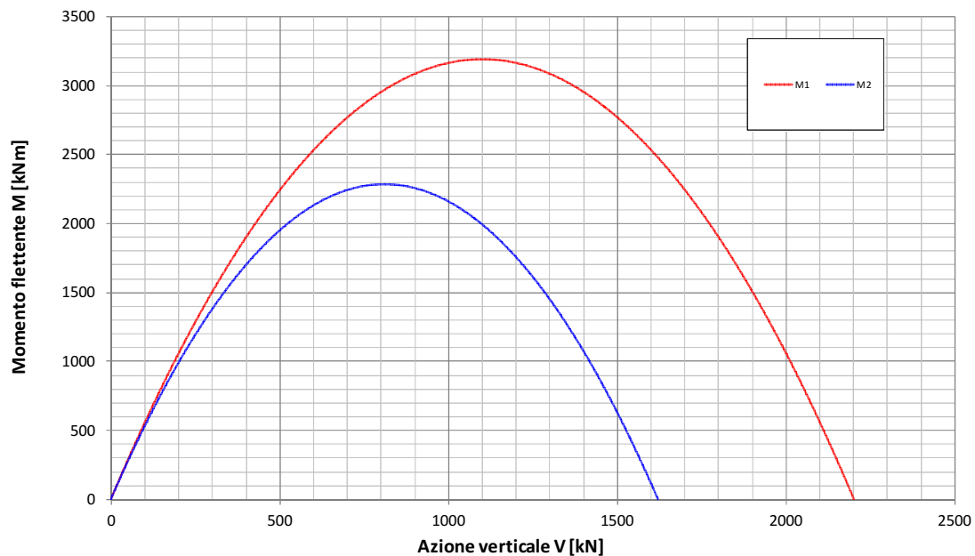
Fondazione B=12.9m - Approfondimento D=0.7m Condizione Sismica Non Drenata Dominio di interazione nel piano V-M ( Gourvenec, 2007 )
