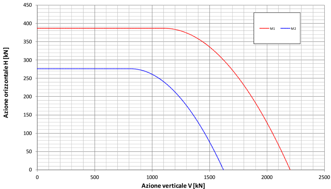
Fondazione B=12.9m - Approfondimento D=0.7m Condizione Statica Non Drenata Dominio di interazione nel piano V-H (Gourvenec, 2007)
