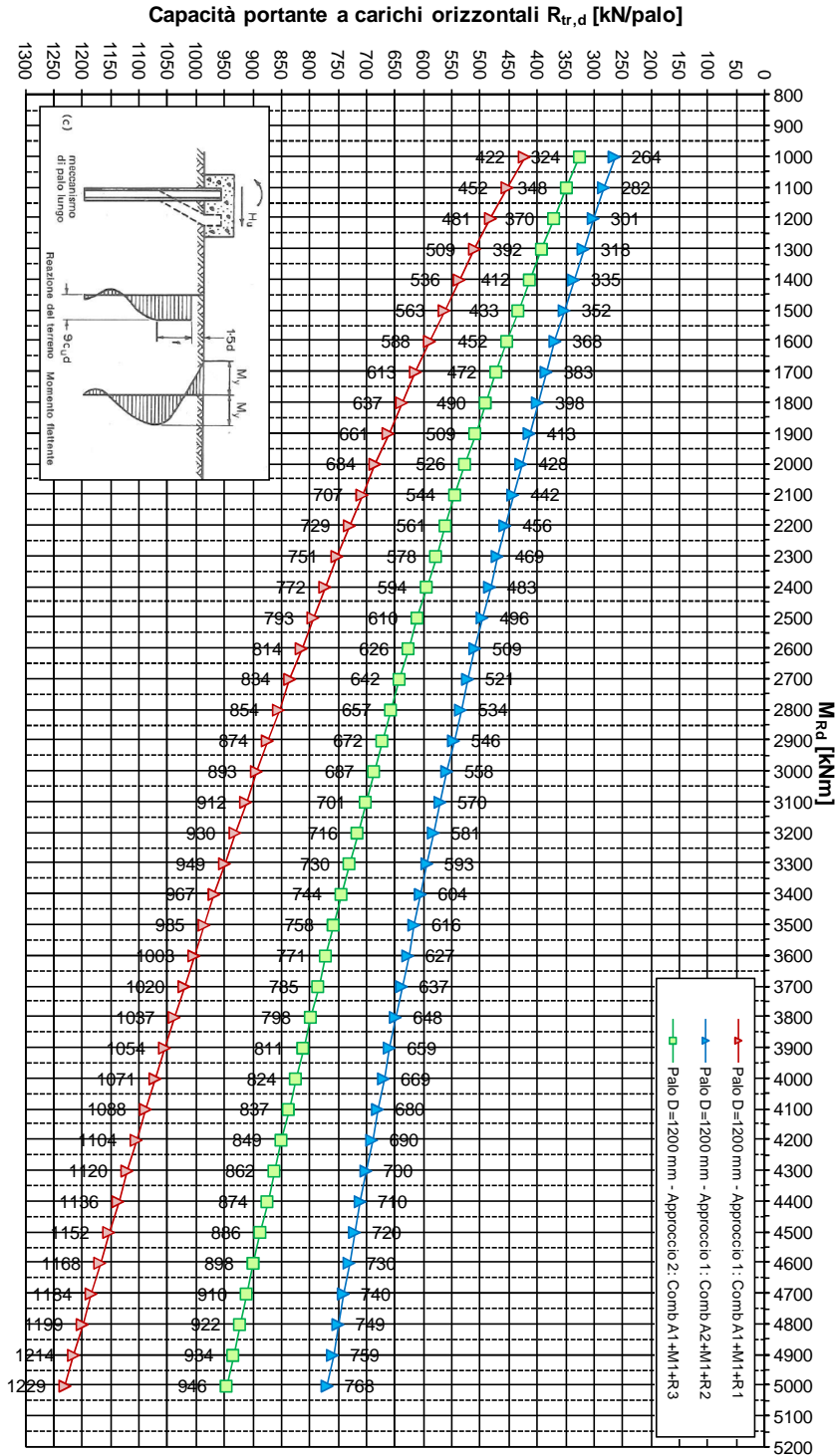
Capacità portante di progetto del singolo palo soggetto a carichi trasversali - R_{tr,d} D = 1200 mm - condizione di incastro in testa Pali di fondazione - Opera VCV14 - Z018
