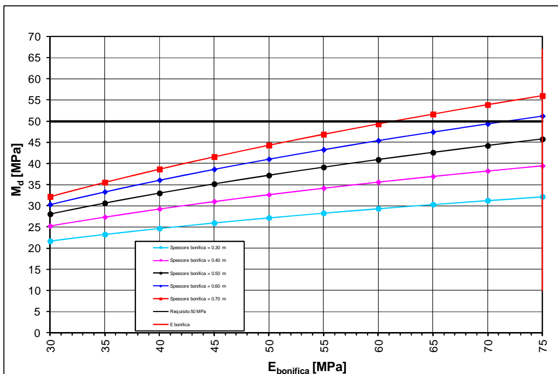
FIGURA 4-2: HRIL ≤ 1M – DETERMINAZIONE SPESSORE DI BONIFICA.
