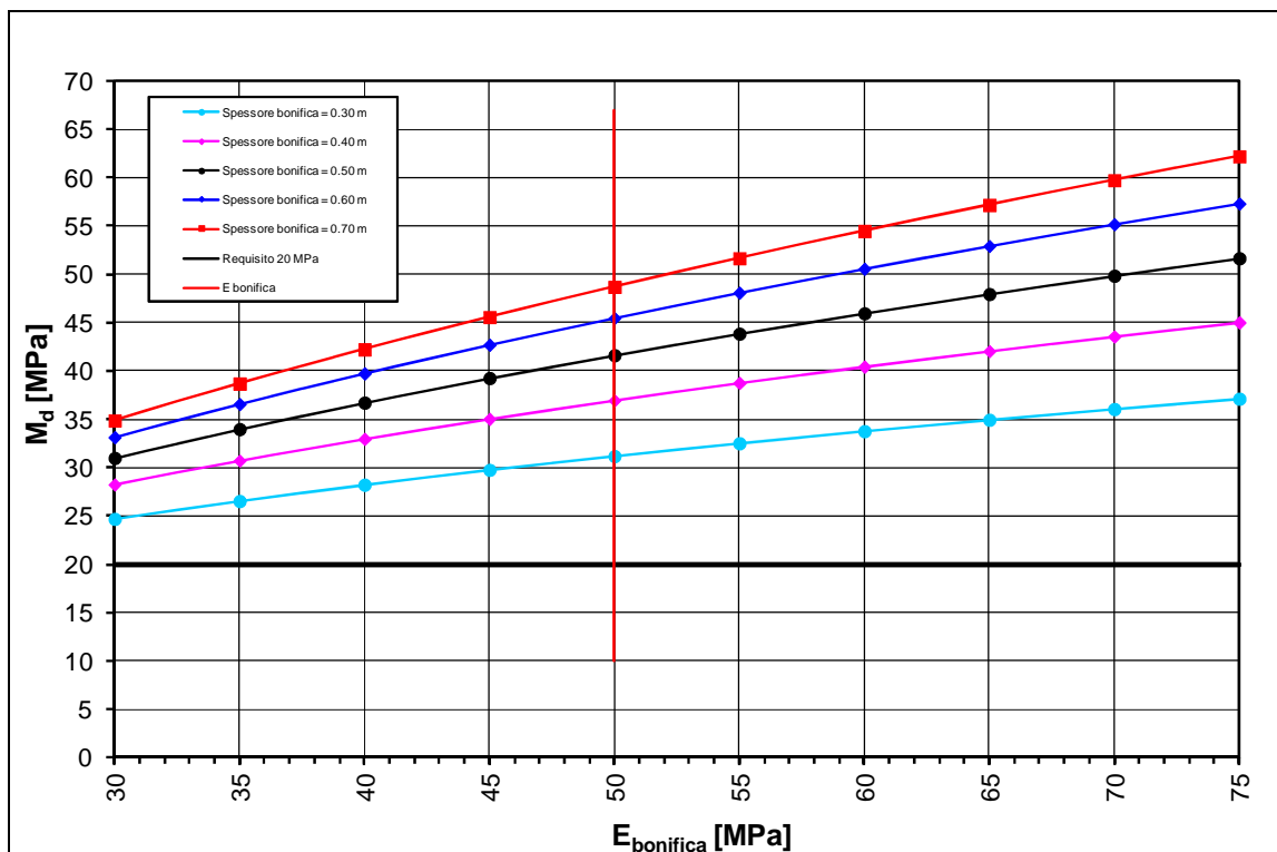
FIGURA 4-3: HRIL > 1M – DETERMINAZIONE SPESSORE DI BONIFICA.
