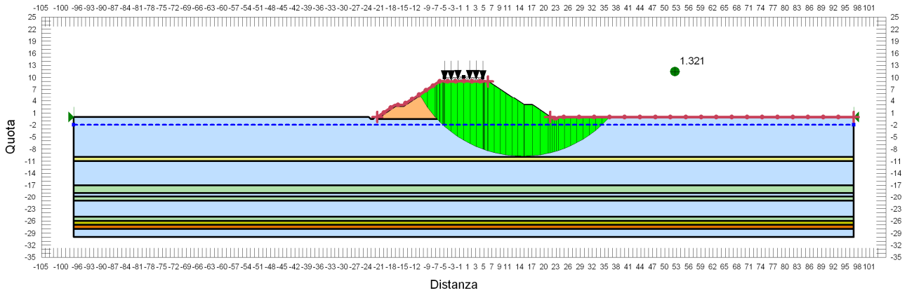
FIGURA 11-7: VERIFICA DI STABILITÀ GLOBALE RILEVATO DI H=9.00 M - CONDIZIONE SISMA+.
