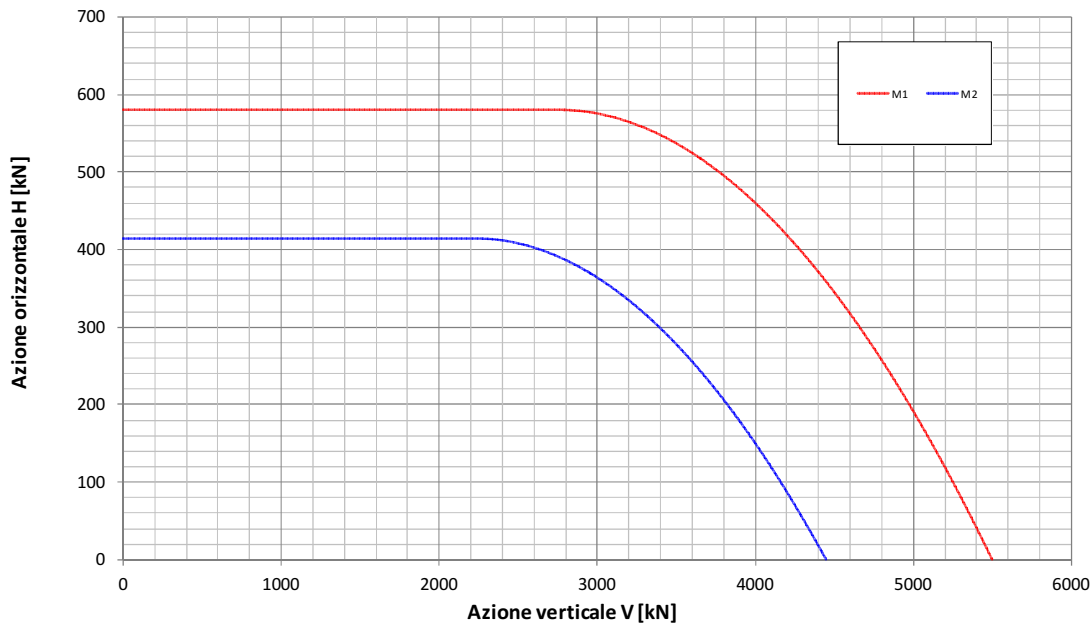
Fondazione B=12.9m - Approfondimento D=7.6m Condizione Statica Non Drenata Dominio di interazione nel piano V-H ( Gourvenec, 2007 )
