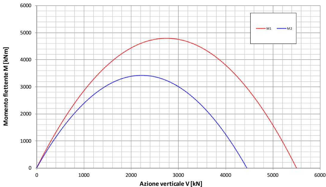
Fondazione B=12.9m - Approfondimento D=7.6m Condizione Statica Non Drenata Dominio di interazione nel piano V-M ( Gourvenec, 2007 )
