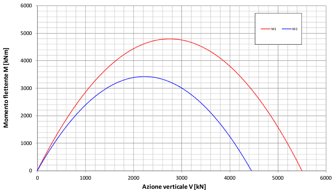
Fondazione B=12.9m - Approfondimento D=7.6m Condizione Sismica Non Drenata Dominio di interazione nel piano V-M ( Gourvenec, 2007 )
