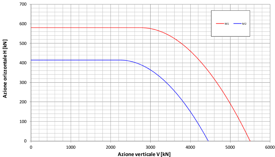
Fondazione B=12.9m - Approfondimento D=7.6m Condizione Sismica Non Drenata Dominio di interazione nel piano V-H ( Gourvenec, 2007 )
