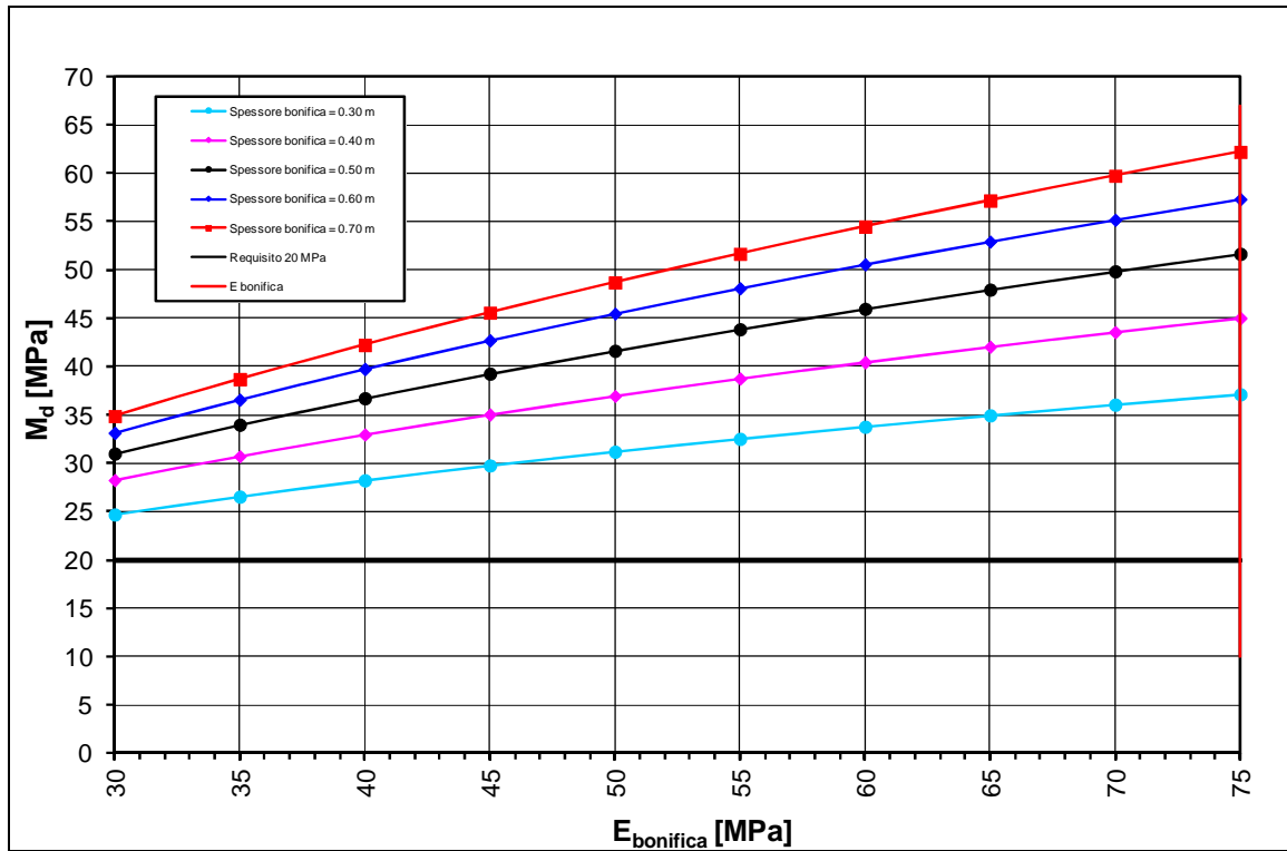
FIGURA 11-3: HRIL > 1M – DETERMINAZIONE SPESSORE DI BONIFICA.
