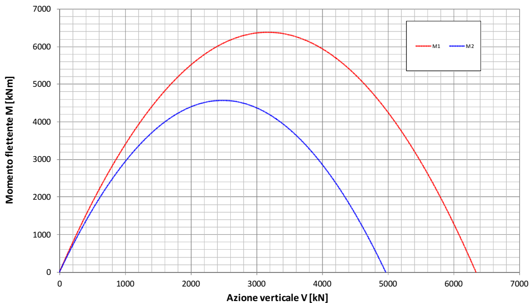
Fondazione B=12.9m - Approfondimento D=6.5m Condizione Statica Non Drenata Dominio di interazione nel piano V-M (Gourvenec, 2007)
