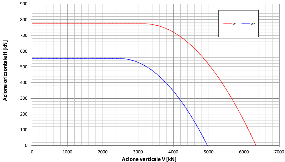
Fondazione B=12.9m - Approfondimento D=6.5m Condizione Sismica Non Drenata Dominio di interazione nel piano V-H (Gourvenec, 2007)
