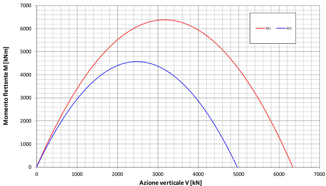
Fondazione B=12.9m - Approfondimento D=6.5m Condizione Sismica Non Drenata Dominio di interazione nel piano V-M (Gourvenec, 2007)
