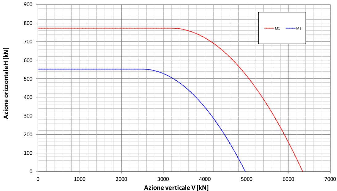
Fondazione B=12.9m - Approfondimento D=6.5m Condizione Statica Non Drenata Dominio di interazione nel piano V-H (Gourvenec, 2007)
