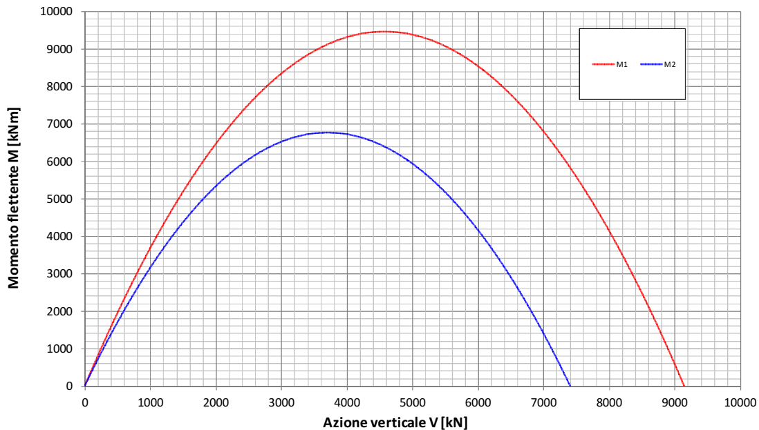
Fondazione B=15.7m - Approfondimento D=10.0m Condizione Statica Non Drenata Dominio di interazione nel piano V-M ( Gourvenec, 2007 )
