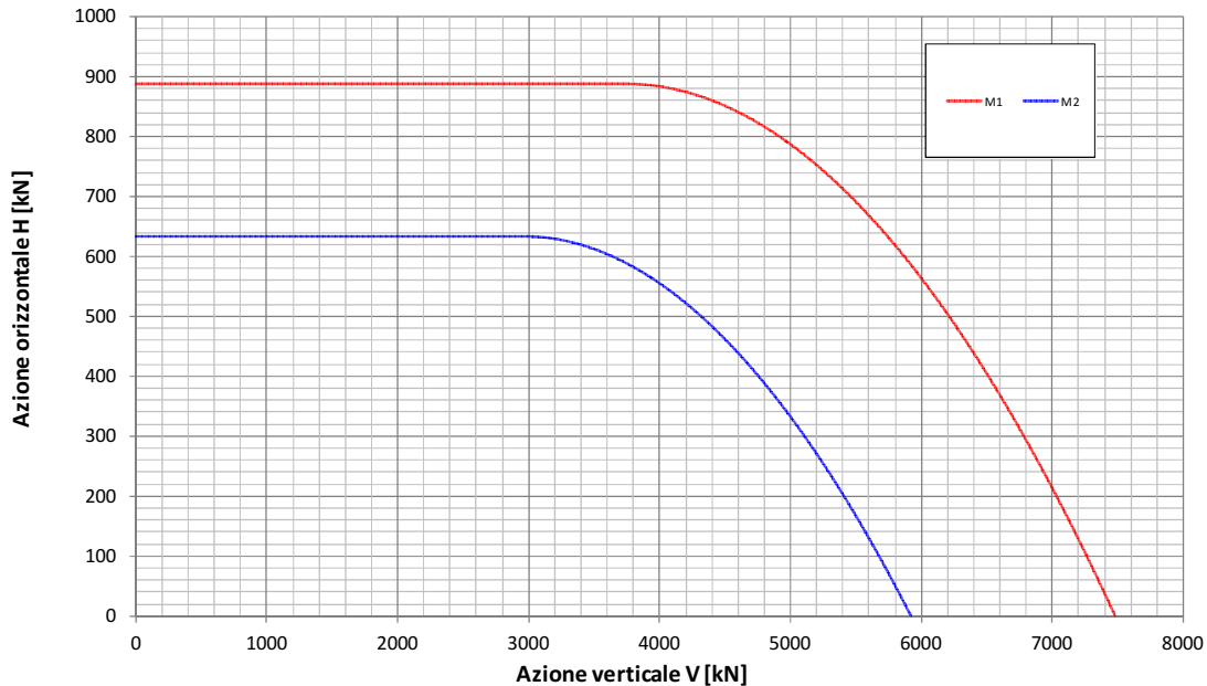
Fondazione B=14.8m - Approfondimento D=7.1m Condizione Statica Non Drenata Dominio di interazione nel piano V-H ( Gourvenec, 2007 )
