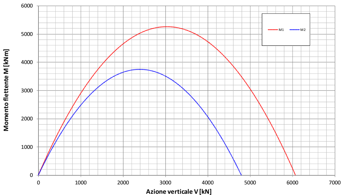
Fondazione B=11.7m - Approfondimento D=7.0m Condizione Statica Non Drenata Dominio di interazione nel piano V-M (Gourvenec, 2007)
