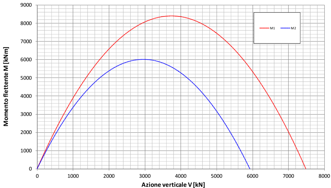
Fondazione B=14.8m - Approfondimento D=7.1m Condizione Sismica Non Drenata Dominio di interazione nel piano V-M ( Gourvenec, 2007 )
