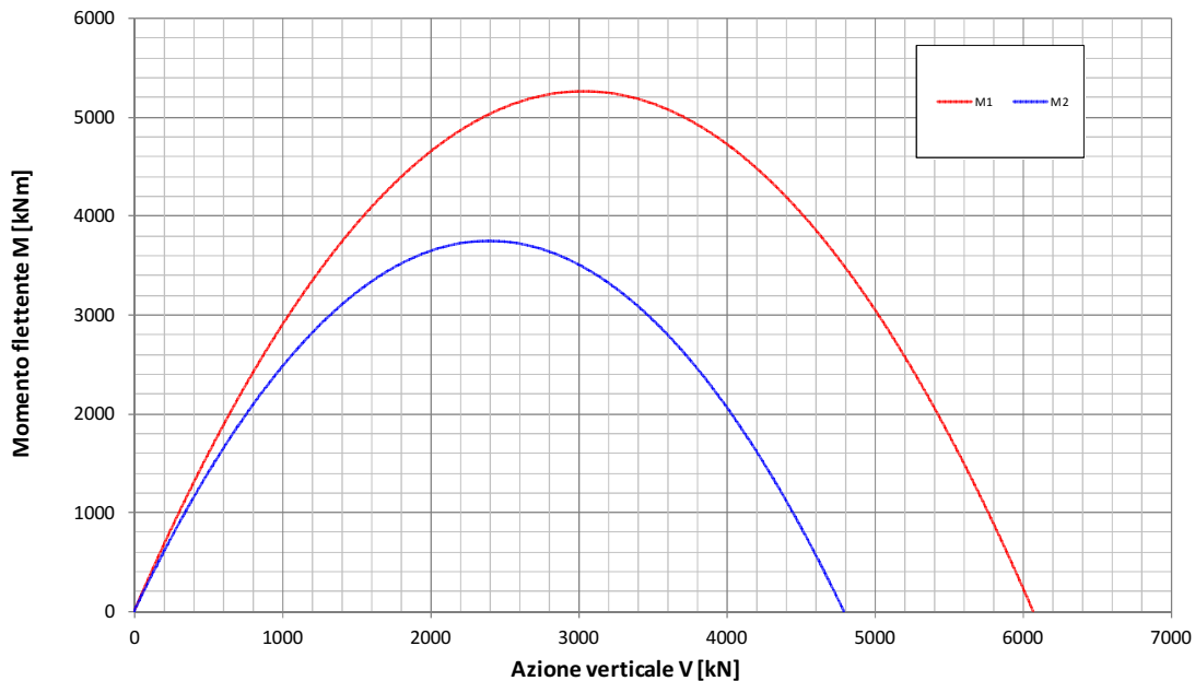
Fondazione B=11.7m - Approfondimento D=7.0m Condizione Sismica Non Drenata Dominio di interazione nel piano V-M (Gourvenec, 2007)
