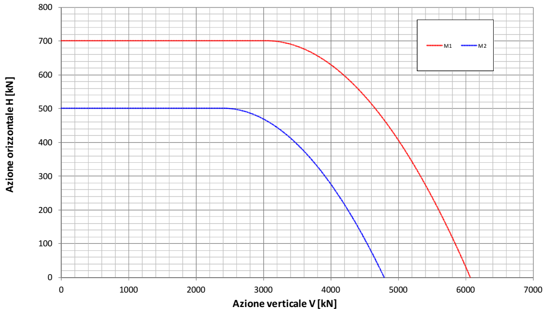
Fondazione B=11.7m - Approfondimento D=7.0m Condizione Sismica Non Drenata Dominio di interazione nel piano V-H (Gourvenec, 2007)
