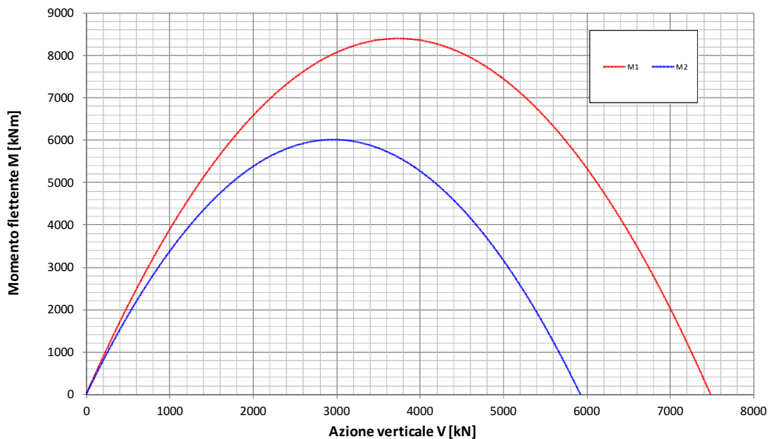
Fondazione B=14.8m - Approfondimento D=7.1m Condizione Statica Non Drenata Dominio di interazione nel piano V-M ( Gourvenec, 2007 )
