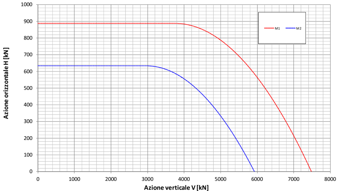
Fondazione B=14.8m - Approfondimento D=7.1m Condizione Sismica Non Drenata Dominio di interazione nel piano V-H ( Gourvenec, 2007 )
