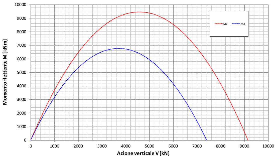
Fondazione B=15.7m - Approfondimento D=10.0m Condizione Sismica Non Drenata Dominio di interazione nel piano V-M ( Gourvenec, 2007 )
