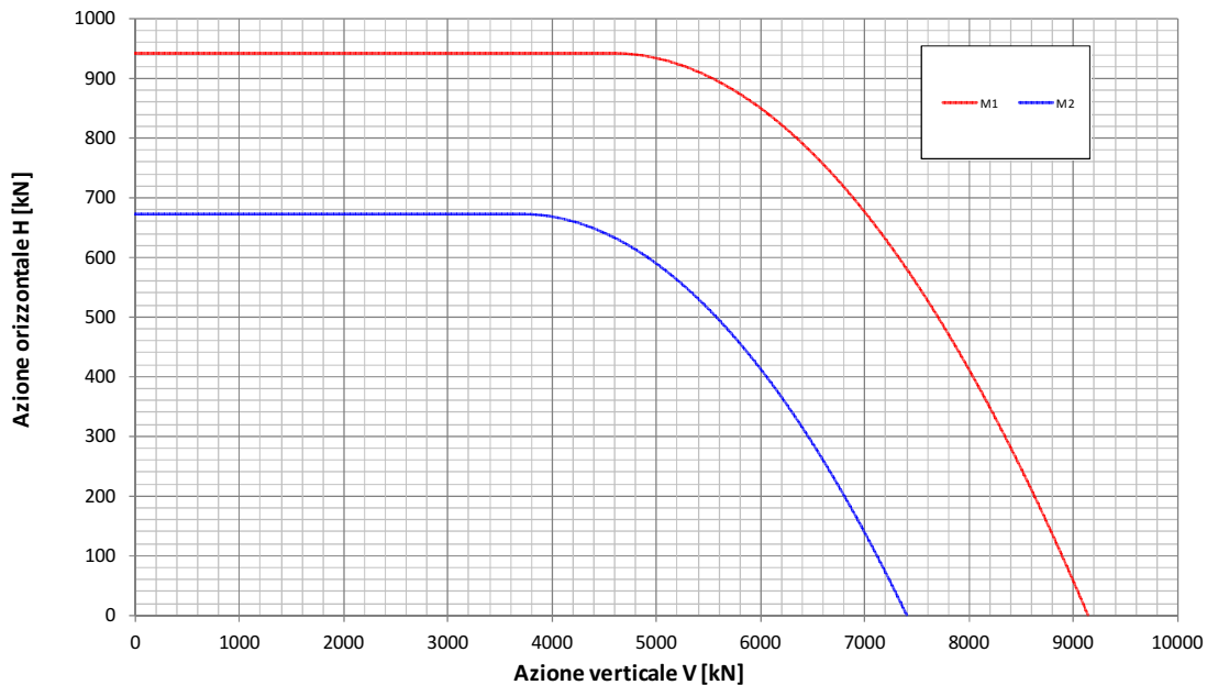
Fondazione B=15.7m - Approfondimento D=10.0m Condizione Sismica Non Drenata Dominio di interazione nel piano V-H ( Gourvenec, 2007 )
