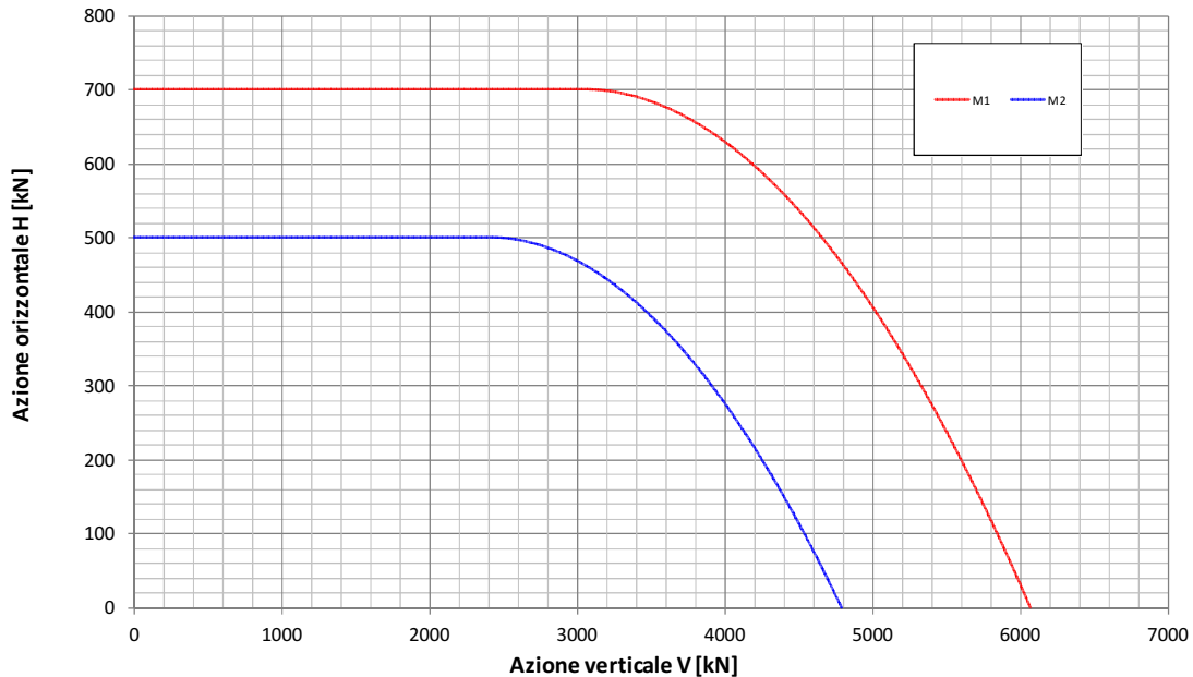
Fondazione B=11.7m - Approfondimento D=7.0m Condizione Statica Non Drenata Dominio di interazione nel piano V-H (Gourvenec, 2007)
