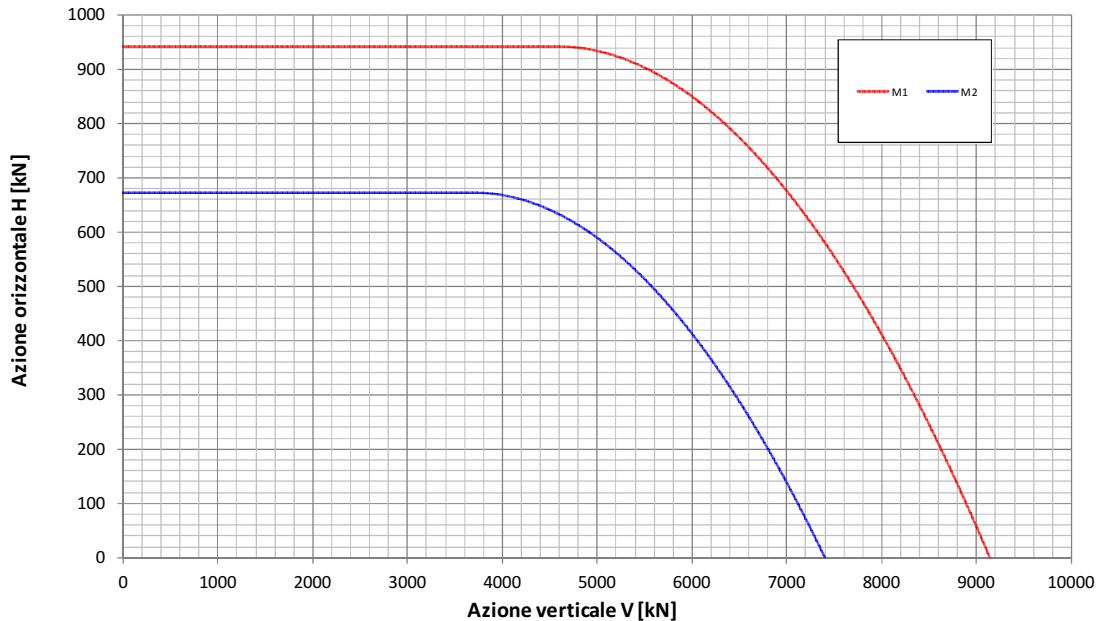
Fondazione B=15.7m - Approfondimento D=10.0m Condizione Statica Non Drenata Dominio di interazione nel piano V-H ( Gourvenec, 2007 )
