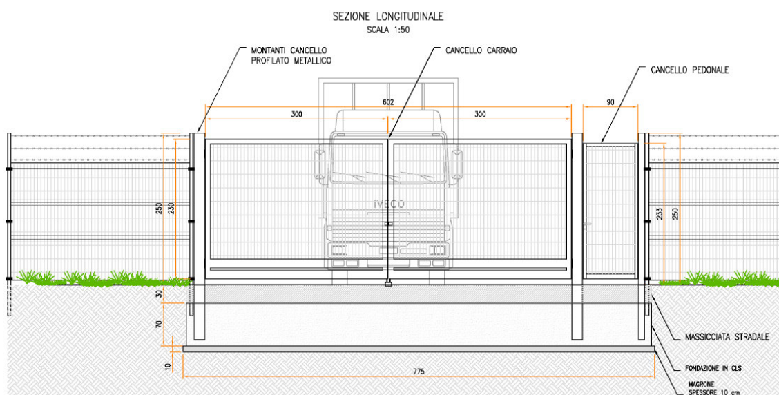
Figura 2.11: Particolare accesso
