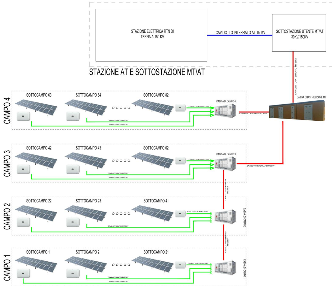
Figura 59 - Schema delle connessioni elettriche
