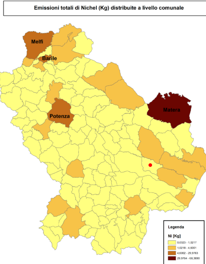
Figura 96 - Carta della emissioni totali di Nichel NI (Kg) distribuite a livello comunale. (Fonte: Progetto di zonizzazione e classificazione - Regione Basilicata - (Decreto Legislativo 13 Agosto 2010, N. 155)
