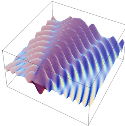
Figura 119 - Diffrazione di un'onda di superficie (fonte: www.Wikipedia.org )
