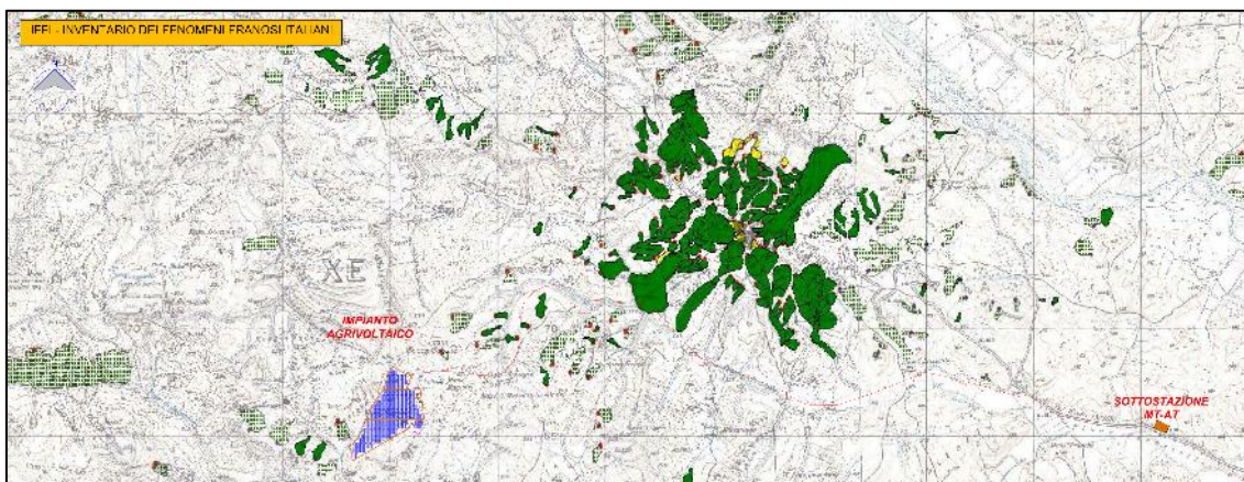
Figura 34 - Inventario dei Fenomeni Franosi Italiani
