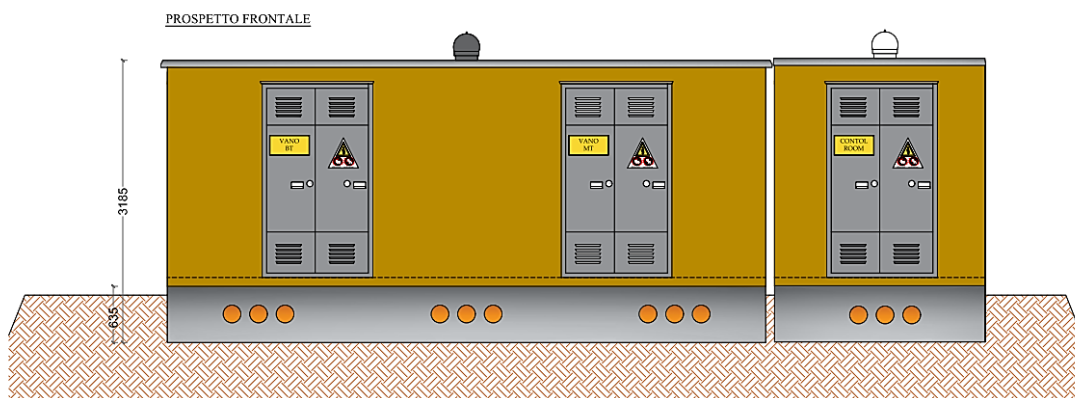
Figura 53 - Cabine
