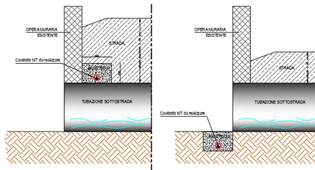
CASO A PACCHETTO STRADALE > 40cm
