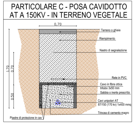
Figura 60 - Sezioni di scavo dei cavidotti
