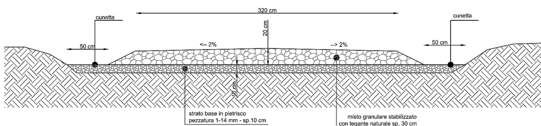
Figura 58 - Sezione tipo strada di collegamento impianto/viabilità pubblica (Fonte: ns elaborazione)
