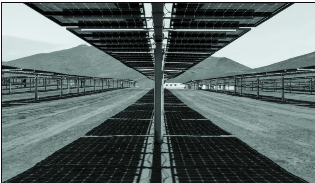
Figura 52 - Esempi di tracker per impianti fotovoltaici
