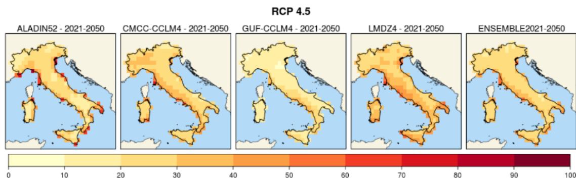
Figura 76 - Aumento dei giorni con onde di calore (giorni), scenario RCP4.5(fonte: ISPRA)
