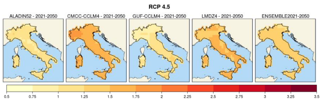
Figura 68 - Temperatura media (°C), scenario RCP4.5 (fonte: ISPRA)
