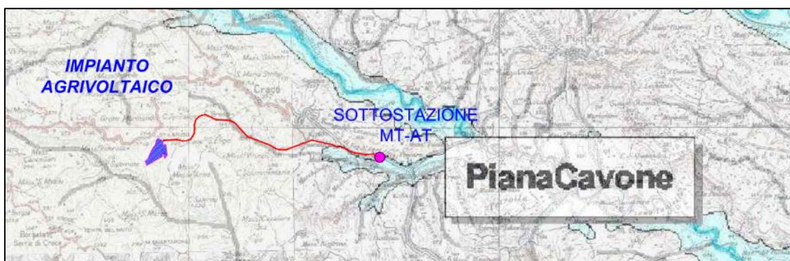
Figura 99 - Corpi idrici sotterranei. Le aree di colore azzurro rappresentano i "Sistemi acquiferi tipo D (Sistemi clastici di Piana Alluvionale)
