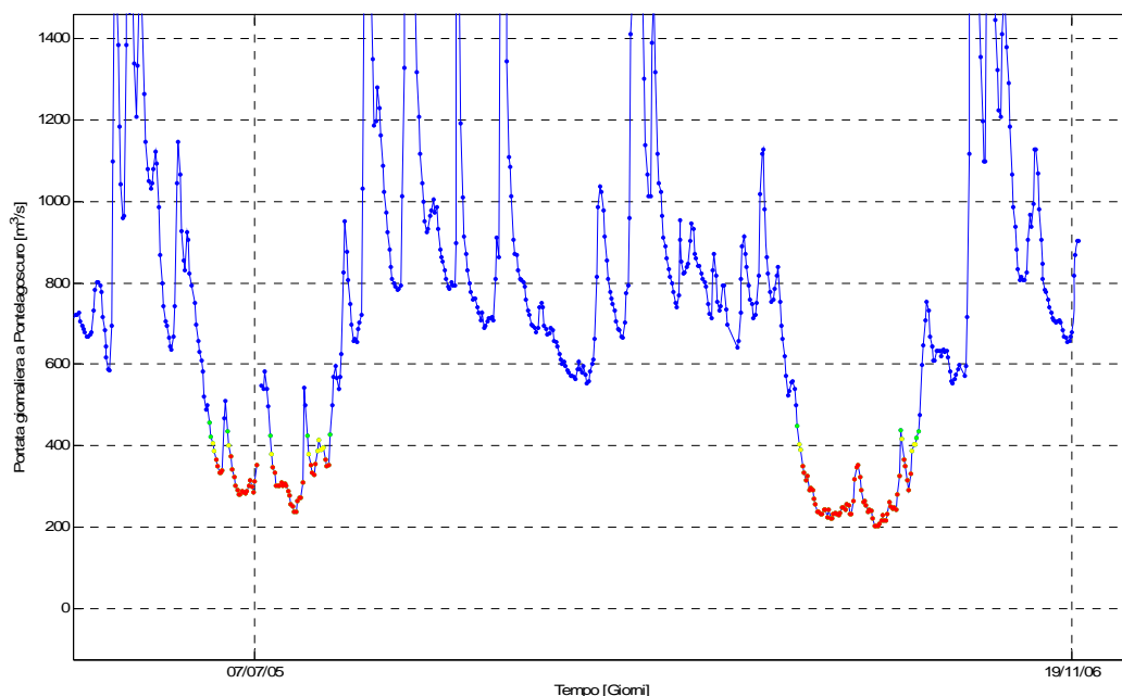
Figura 2 - Andamento della portata registrata nel Po a Pontelagoscuro tra le magre estive del 2005 e del 2006, con indicati i dati per cui le tre portate 460 m 3 /s (in verde in Figura), 420 m 3 /s (in giallo in Figura) e 380 m 3 /s (in rosso in Figura) non vengono superate.
