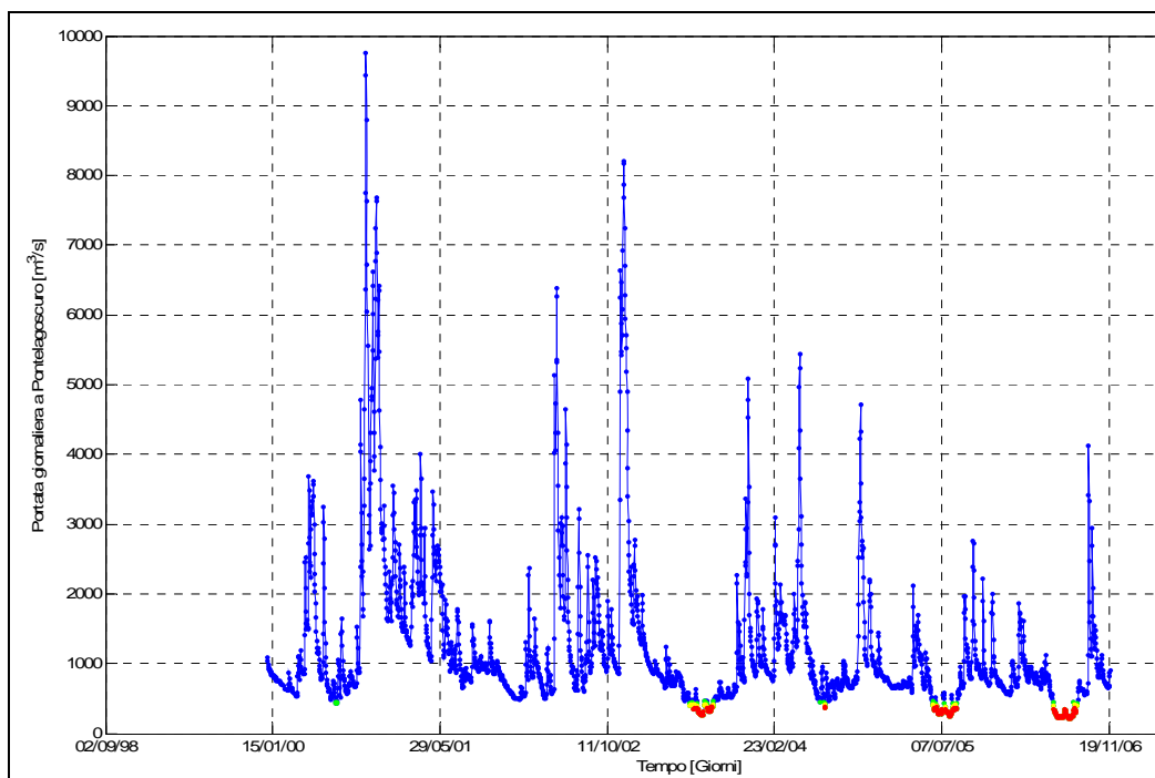
Figura 1 - Andamento della portata registrata nel Po a Pontelagoscuro negli anni 2000 e 2006, con indicati i dati per cui le tre portate 460 m 3 /s (in verde in Figura), 420 m 3 /s (in giallo in Figura) e 380 m 3 /s (in rosso in Figura) non vengono superate.
