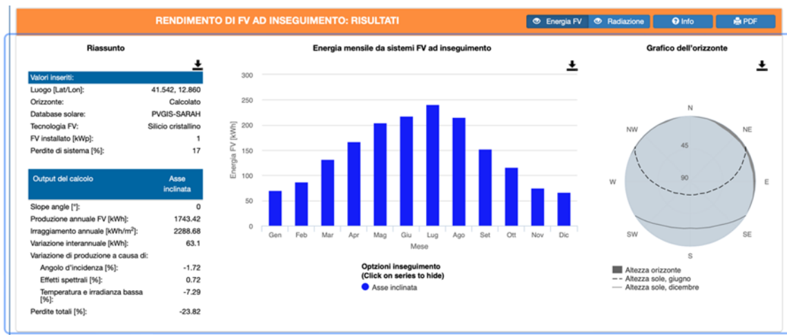
Grafico 7 - Producibilità annua per 1 kWp installato
