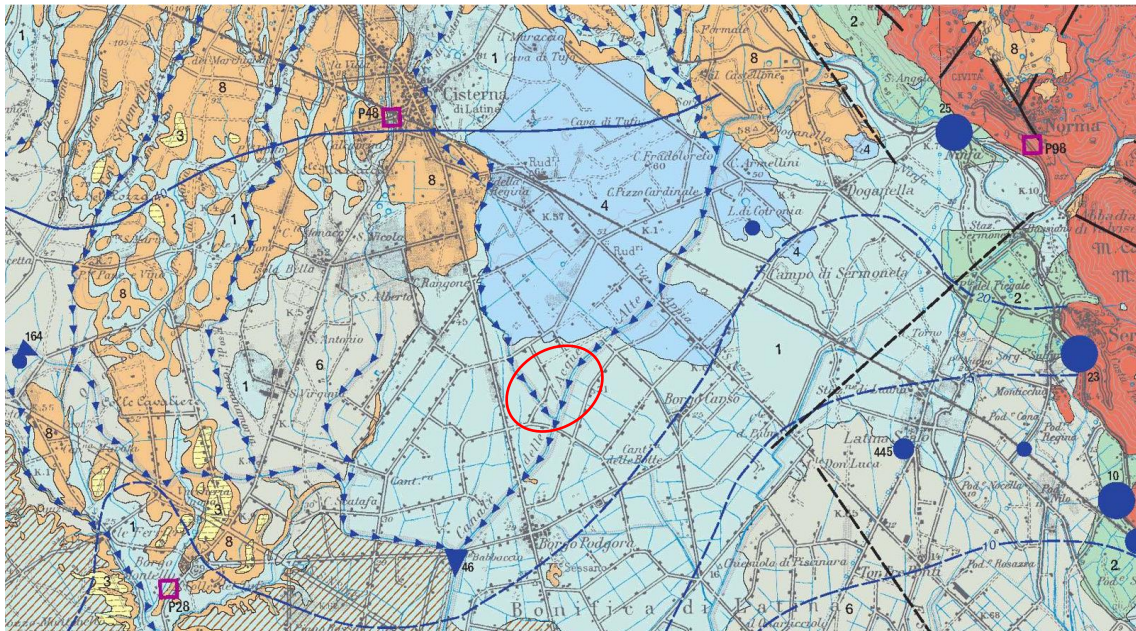
Figura 11 - Stralcio della Carta Idrogeologica del territorio della Regione Lazio riportante l'area entro la quale ricade l'impianto agrovoltatico in progetto e relativa Legenda d'interesse (segue Legenda)
