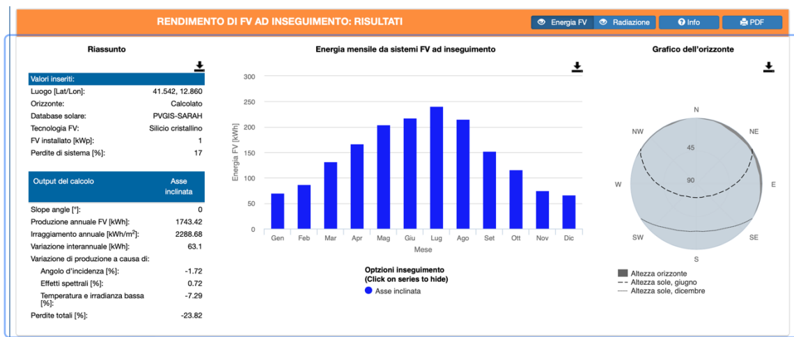
Gráfico 6 - Producibilità annua per 1 kWp installato
