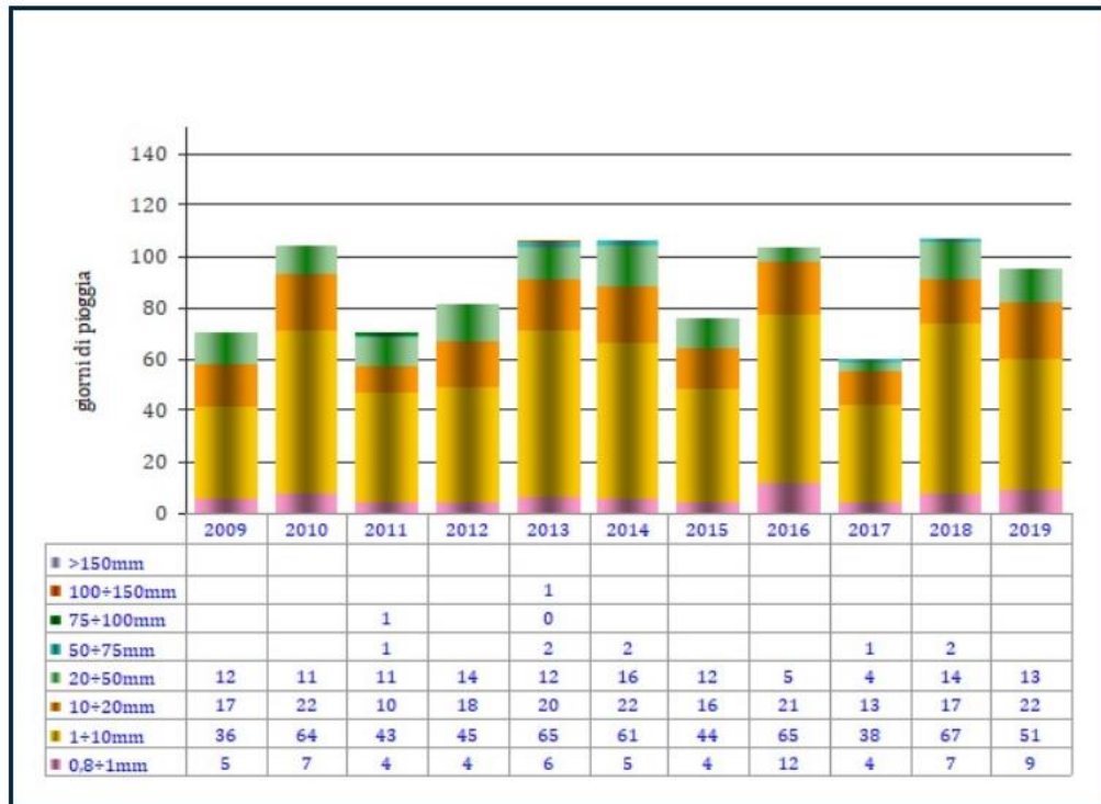
Grafico 4 - Rappresentazione grafica del numero di giorni di pioggia entro il range 2009-2019
