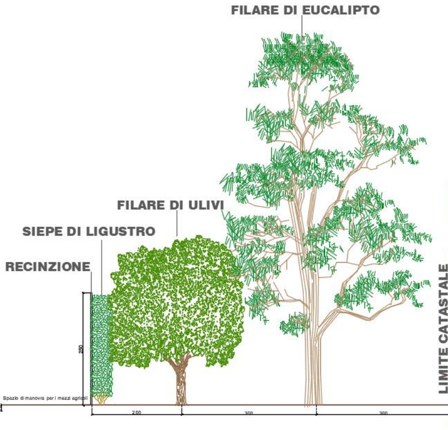
Figura 33 - Schemi di posa delle piantumazioni delle opere di mitigazione
