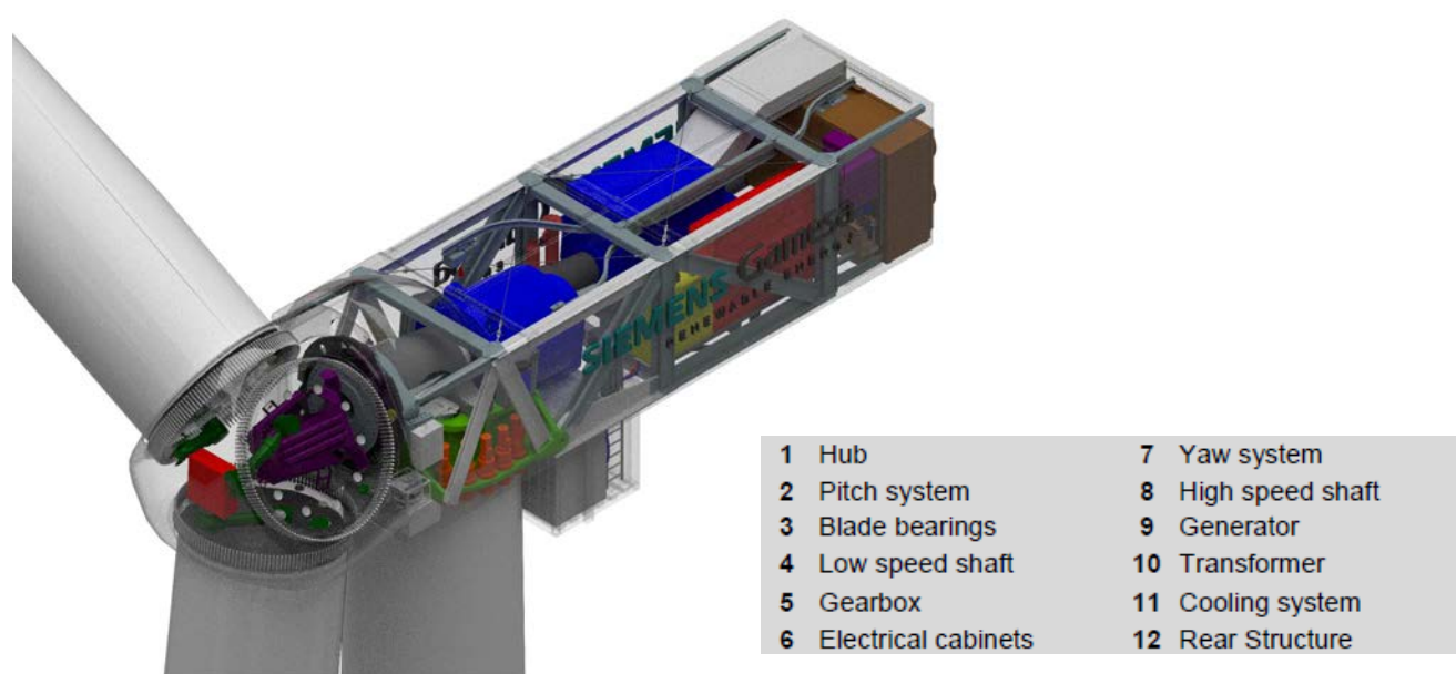
Dettaglio rotore
